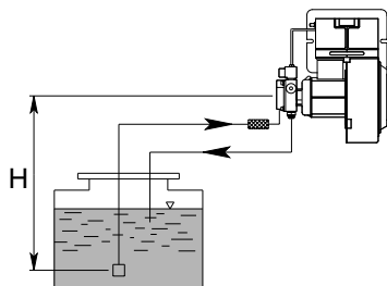
Raccordement bitube en aspiration
