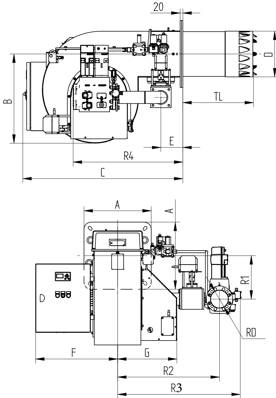
Fig. 7 Dimensioni ingombro
