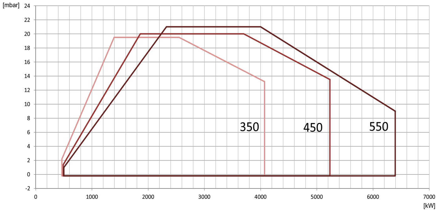
Fig. 6 X = Potenza termica [kW] Y = Pressione in camera di combustione [mbar]
