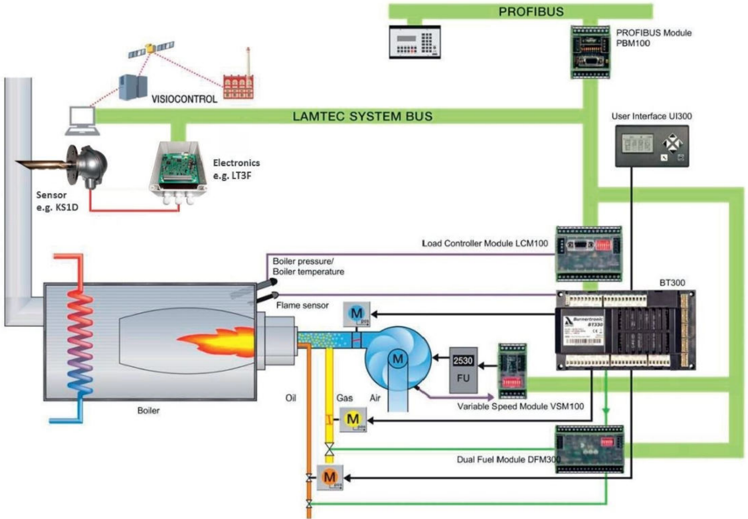
Fig. 5 Camma elettronica Lamtec BT3
