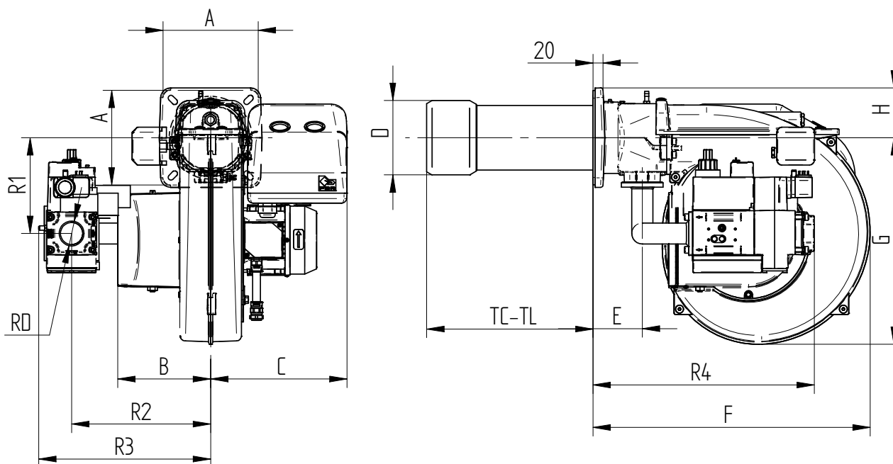
Fig. 3 Dimensioni ingombro GAS XP60CE EVO
