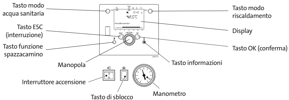
Fig. 12: Regolatore di sistema integrato ISR-Plus LMS, pannello di comando EcoTherm Plus BBS 15 - 28 serie E
