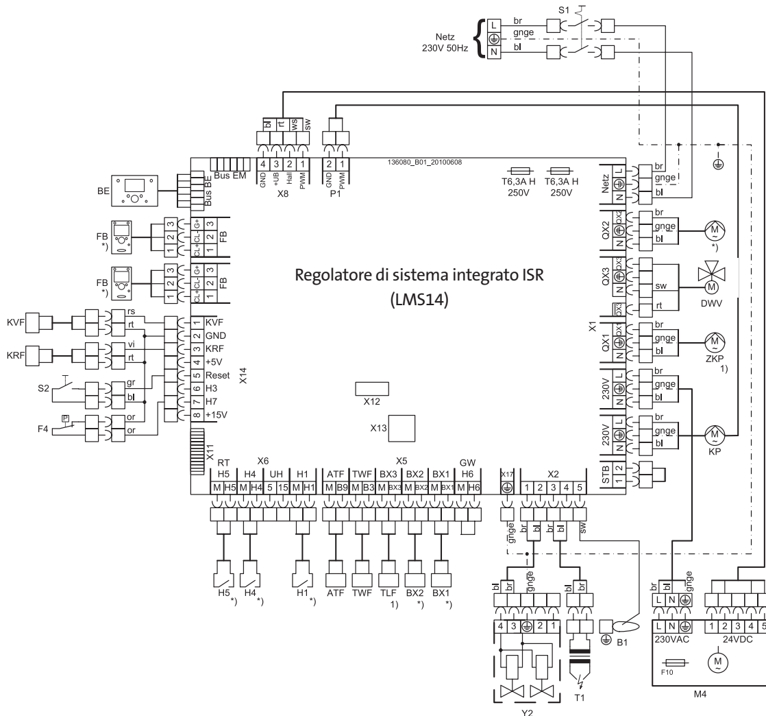
Schema degli allacciamenti EcoCondens BBS serie E
