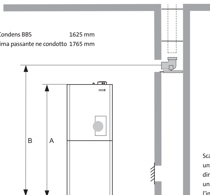
Fig. 15: Dimensioni d'installazione minime
