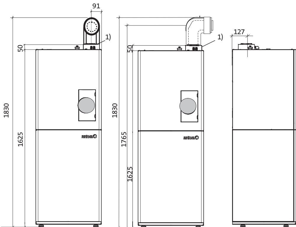
Fig. 14: Dimensioni attacco scarico fumi EcoCondens BBS
