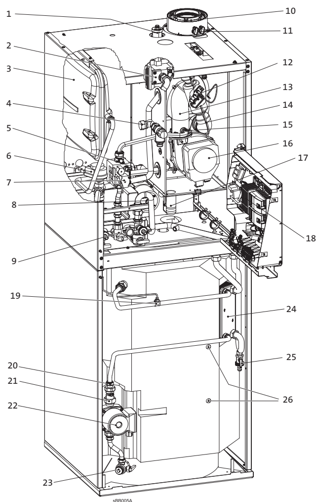
Fig. 7: Vista della caldaia (rappresentata senza pannello frontale e copertura della regolazione)
