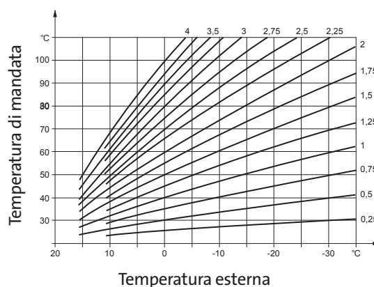
Fig. 13: Diagramma curve caratteristiche di riscaldamento
