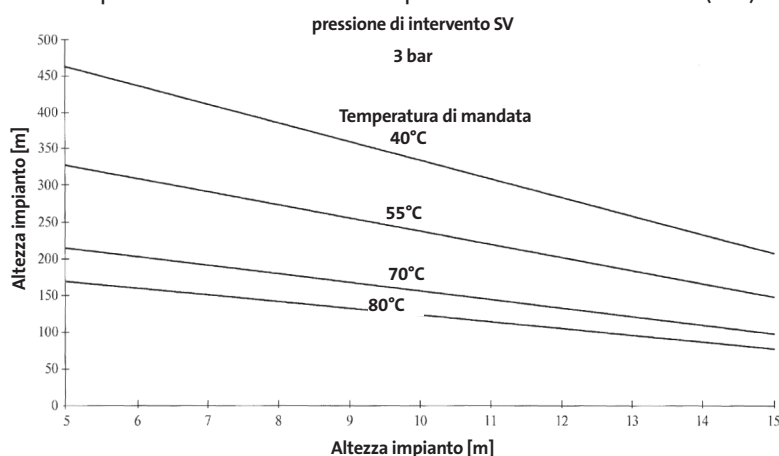
Fig. 19: max. contenuto dell'impianto utilizzando il vaso d'espansione a membrana MAG (12 l)
