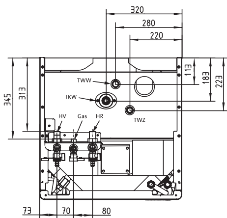
Fig. 17: Vista dall'alto sul bollitore
