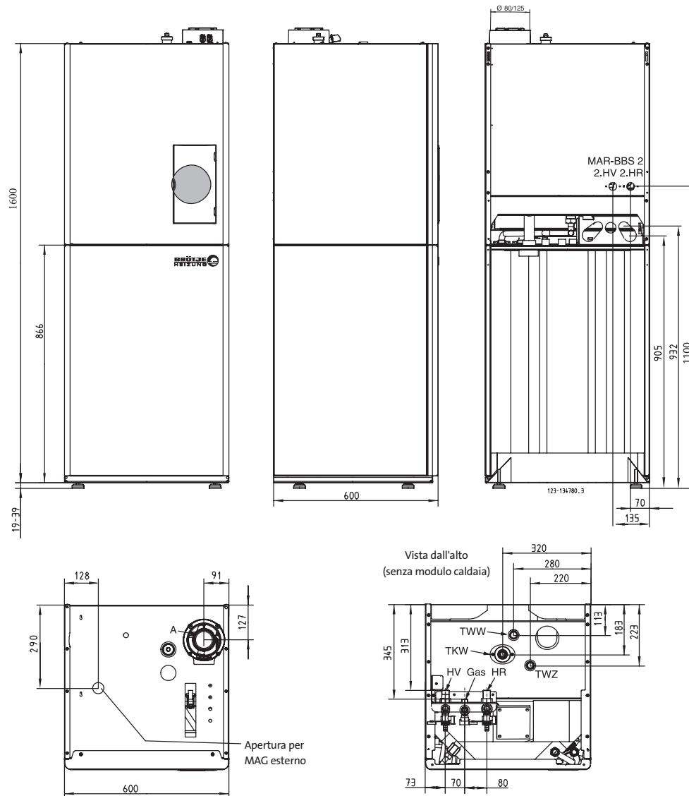
Fig. 10: Dimensioni EcoCondens BBS 15 E, 20 E e 28 E
