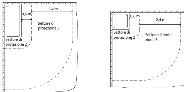
Fig. 18: Distanze minime dei settori di protezione in ambienti umidi 2 e 3
