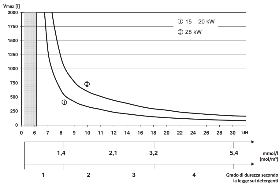
Fig. 20: Diagramma durezza dell'acqua EcoCondens BBS 15–28
