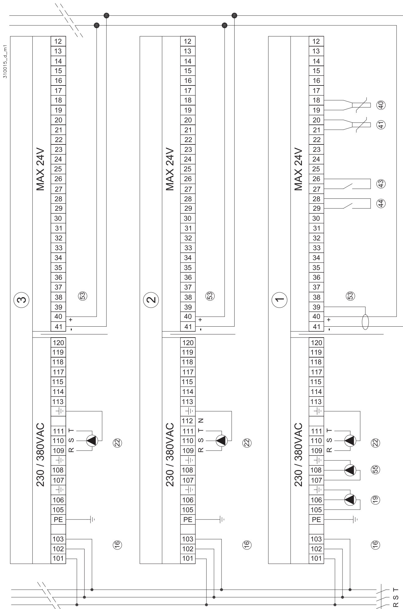
Figura 5-22 - Esempio di collegamento elettrico della cascata con un MASTER
