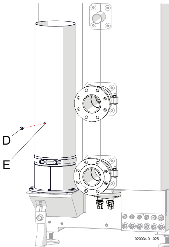
Figura 6-4 - Foro per analisi combustione
