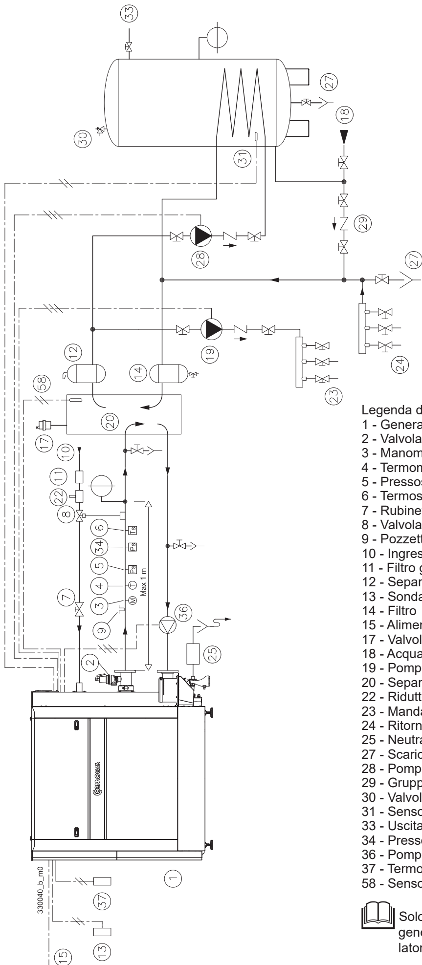
Figura 5-10 - Esempio di collegamento con separatore idraulico e bollitore
