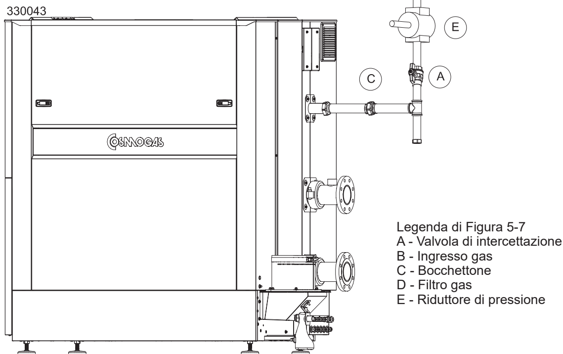
Figura 5-7 - Collegamento gas
