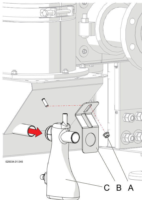
Figura 8-21 - Pulizia dello scarico della condensa
