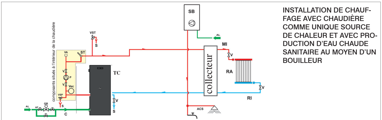
INSTALLATION DE CHAUFFAGE AVEC CHAUDIÈRE COMME UNIQUE SOURCE DE CHALEUR ET AVEC PRODUCTION D'EAU CHAUDE SANITAIRE AU MOYEN D'UN BOUILLEUR
