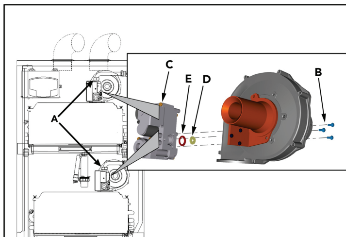
fig. 39 - Trasformazione gas
