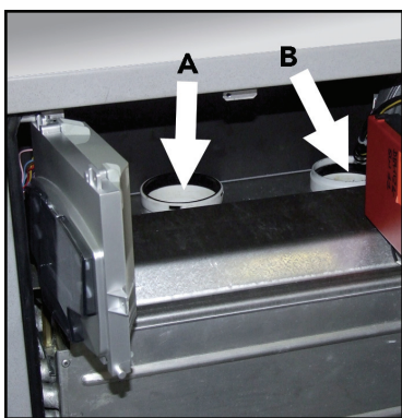
fig. 30 - Riempimento sifone
