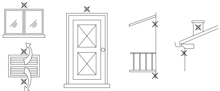
fig. 25 - Posizionamento sconsigliato sonda esterna
