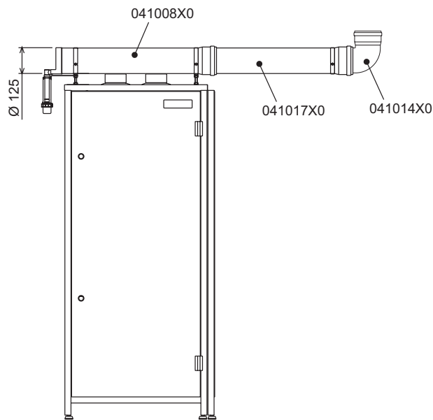
fig. 31 - Installazione di un modulo
