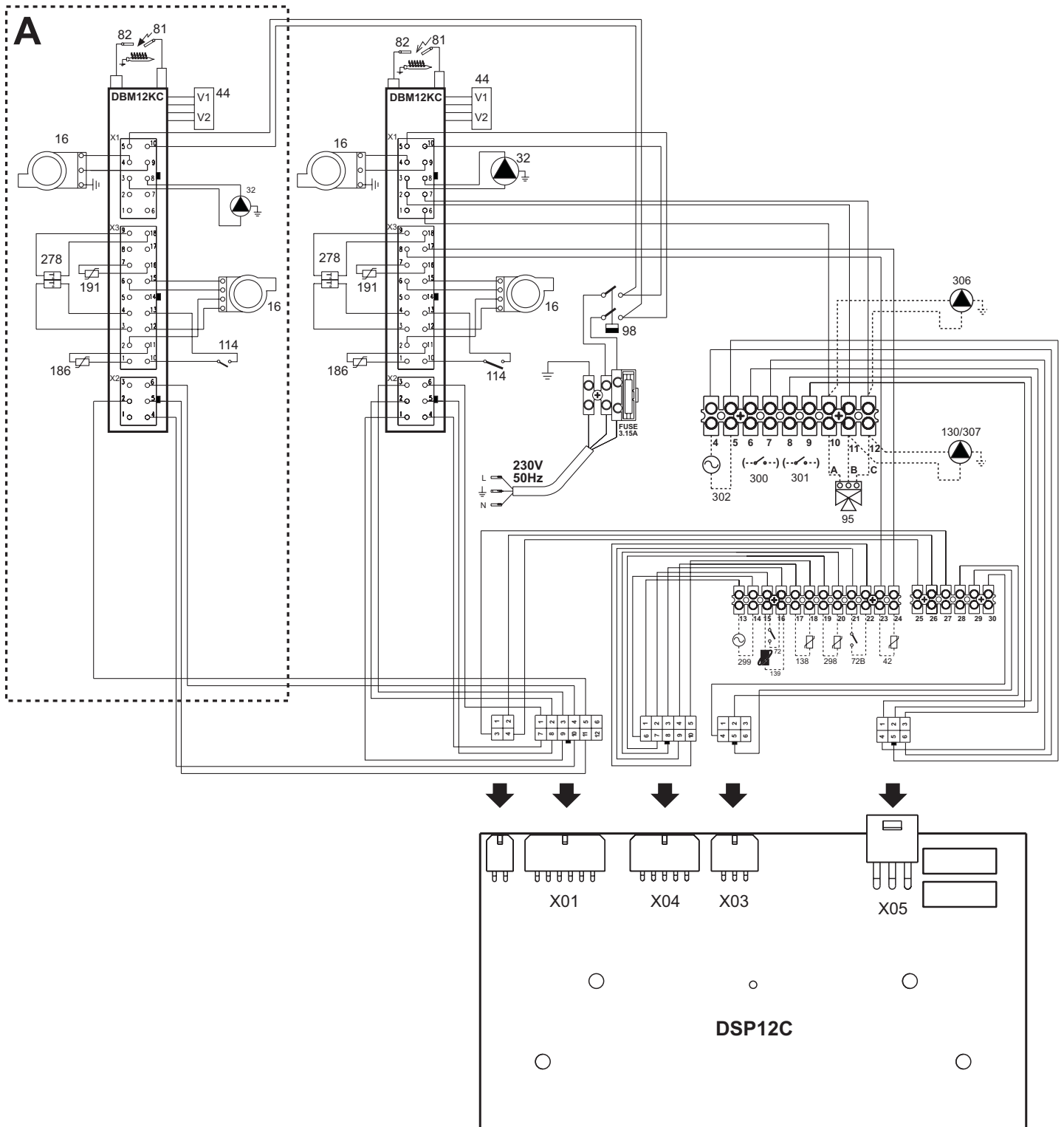
fig. 47 - Schema elettrico
