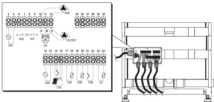
fig. 26 - Morsetteria elettrica
