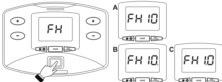
fig. 4 - Accensione caldaia
