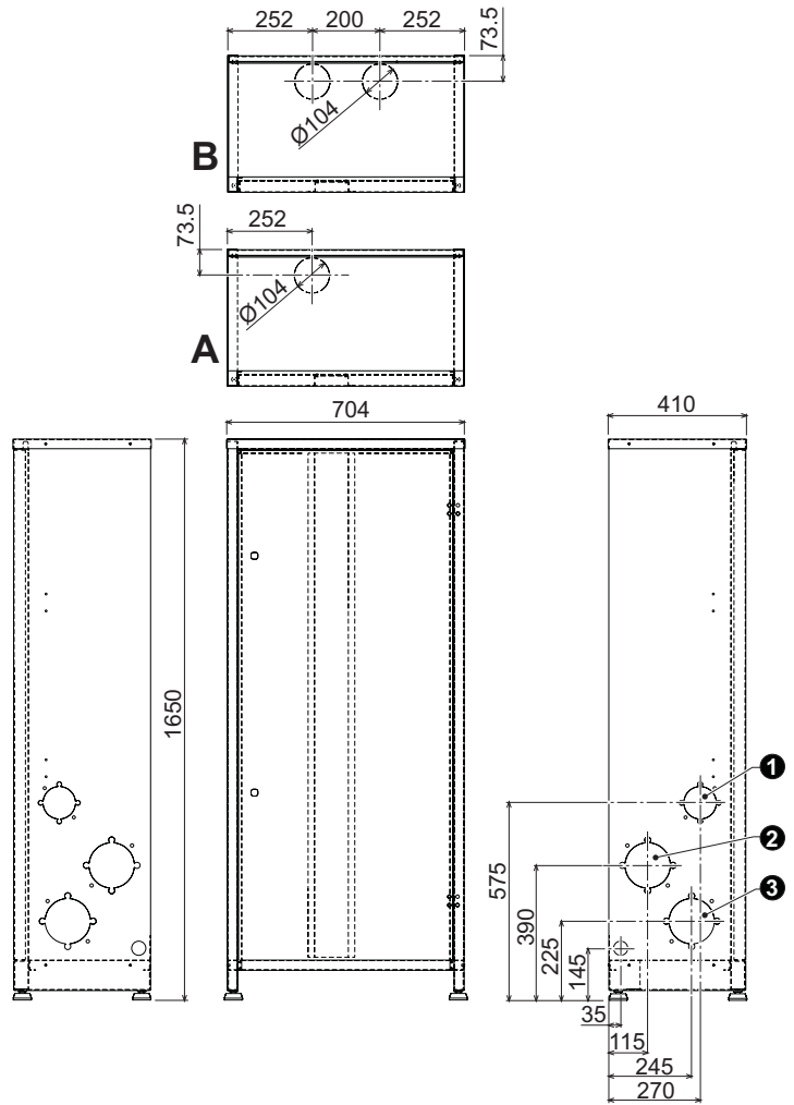
fig. 41 - Dimensioni e attacchi
