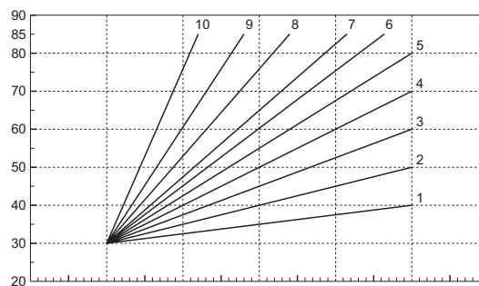
fig. 12 - Curve di compensazione
