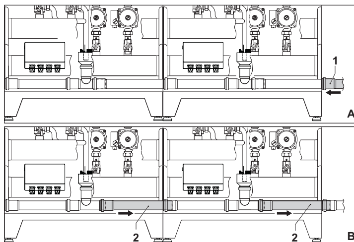
fig. 38 - Collegamento scarico condensa con più generatori
