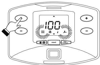
fig. 40 - Modalità TEST (potenza riscaldamento = 100%)
