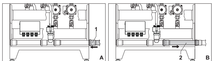
fig. 37 - Collegamento scarico condensa con un generatore
