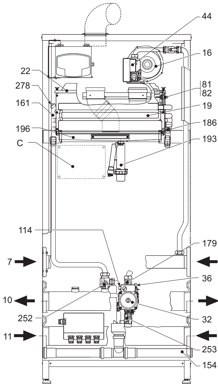
fig. 42 - Vista generale AURA COMBI 51/i
