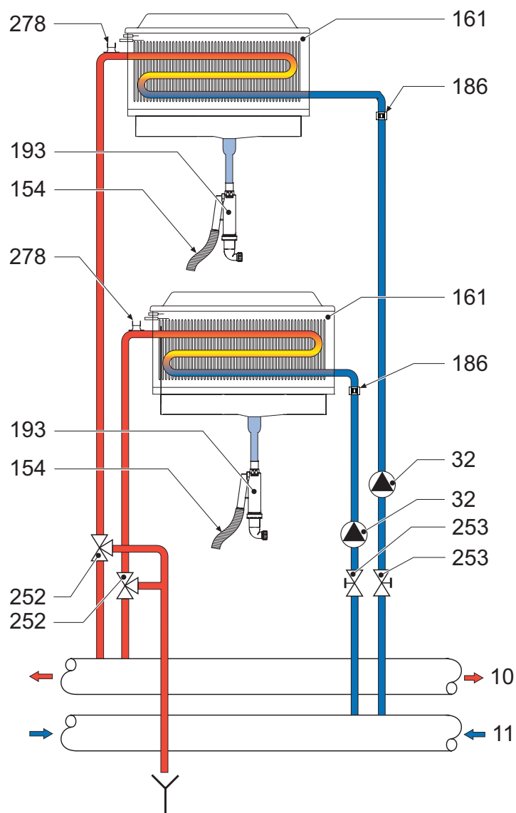
fig. 45 - Circuito idraulico AURA COMBI 71/i-101/i
