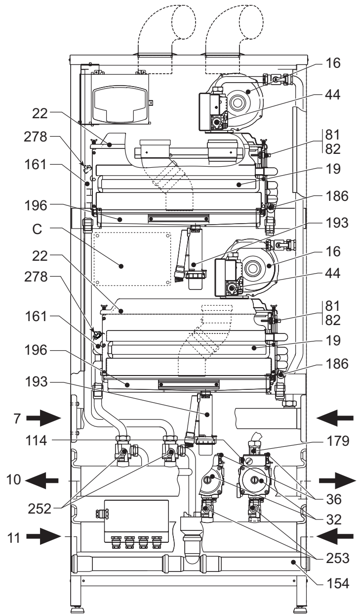
fig. 43 - Vista generale AURA COMBI 71/i-101/i
