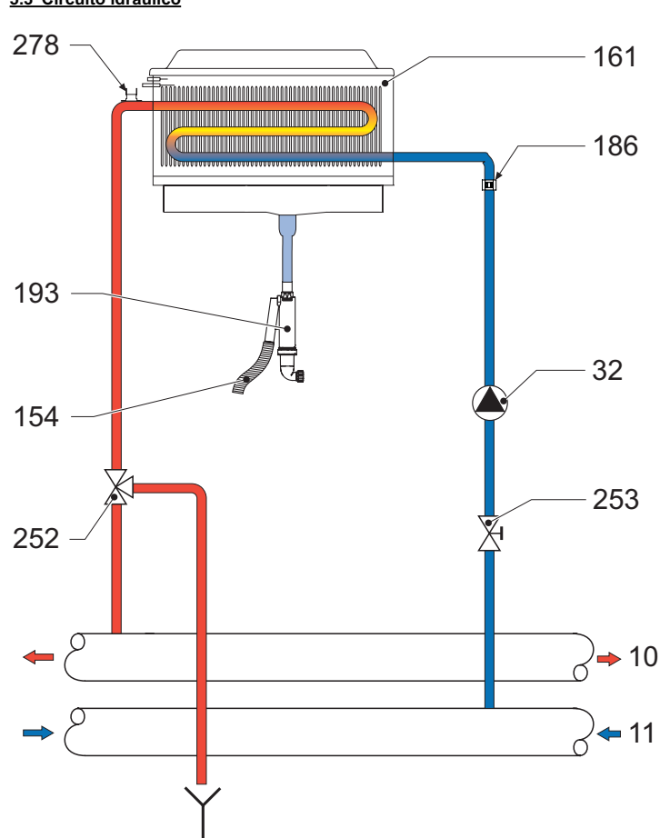
fig. 44 - Circuito idraulico AURA COMBI 51/i
