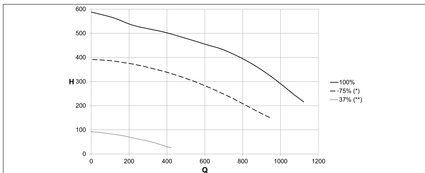
Fig. 23 Prevalenza disponibile ALISEA 28C
