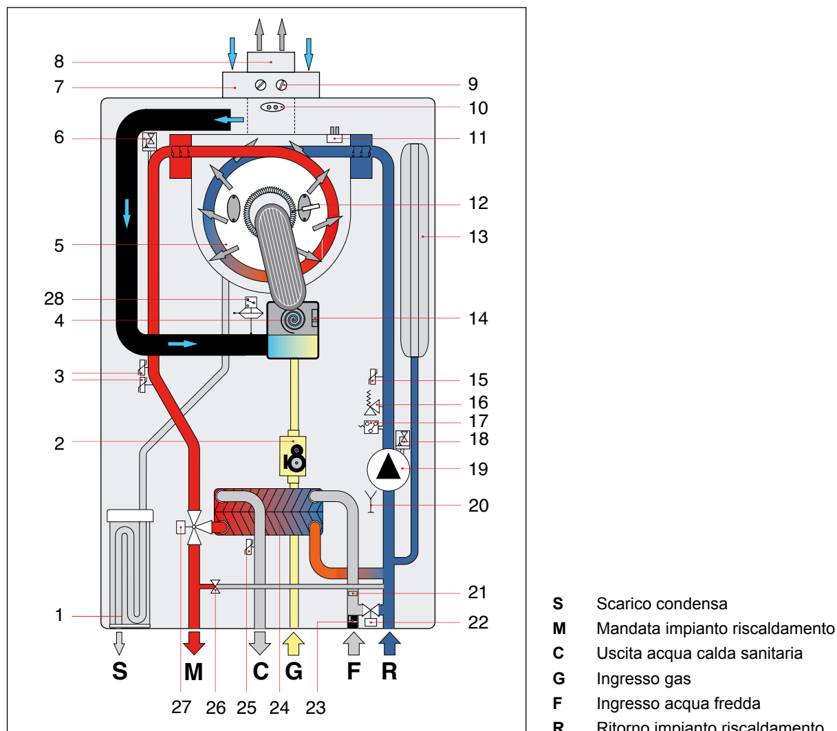
Fig. 4 Schema idraulico
