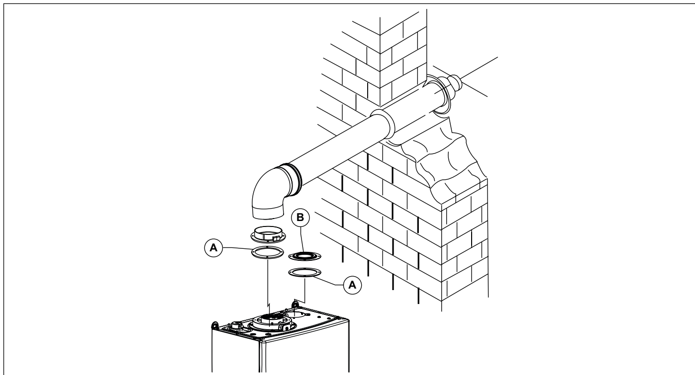
Fig. 13 Condotti coassiali tipo C13 - C33
