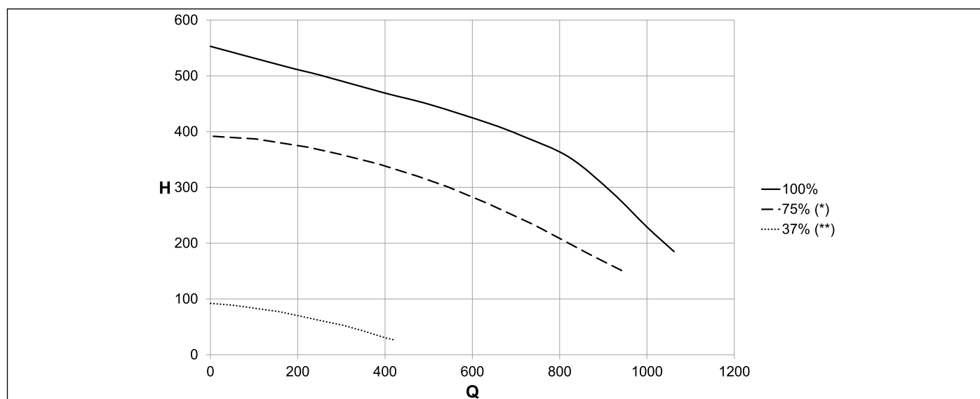
Fig. 22 Prevalenza disponibile ALISEA 24/28C
