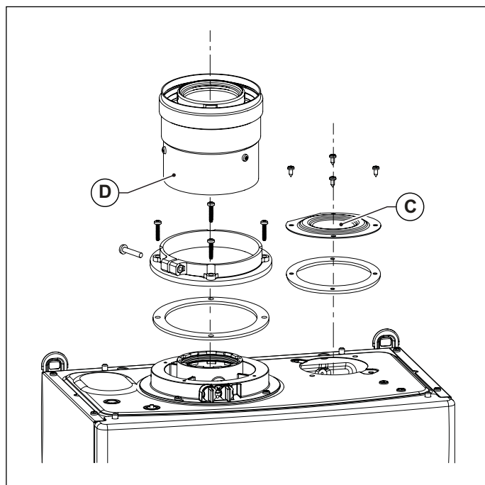
Fig. 7 Installazione kit coassiale
