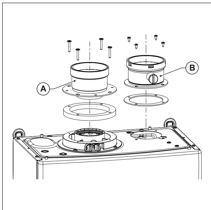
Fig. 6 Installazione kit sdoppiato
