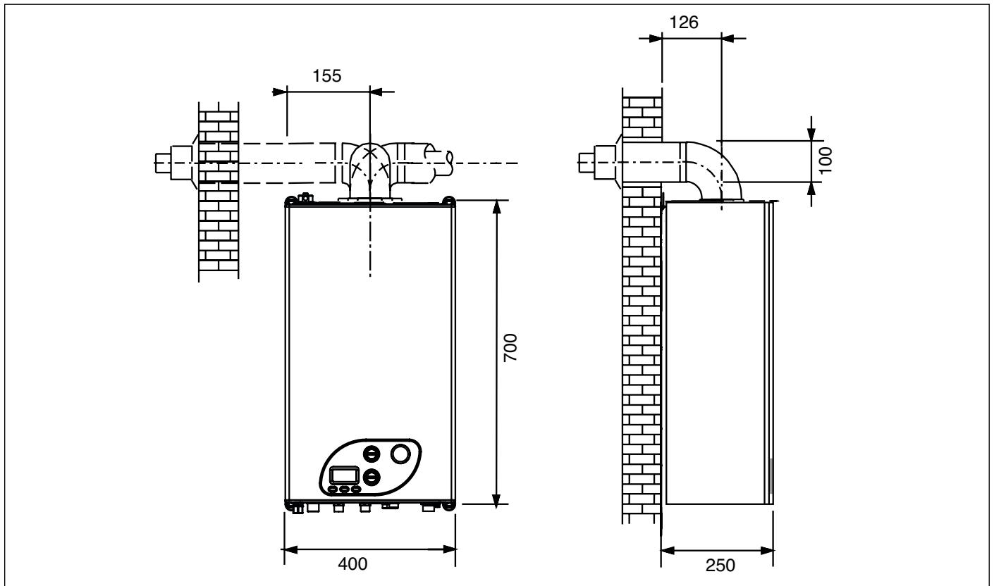
Fig. 14 Dimensioni condotti coassiali tipo C13 - C33
