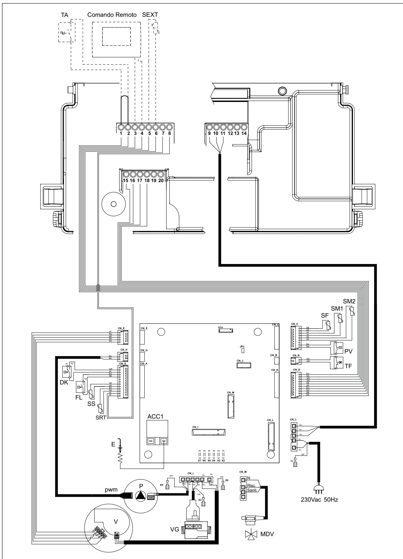
Fig. 24 Schema elettrico
