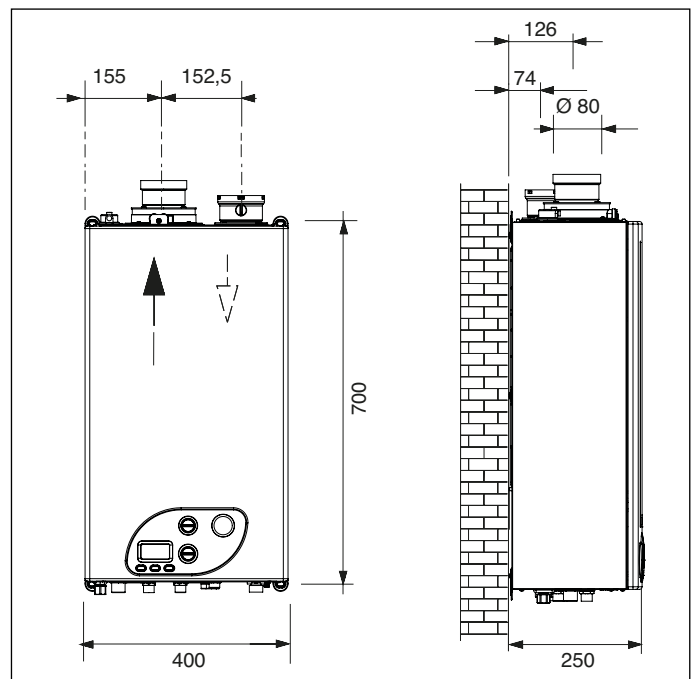
Fig. 16 Quote dimensionali condotti separati
