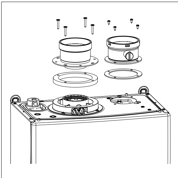
Fig. 15 Kit di sdoppiaggio
