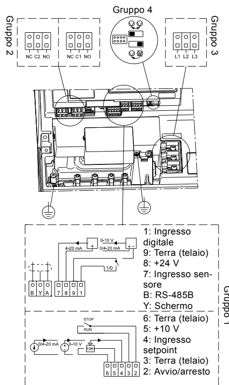
Fig. 110 Morsetti di connessione TPED serie 2000
