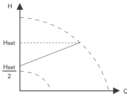
Fig. 52 Pressione proporzionale
