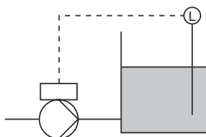
Fig. 65 Livello costante
