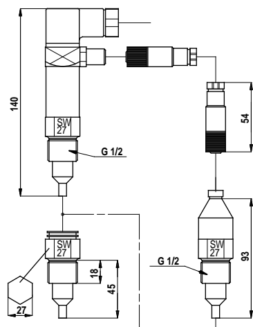
Fig. 116 Disegno dimensionale
