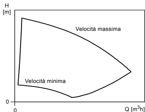
Fig. 26 Gamma di lavoro TPE3
