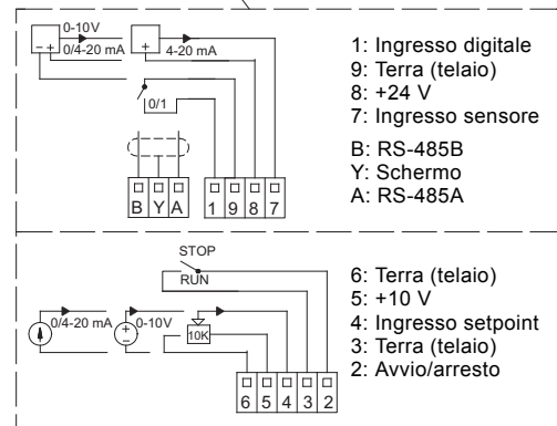
Fig. 107 Morsetti di connessione TPED serie 2000
