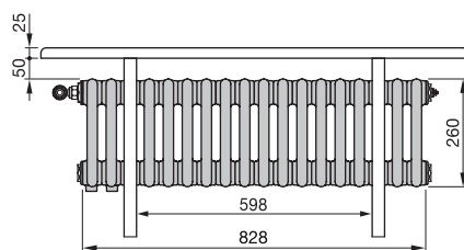
VISTA FRONTALE Modello 18 elementi
