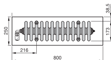
VISTA DALL'ALTO Modello 13 elementi
