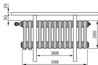
VISTA FRONTALE Modello 13 elementi
