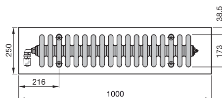
VISTA DALL'ALTO Modello 18 elementi
