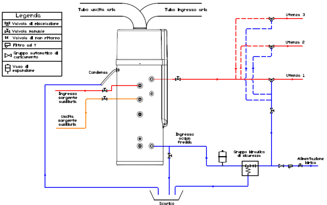
Schema di installazione in caso di fonte di calore ausiliaria Nota: il serpentino di integrazione ausiliario è presente solo nei modelli PD
