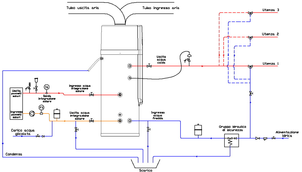
Schema di installazione in caso di ricircolo di acqua di integrazione solare Nota: il serpentino di integrazione solare è presente solo sui modelli PM e PD
