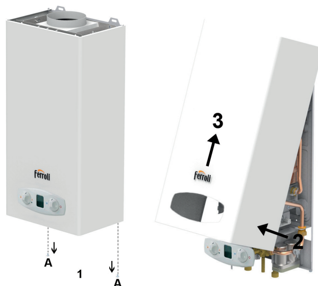
fig. 17 - Apertura del mantello
