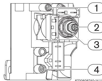
Fig. 12 Punti di controllo/regolazione gas
