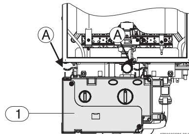
Fig. 10 Estrarre il quadro comandi
