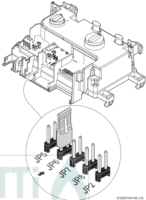
Fig. 16 Posizione morsetti e ponticello
