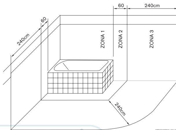
Fig. 4 Raffigurazione della Zona 3 (CEI 64-8)
