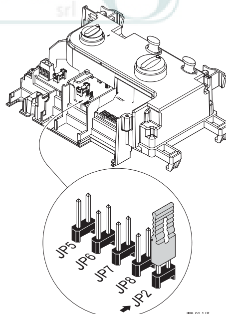
Fig. 20 Inserimento del ponticello JP2
