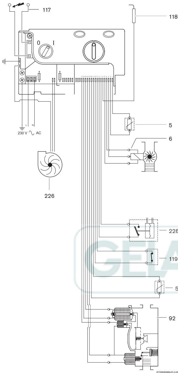
Fig. 3 Schema elettrico
