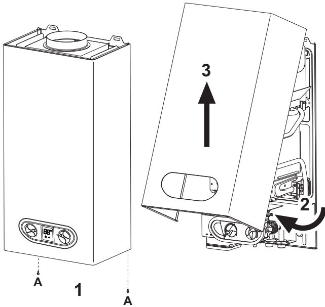
fig. 11 - Apertura mantello
