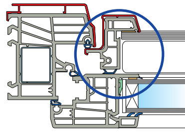
i lati della veneziana sono sormontati dal profilo dell'anta, garantendo una perfetta protezione dagli sguardi indesiderati
