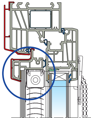
il cassonetto della veneziana è in tinta con il colore delle lamelle
