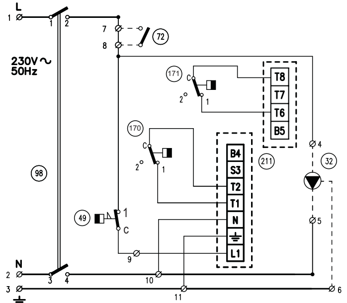
fig. 9 - Schema elettrico di principio G3G 80 - 98
