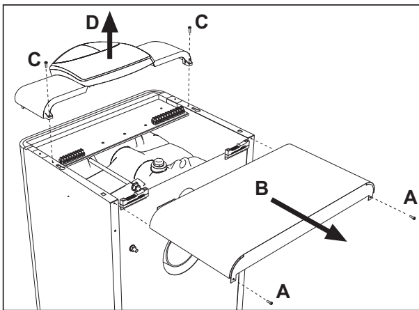
εικ. 44 - Πρόσβαση στη βάση ακροδεκτών
