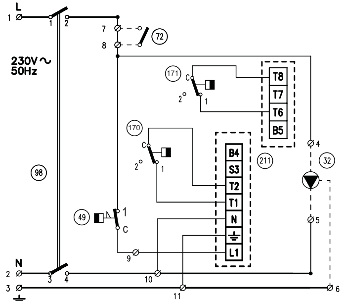
fig. 39 - Schéma électrique de base G3G 80 - 98
