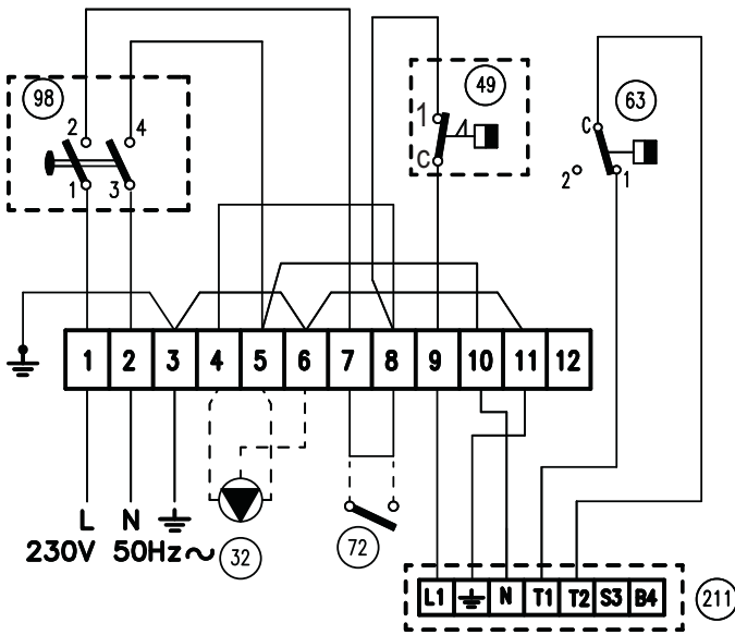
ΕΙΚ. 48 - Διάγραμμα συνδεσμολογίας G3G 32χ63
