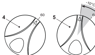
fig. 33 - Réglage de la température modèle G3G 80 - 98
