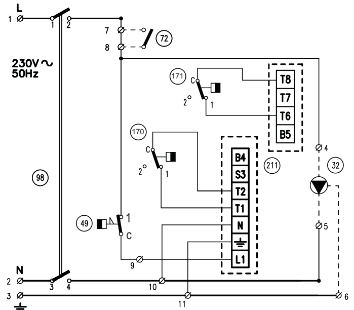
ΕΙΚ. 49 - Ηλεκτρικό σχεδιάγραμμα αρχής λειτουργίας G3G 80 - 98
