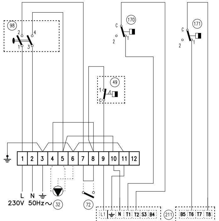
fig. 40 - Schéma électrique de raccordement G3G 80 - 98
