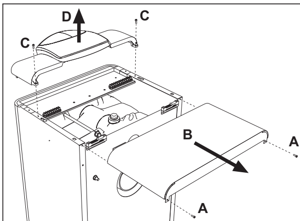
fig. 4 - Accesso alla morsettiera
