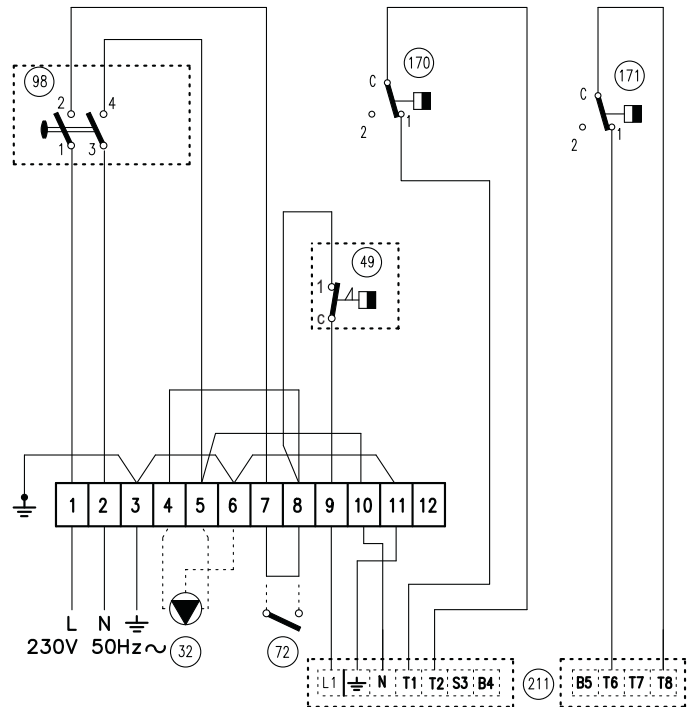
ΕΙΚ. 50 - Σχεδιάγραμμα ηλεκτρικής σύνδεσης G3G 80 - 98
