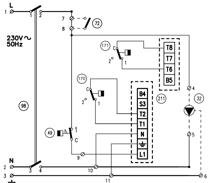
fig. 19 - Esquema eléctrico general G3G 80 - 98
