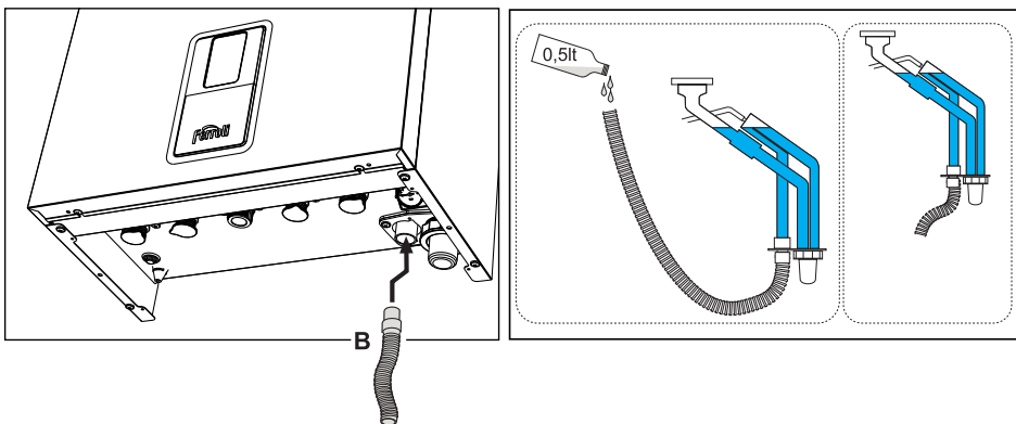
fig. 38- Racordarea evacuării condensului
