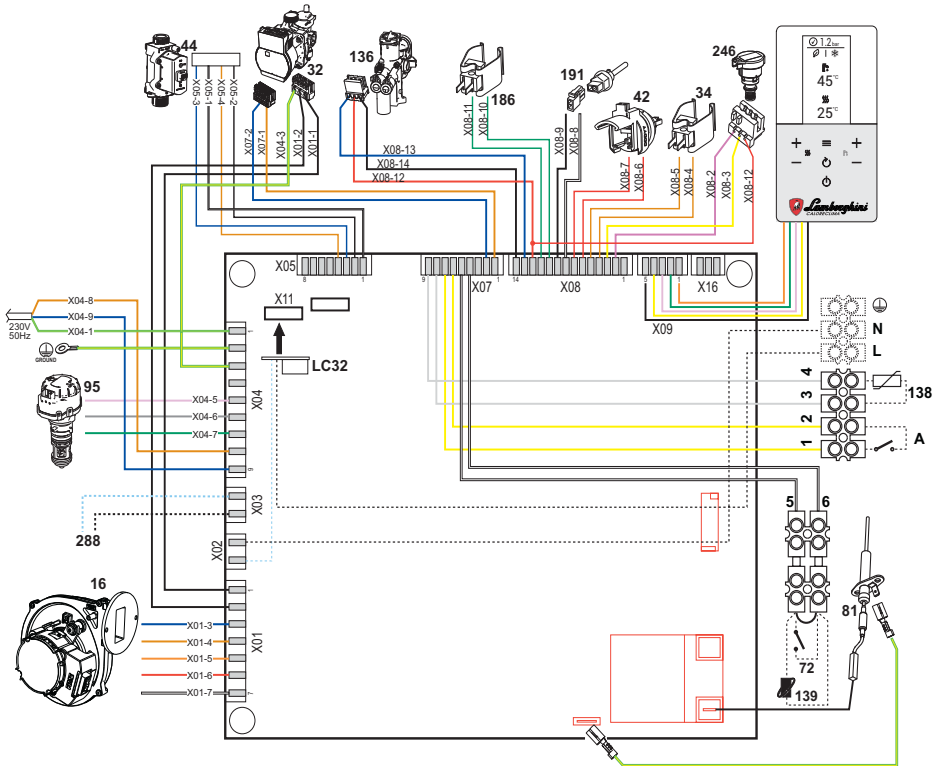
fig. 67 - Schema elettrico
