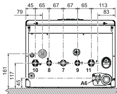
fig. 61- Vista inferior
