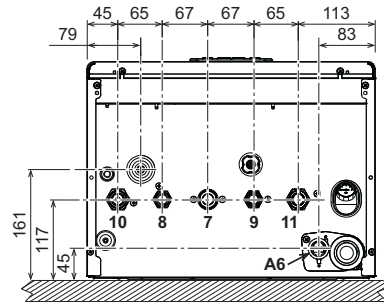
εικ. 62- Άνωψη
