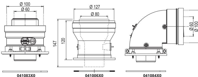
wygląd 32- Akcesoria wyjściowe do przewodów współosiowych
