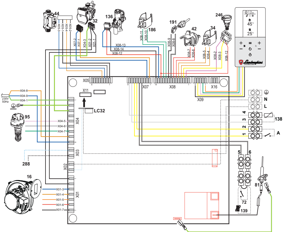
fig. 66- Schema electrică
