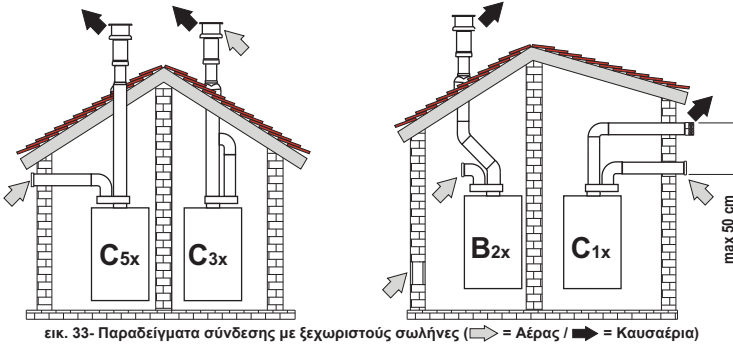
εικ. 33- Παραδείγματα σύνδεσης με ξεχωριστούς σωλήνες (⇨ = Αέρας / ⇨ = Κουσαερία)
