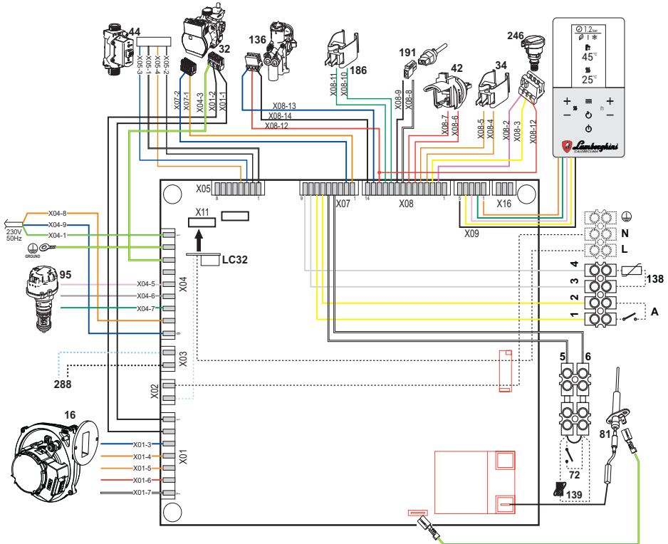
fig. 66- Wiring diagram
