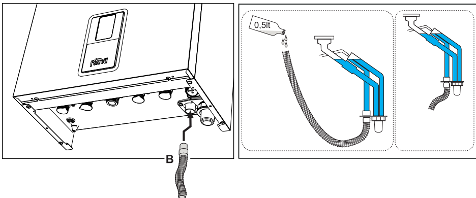
fig. 38- Conexión de la descarga de condensado
