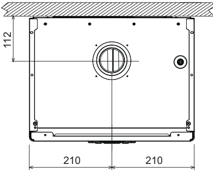
εικ. 61- Κάτωψη
