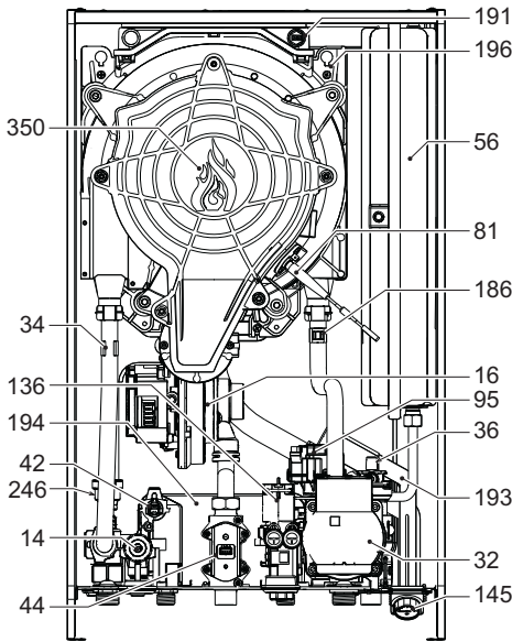
fig. 62- Vedere generală
