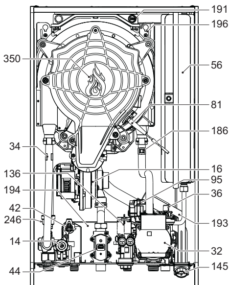
εικ. 63- Γενική όψη
