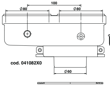
fig. 34- Accesorio inicial para conductos separados
