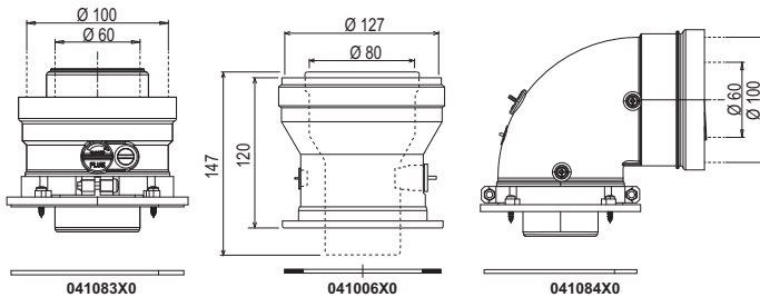
fig. 32 - Accessori di partenza per condotti coassiali
