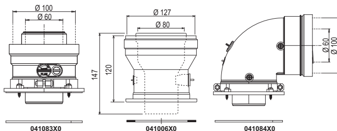
fig. 32- Accesorii de pornire pentru conducte coaxiale
