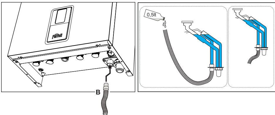
wygląd 38- Podłączenie spustu kondensatu
