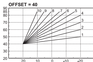
fig. 25- Exemplu de deplasare paralelă a curbelor de compensare
