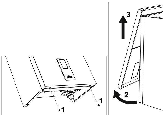
εικ. 42- Άνοιγμα μπροστινού πύνακα
