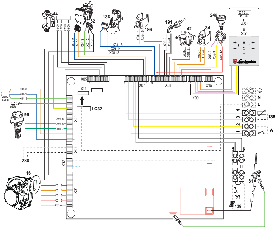
fig. 66- Esquema eléctrico
