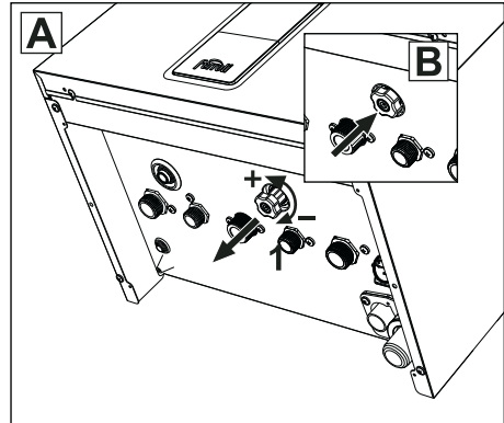
fig. 26 - Manopola di carica
