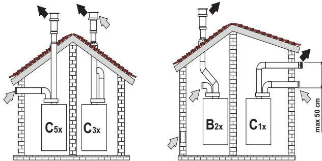
wygląd 33- Przykłady połączenia przewodami oddzielnymi (⇐ = Powietrze / ➡ = Spaliny)
