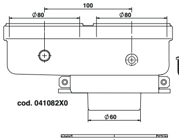
εικ. 34- Εξάρτημα σύνδεσης για ξεχωριστούς αγωγούς
