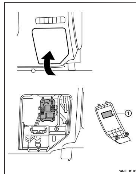
Scatola portafusibili secondaria (modelli con guida a sinistra)
