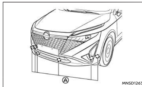
Modelli con 6 sensori di parcheggio
