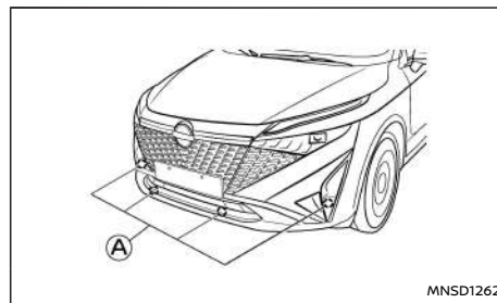
Modelli con 4 sensori di parcheggio
