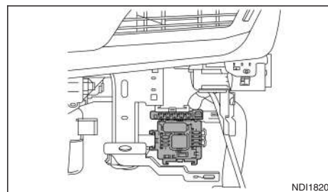
Scatola portafusibili secondaria (modelli con guida a sinistra)
