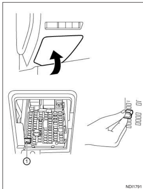
Scatola portafusibili principale (modelli con guida a sinistra)
