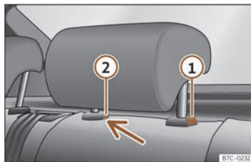
Fig. 88 Poggiatesta posteriore: smontaggio.
