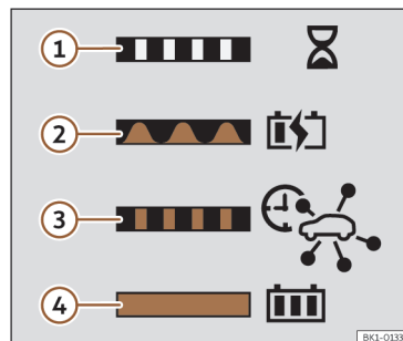
Fig. 60 All'interno del coperchio della presa di carica della batteria: adesivo con informazioni sull'indicatore del processo di carica.
