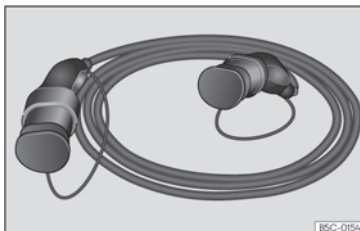
Fig. 64 Cavo di ricarica per stazioni di ricarica con corrente alternata (CA).
