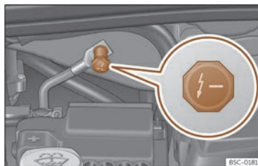
Fig. 175 Nel vano anteriore: presa per l'avviamento d'emergenza (terminale di massa).
