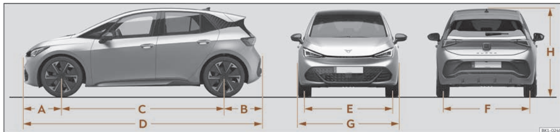
Fig. 204 Dimensioni
