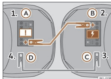
Fig. 176 Schema di collegamento dei cavi di emergenza.
