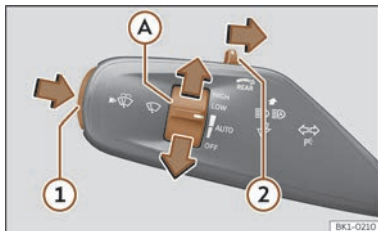
Fig. 97 Uso del tergicristalli e del tergilunotto.
