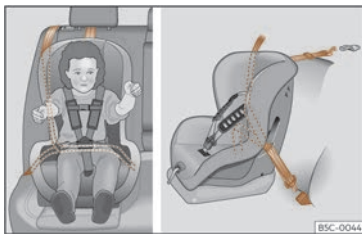
Fig. 44 Nei sedili posteriori: montaggio del sedile per bambini.
