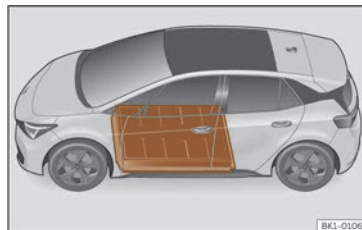
Fig. 52 Alloggiamento della batteria ad alta tensione
