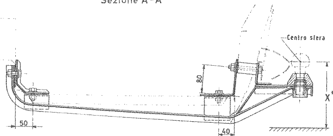
Sezione A-A
