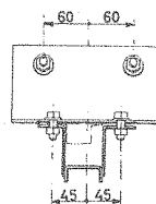
Sezione F-F
