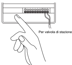
FIGURA 18: Collegamento dei fili delle valvole
