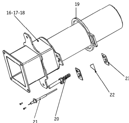
BRUCIATORE
