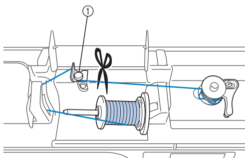
① Guida filo dell'avvolgimento della spolina
