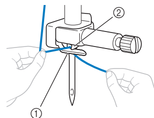
① Guida del filo della barra dell'ago ② Linguetta
