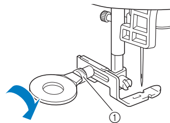
① Vite di posizionamento
