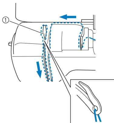
① Dischi di tensione
