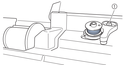
① Sostegno della guida dell'avvolgitore spolina (a chiave)
