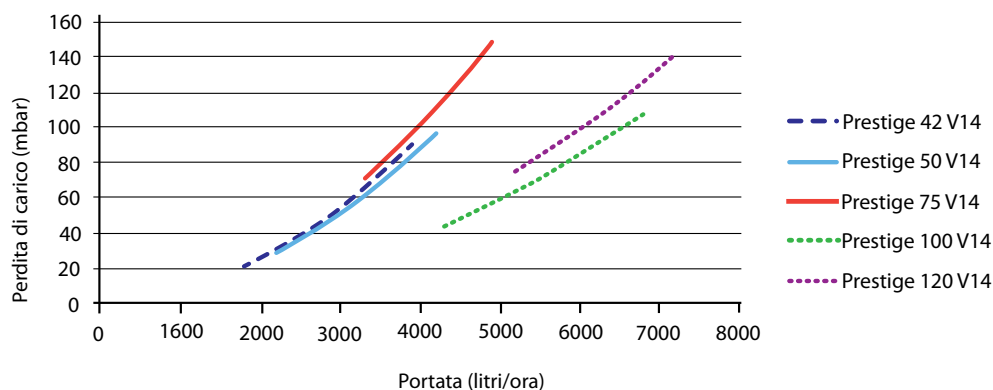
Prestige 42-50-75-100-120 Solo - perdita di carico in base alla portata
