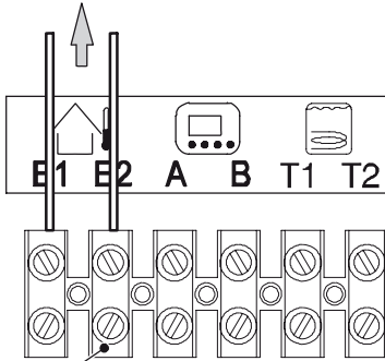
Morsettiere collegamento sonda esterna Fig. 5.46
