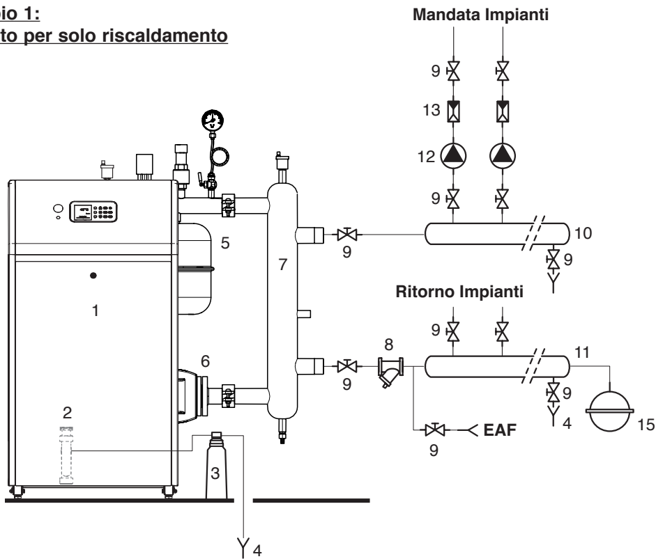
Esempio 2: Impianto per riscaldamento e produzione di A.C.S. con bollitore a valle del separatore idraulico
