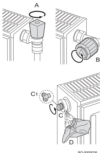
Fig.68 Deareazione impianto
