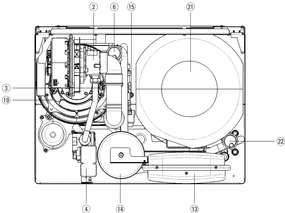
Vista superiore Althea S (modelli BI)
