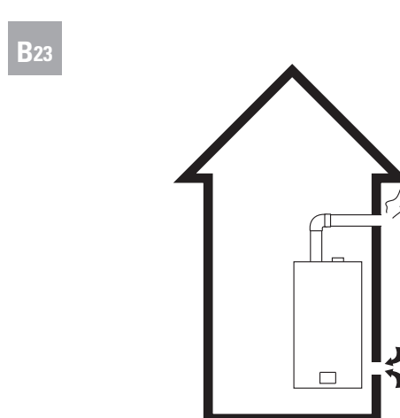
3.8.8 Scarico fumi a parete ed aspirazione aria in ambiente (solo in ambienti correttamente ventilati)
