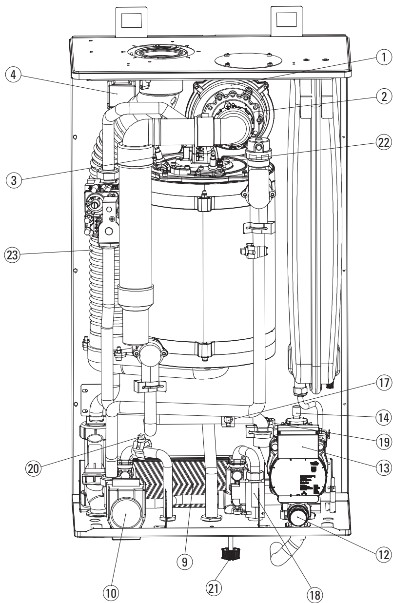
Vista superiore Althea SR (modelli K, B e C)
