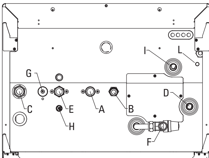
Vista inferiore Althea S (modelli BI): attacchi
