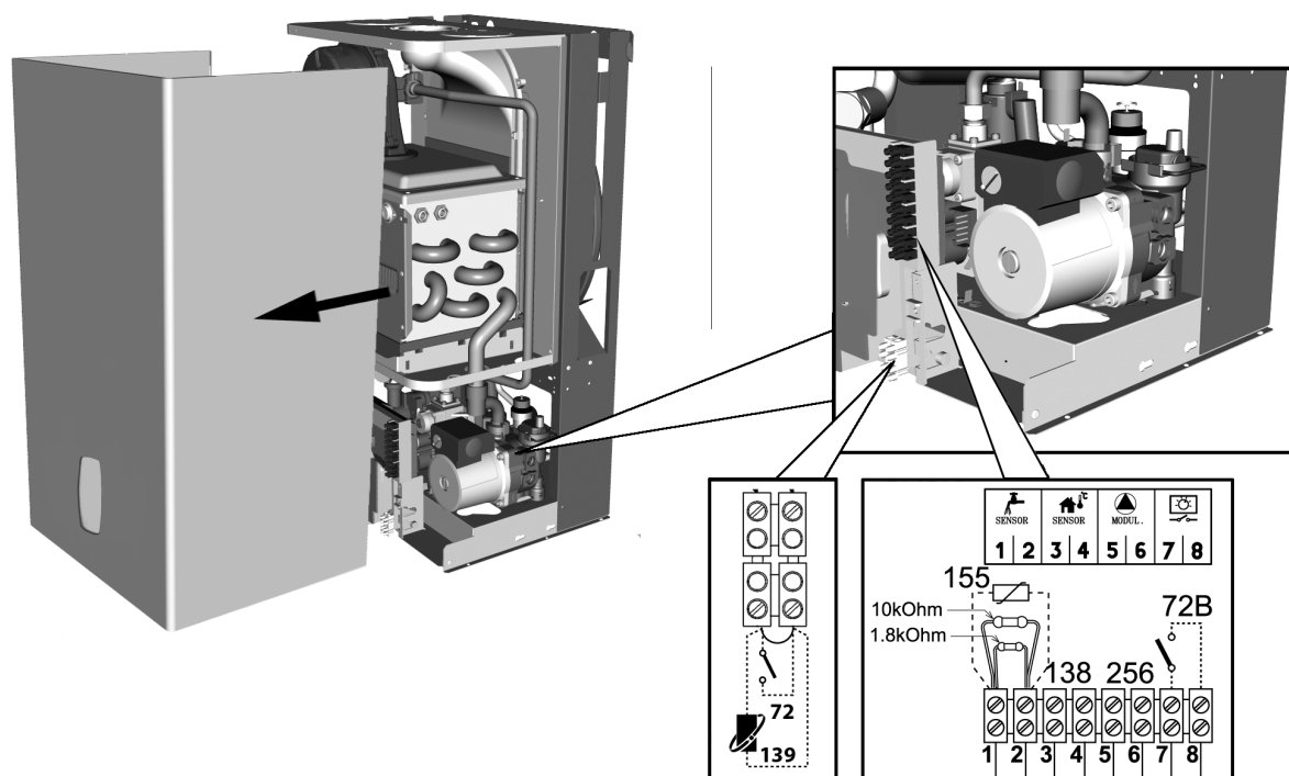
fig. 17 - Accesso alla morsettiera
