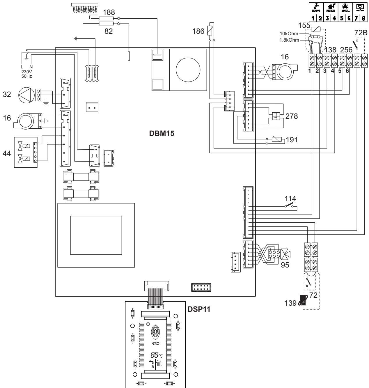
fig. 32 - Schema elettrico
