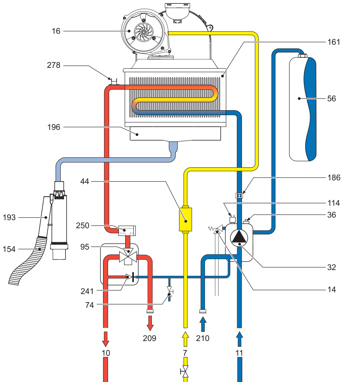
fig. 31 - Circuito idraulico
