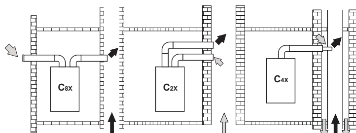
fig. 19 - Exemple de racordare la hornuri (⇨ = Aer / ⇨ = Gaze arse)
