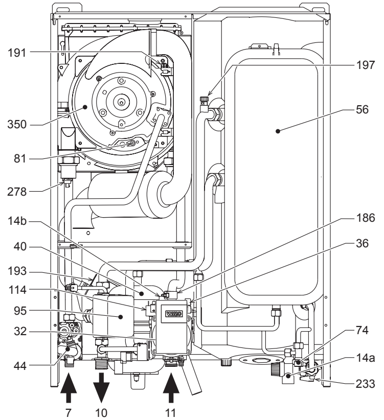
fig. 26 - Vista frontal
