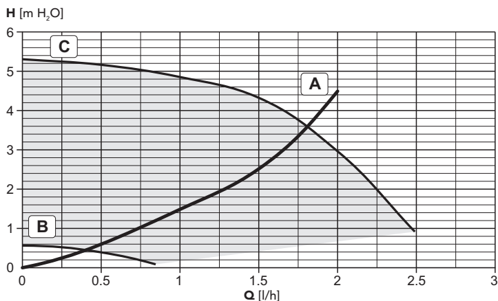
рис. 28 - Потеря напора/Напор циркуляционных насосов BLUEHELIX 25 K 50
