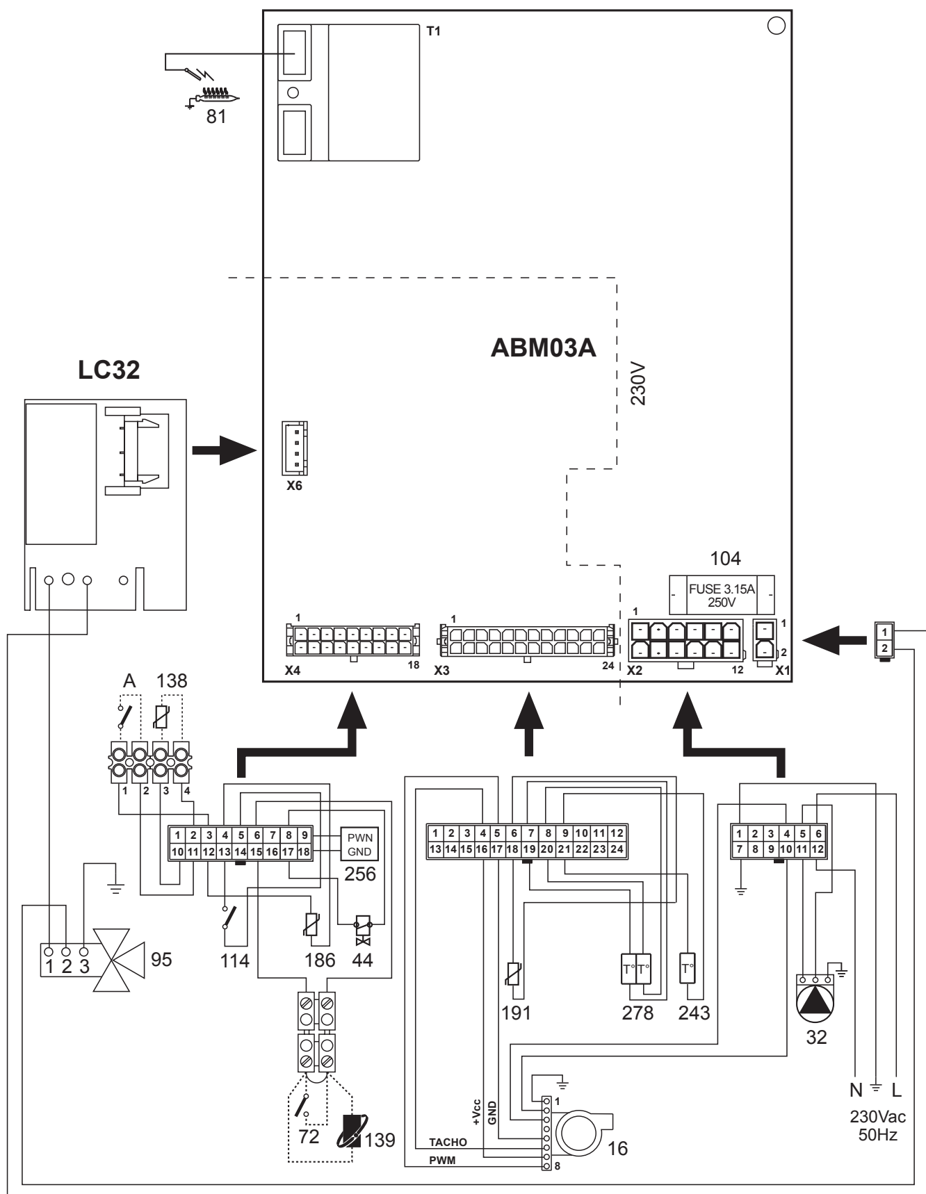
fig. 29 - Schemă electrică
