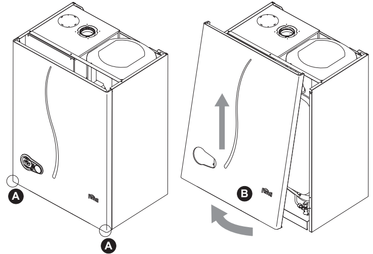
şek. 24 - Ön paneli açma
