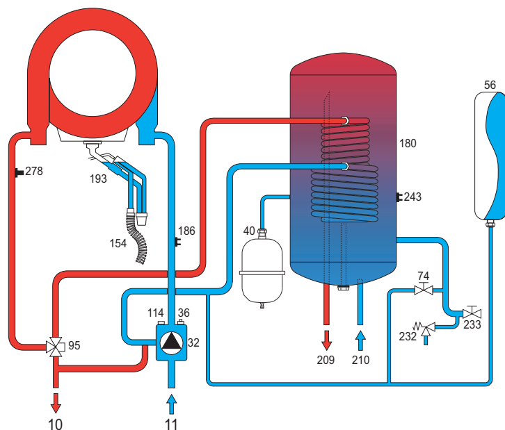
fig. 27 - Circuit hydraulique
