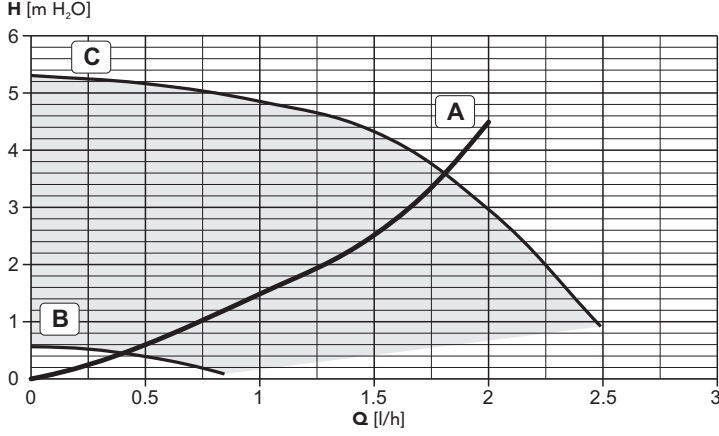
şek. 28 - Sirkülör yük / basınç kayıpları BLUEHELIX 25 K 50
