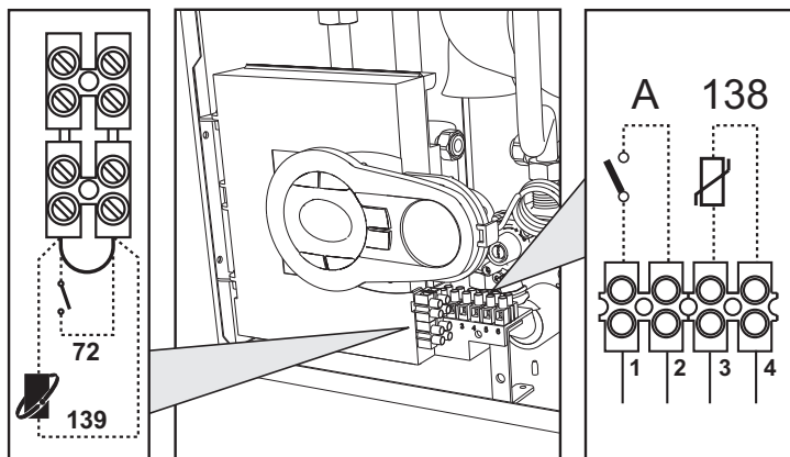
fig. 14 - Accesso alla morsettiere
