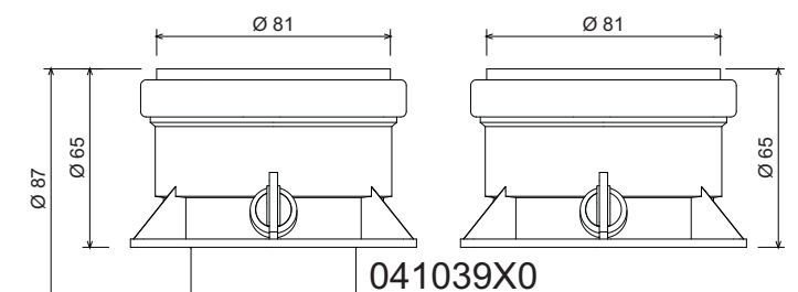
fig. 18 - Accessoire de départ pour conduits séparés
