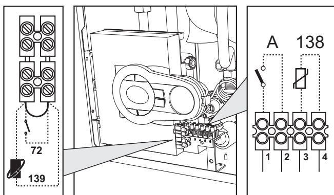
fig. 14 - Accès au bornier
