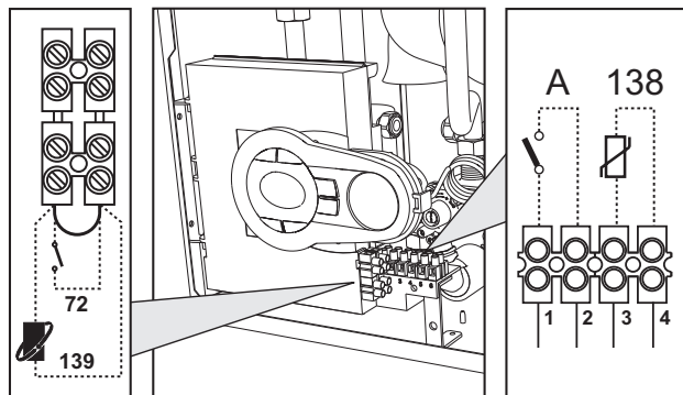
рис. 14 - Доступ к клеммной панели
