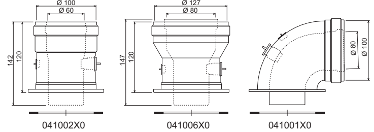
şek. 16 - Koaksiyal kanallar için çıkış aksesuarları
