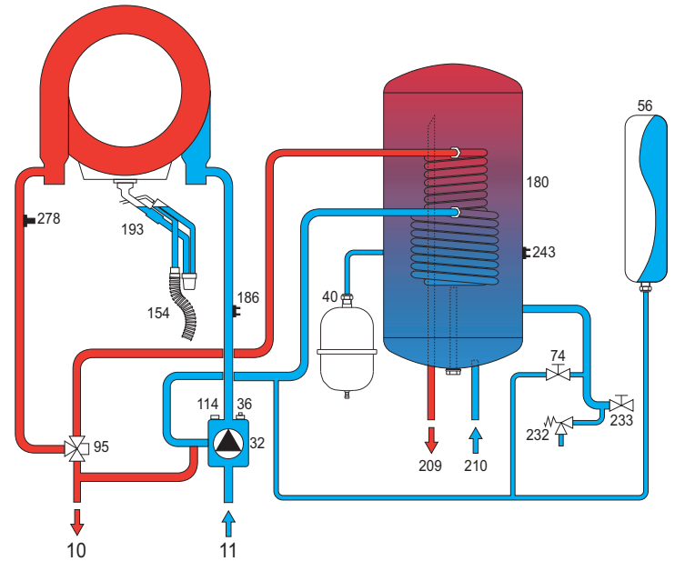
fig. 27 - Circuito idraulico
