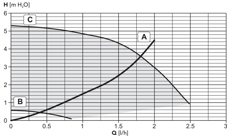
fig. 28 - Pérdida de carga/altura manométrica bomba BLUEHELIX 25 K 50
