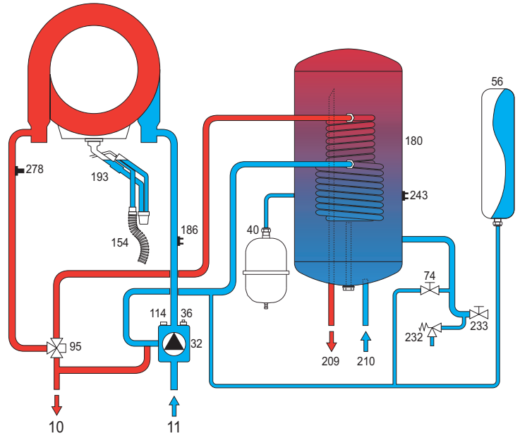
şek. 27 - Hidrolik devre
