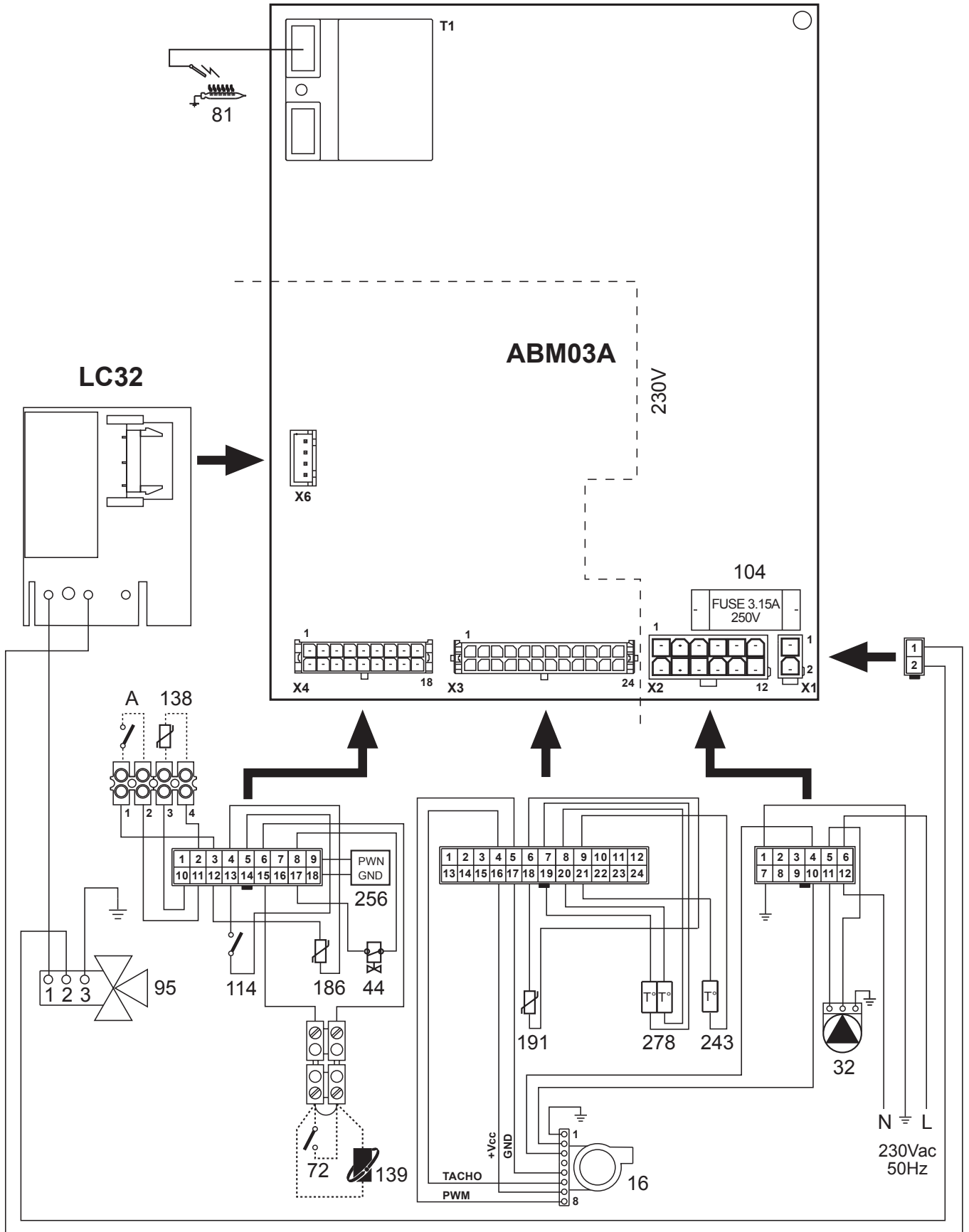
şek. 29 - Elektrik şeması
