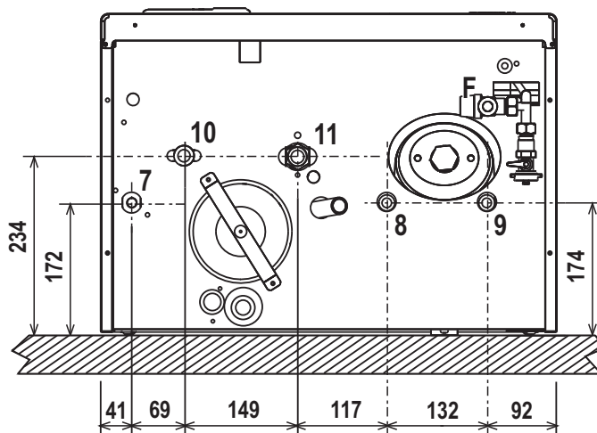
fig. 13 - Conexiones hidráulicas
