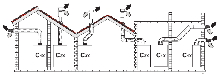
рис. 15 - Примеры присоединения с помощью коаксиальных труб (→ = Воздух / → = Дымовые газы)
