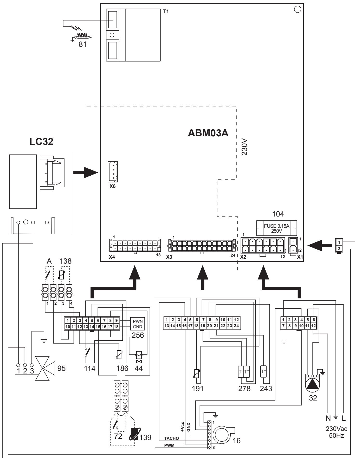
fig. 29 - Schema elettrico
