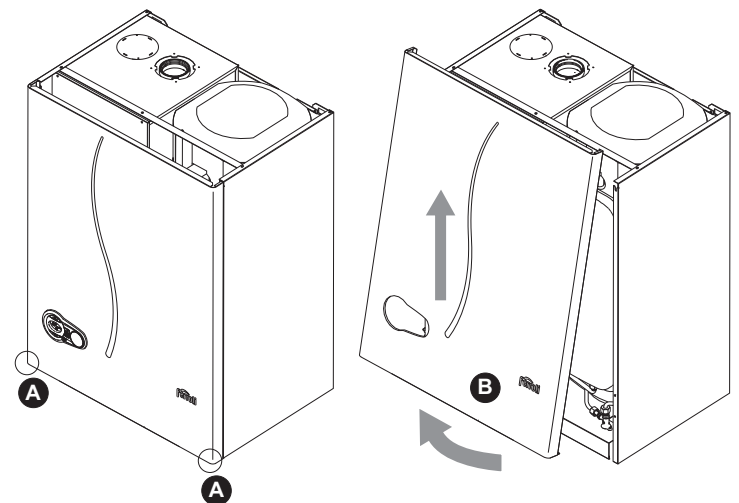
fig. 24 - Ouverture du panneau avant
