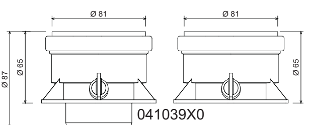
мал. 18 Початковий елемент для відокремлених трубопроводів
