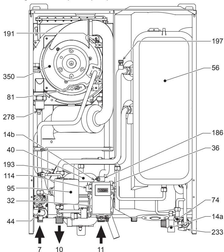
fig. 26 - Vue de face
