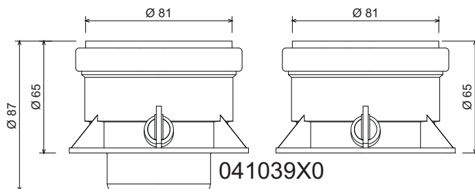
fig. 18 - Accesorii de pornire pentru conducte separate
