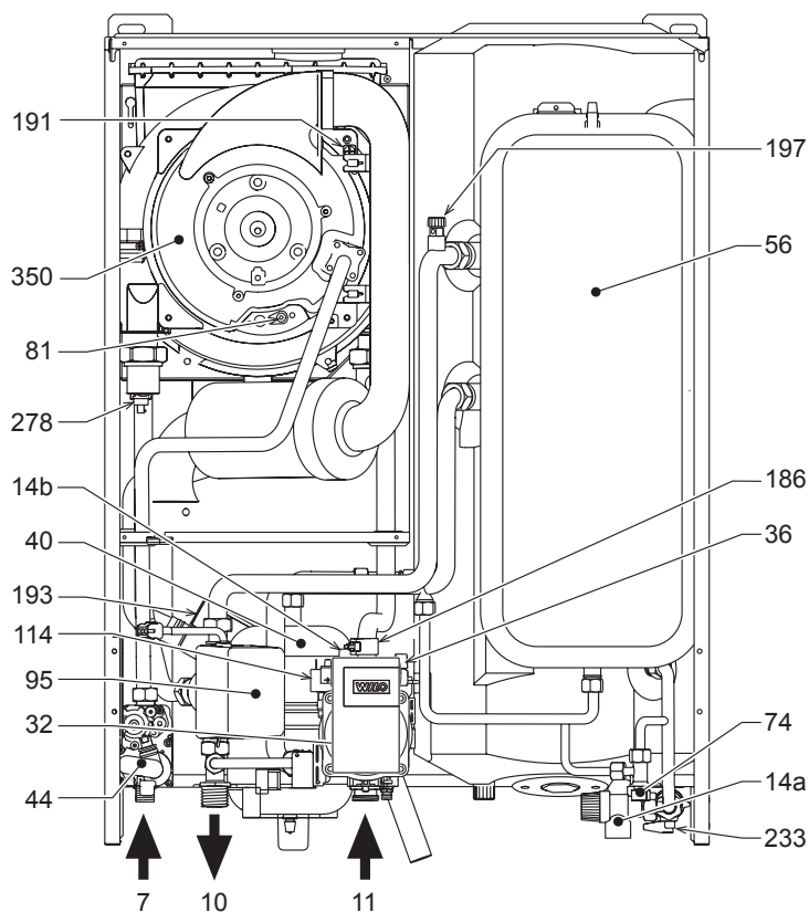
рис. 26 - Вид спереди
