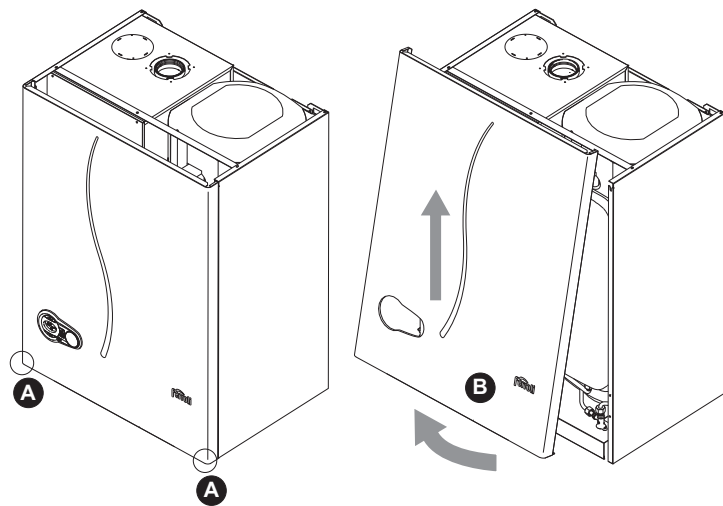
мал. 24 - Відкриття передньої панелі
