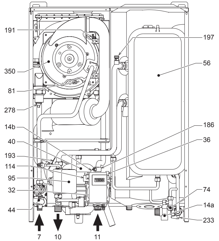
fig. 26 - Vista frontale
