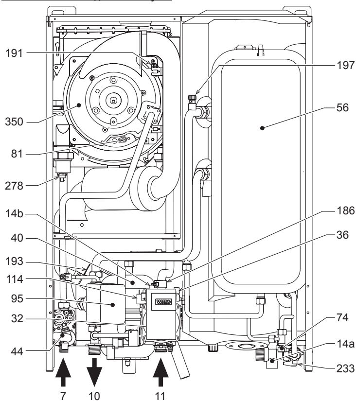
мал. 26 - Вигляд спереду
