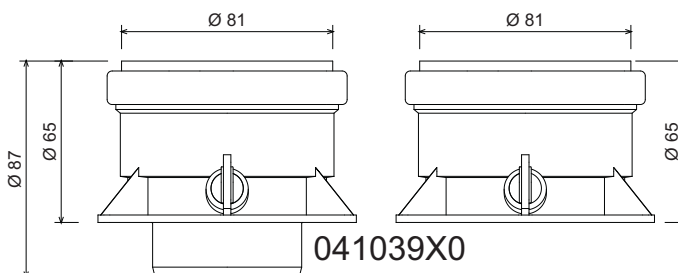
fig. 18 - Accessorio di partenza per condotti separati
