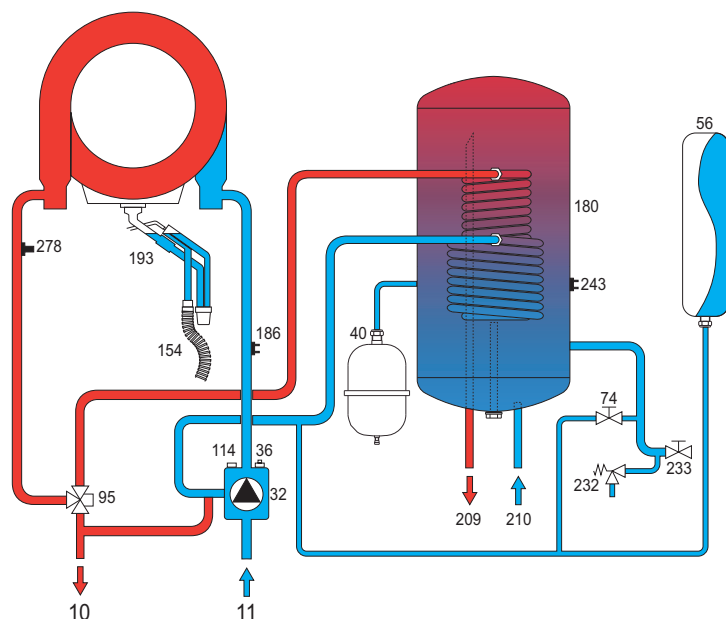
fig. 27 - Circuitul hidraulic
