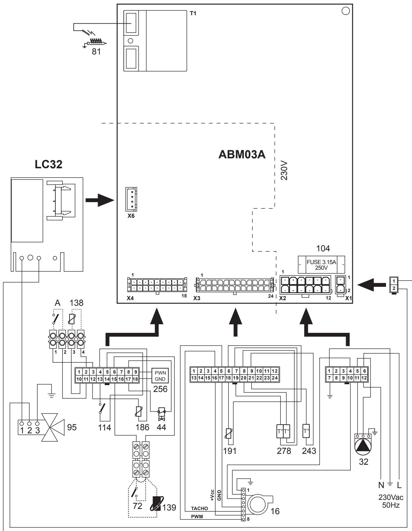
fig. 29 - Esquema eléctrico
