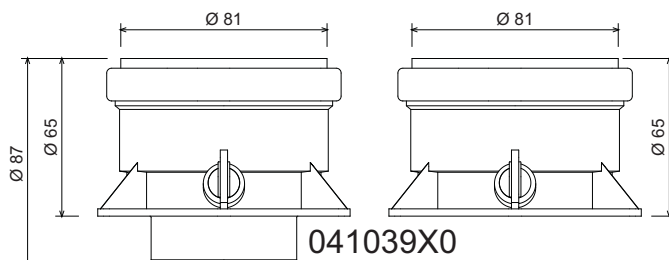
fig. 18 - Accesorio inicial para conductos separados
