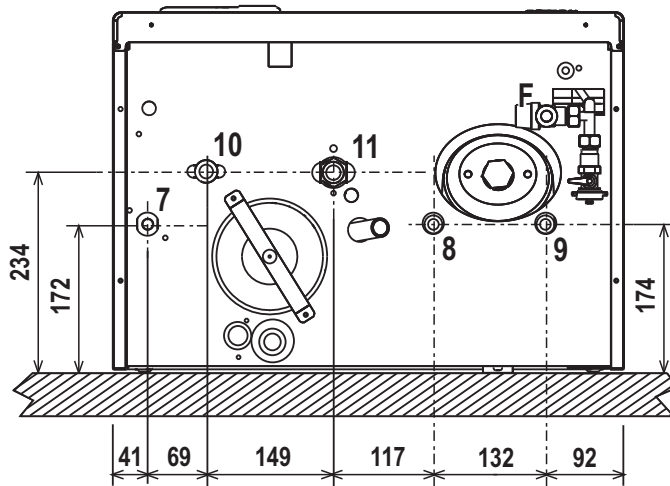
мал. 13 - Водопровідні штуцери
