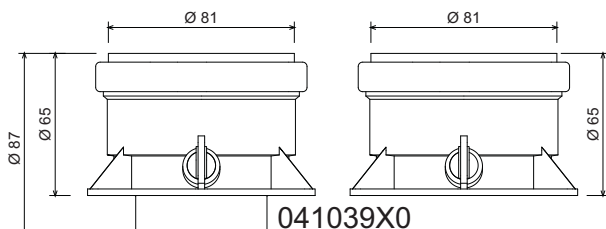
рис. 18 - Соединительный элемент для отдельных труб
