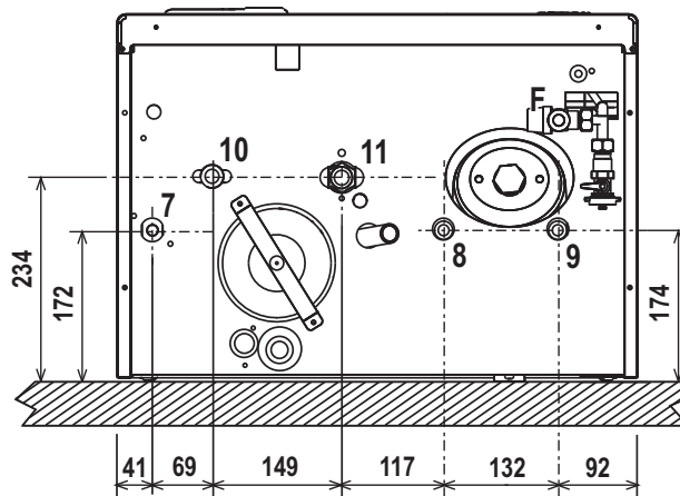
рис. 13 - Гидравлические штуцеры
