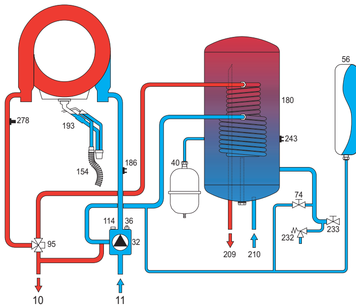
мал. 27 - Гідравлічний контур
