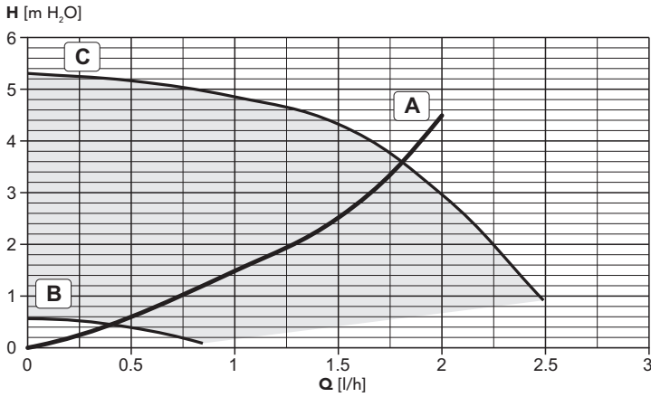
мал. 28 - Втрати напору / Напір циркуляційних насосів BLUEHELIX 25 K 50
