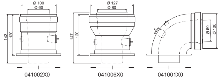
мал. 16 - Початкові елементи для коаксіальних трубопроводів
