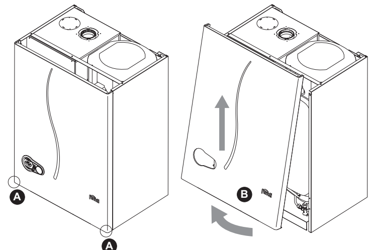
fig. 24 - Deschiderea panoului frontal
