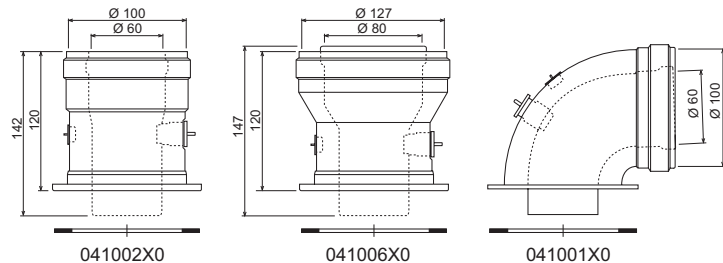
рис. 16 - Элементы для коаксиальных воздухопроводов
