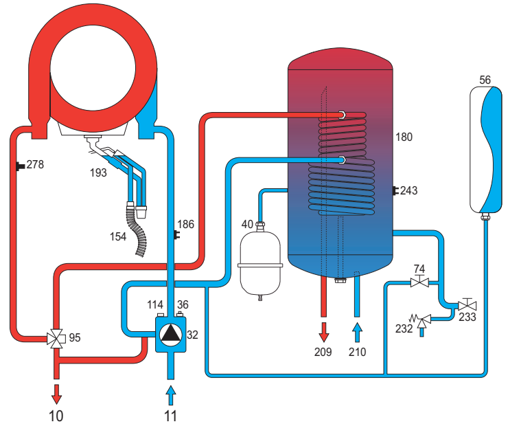
fig. 27 - Circuito hidráulico
