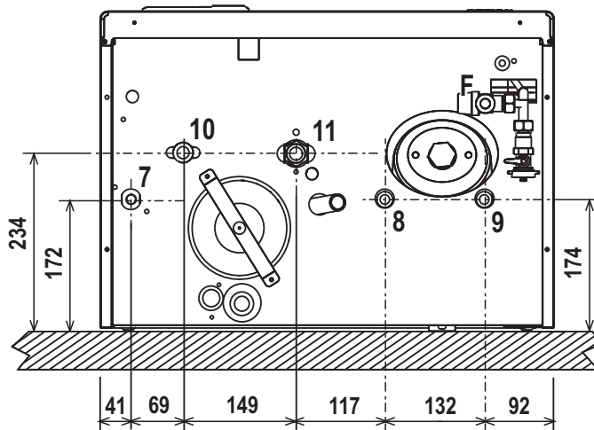
fig. 13 - Attacchi idraulici
