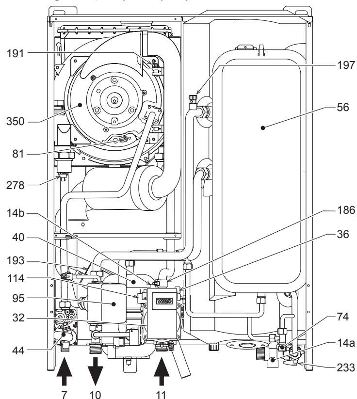
fig. 26 - Vedere frontală
