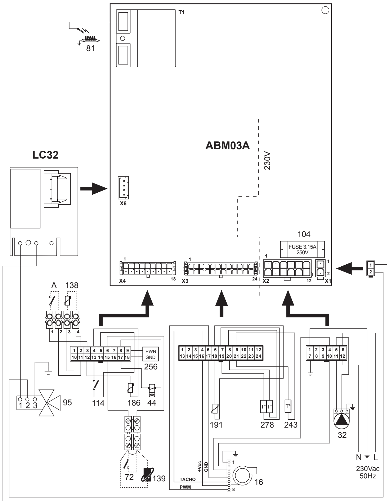
мал. 29 - Електрична схема
