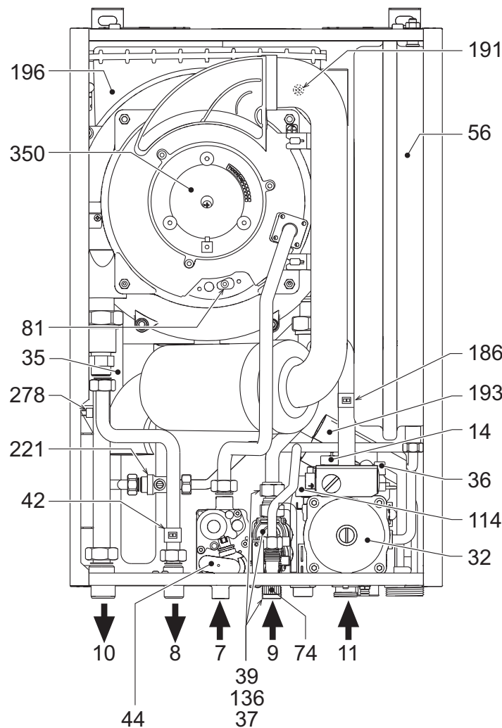
fig. 26 1.4 Vue générale
