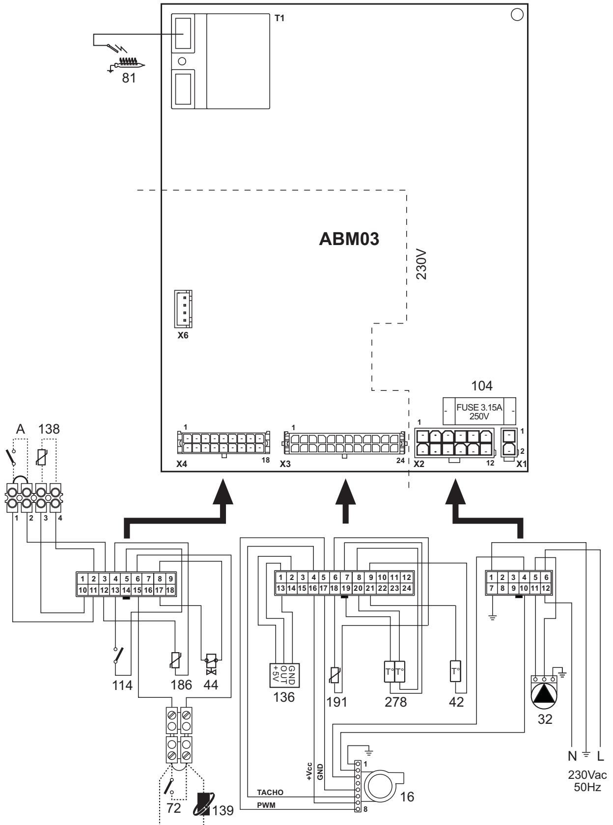
fig. 30 - Esquema eléctrico
