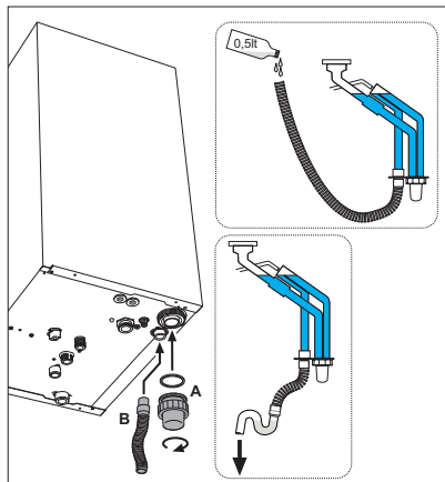
мал. 20 - Підключення для зливу конденсату
