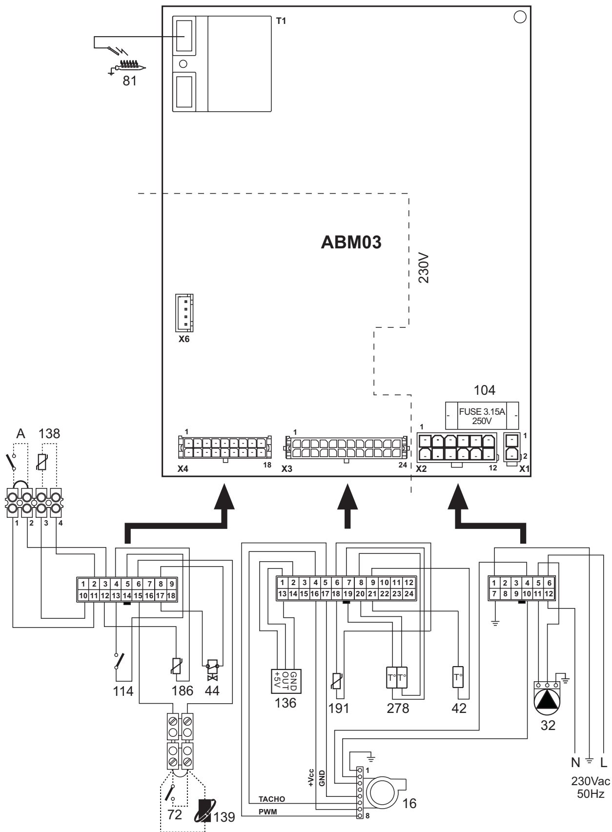
fig. 30 - Schema elettrico
