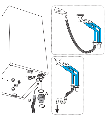
рис. 20 - Подсоединение трубы для слива конденсата
