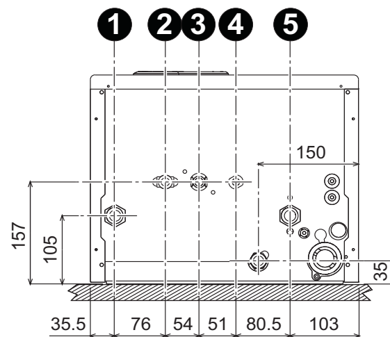
fig. 13 - Attacchi idraulici
