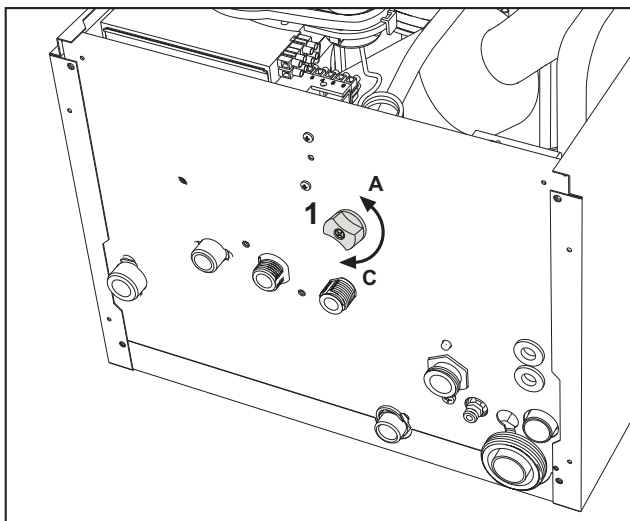
fig. 12 - Filling knob
