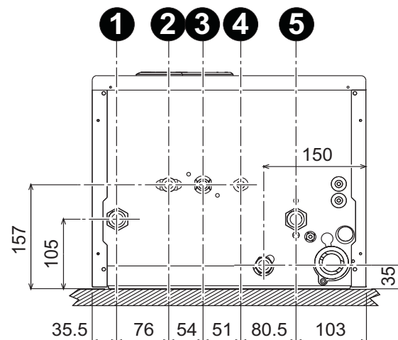
fig. 13 - Conexiones hidráulicas
