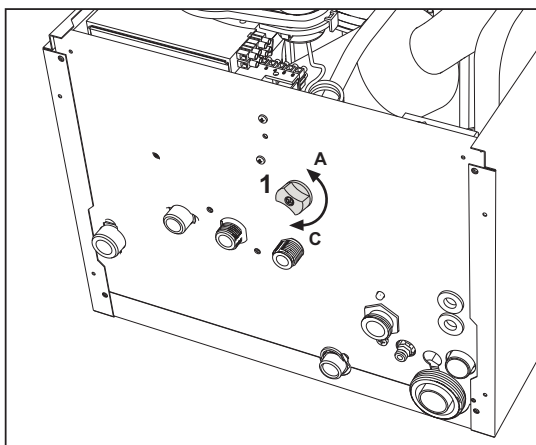
мал. 12 - Кран для заправлення
