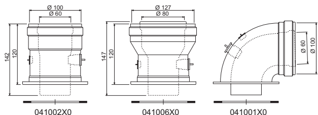
рис. 16 - Элементы для коаксиальных воздухопроводов
