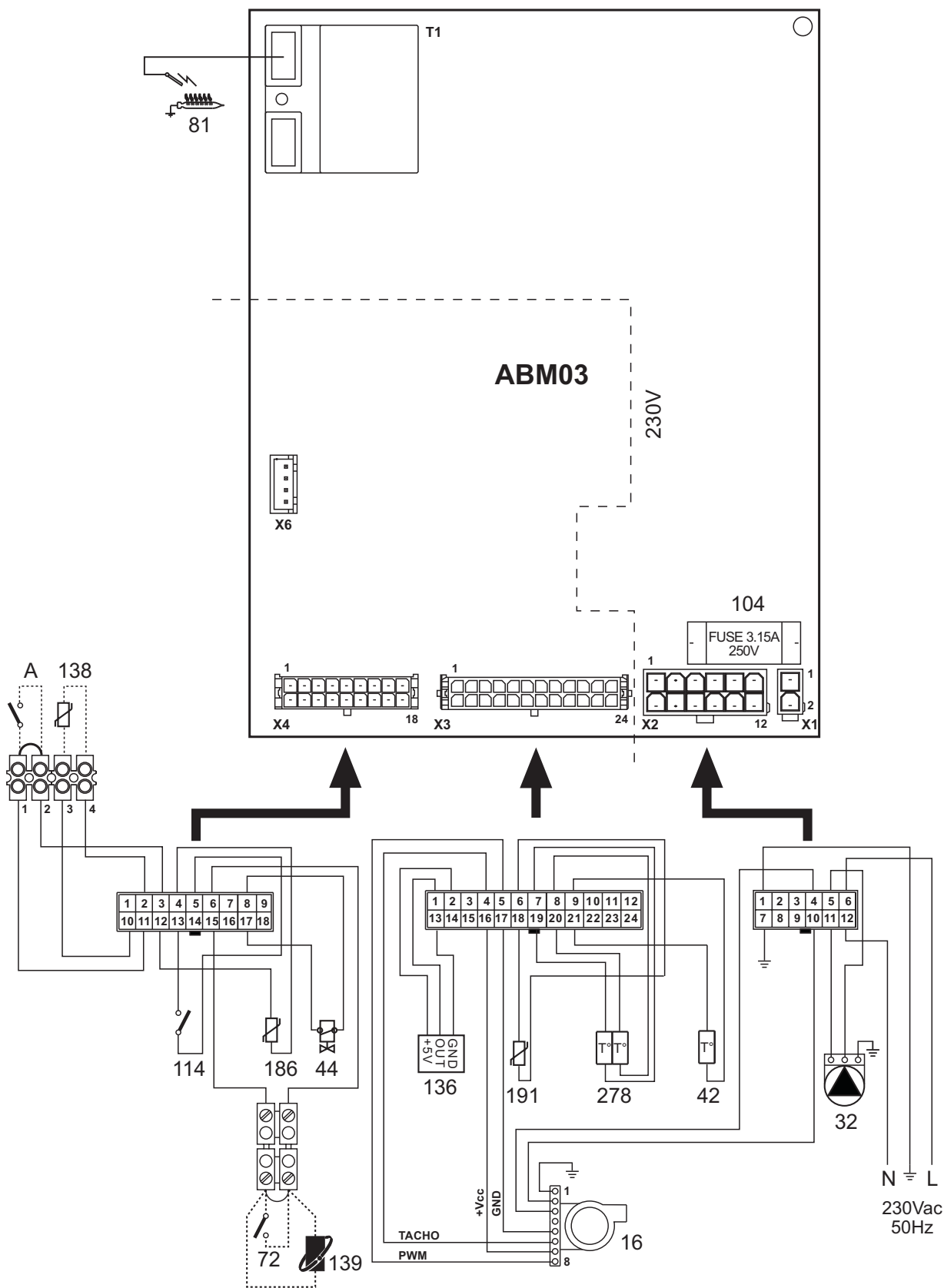
fig. 30 - Schéma électrique
