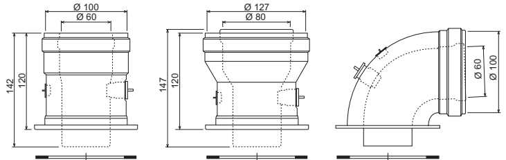
мал. 16 - Початкові елементи для коаксіальних трубопроводів
