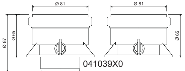
şek. 18 - Ayrı kanallar için çıkış aksesuarları
