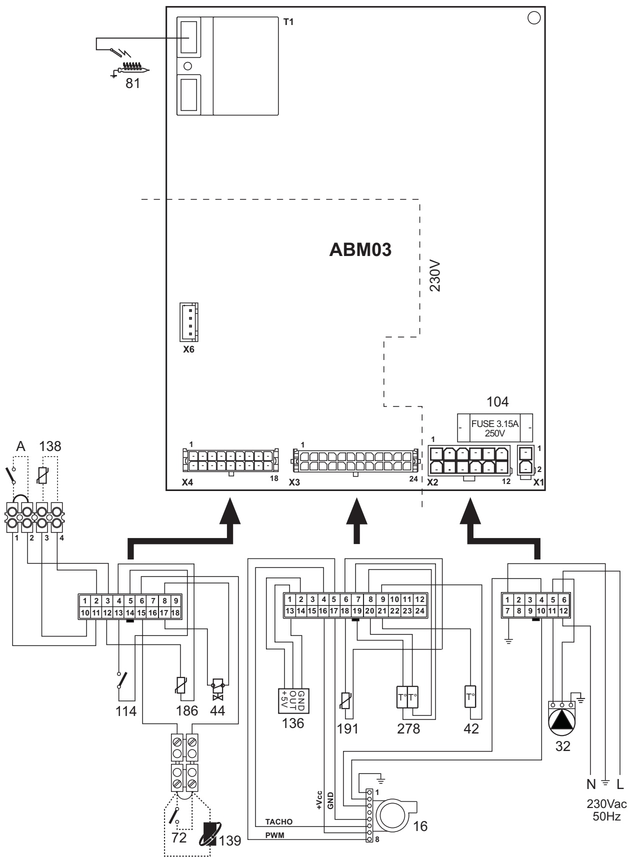
рис. 30 - Электрическая схема
