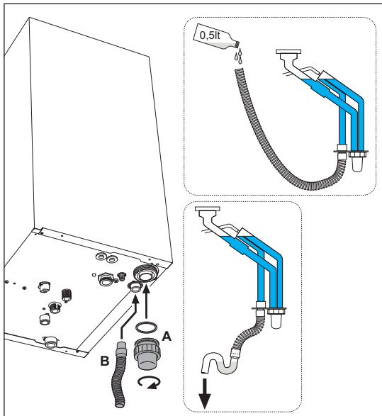
şek. 20 - Yoğuşma tahliye bağlantısı
