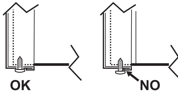
fig. 25 - Position correcte du panneau avant
