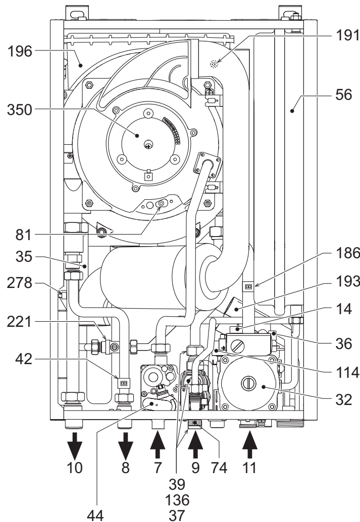
fig. 26 - Vista generale
