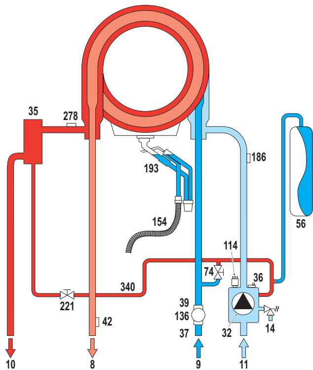
fig. 27 - Circuito idraulico
