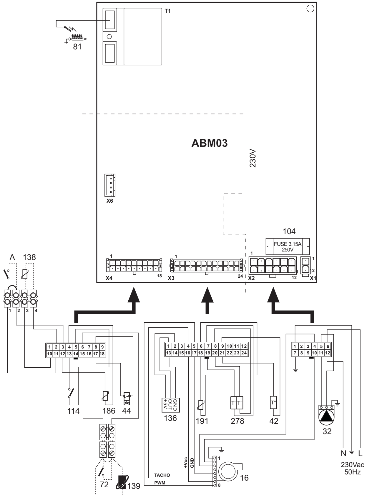
fig. 30 - Wiring diagram
