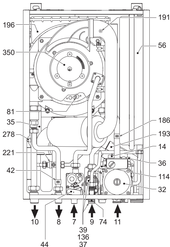
рис. 26 - Общий вид
