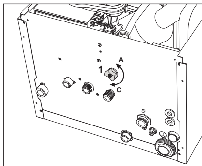
рис. 12 - Кран для заливки
