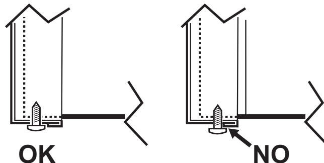
мал. 25 - Коректне положення передньої панелі
