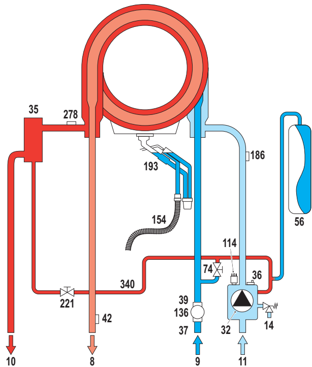
рис. 27 - Гидравлический контур
