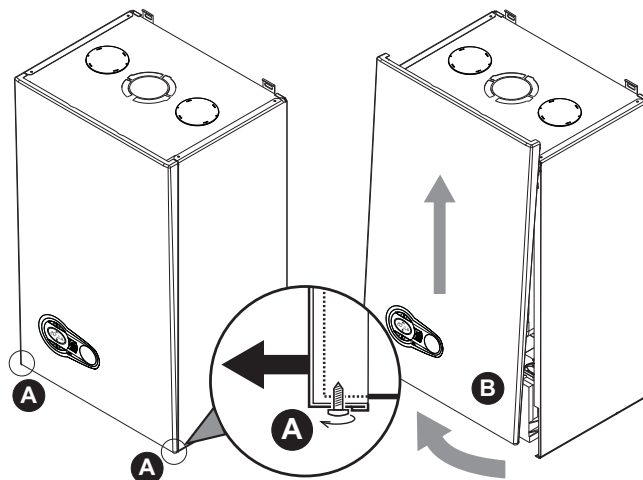
fig. 24 - Ouverture du panneau avant
