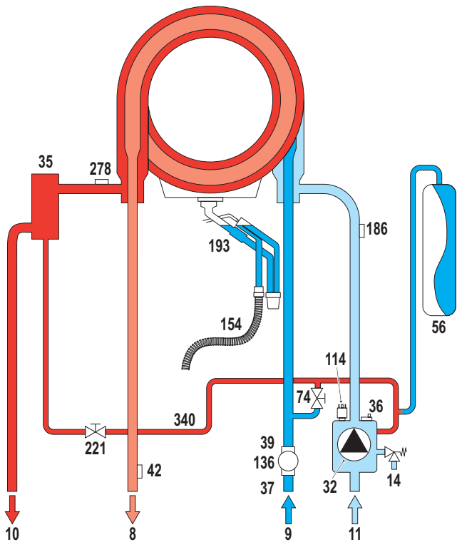
fig. 27 - Circuito hidráulico
