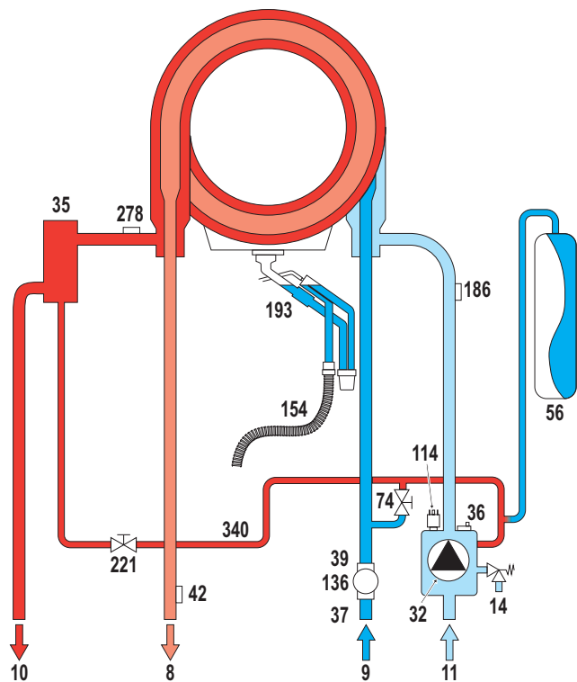
fig. 27 - Circuit hydraulique
