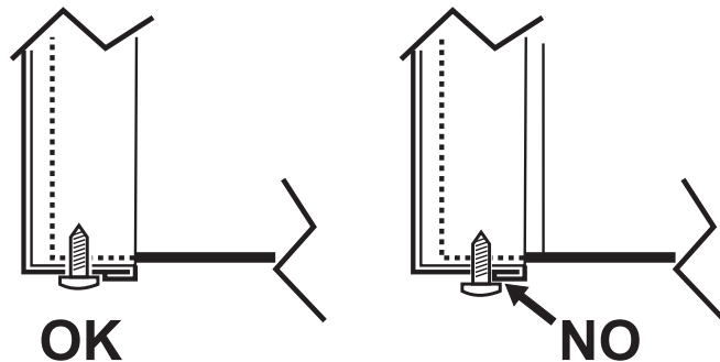
fig. 25 - Posición correcta del panel frontal
