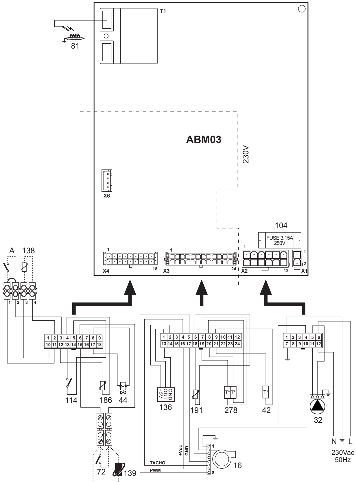
fig. 30 - Schemă electrică
