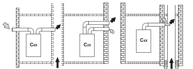
рис. 19 - Примеры подсоединения к дымоходам (⇐ = Воздух / ⇨ = Дымовые газы)
