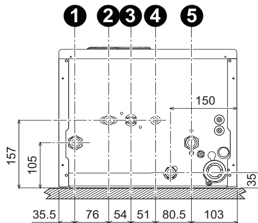
рис. 13 - Гидравлические штуцеры
