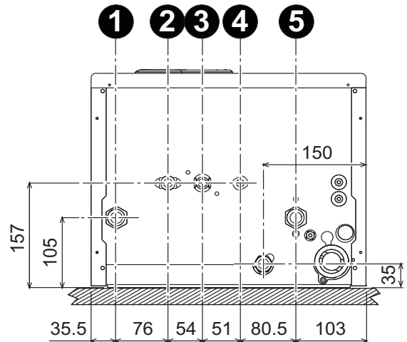
fig. 13 - Racorduri hidraulice
