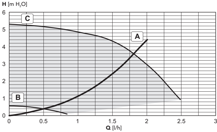
şek. 28 - Sirkülasyon yük / basınç kayıpları BLUEHELIX TECH 25 C
