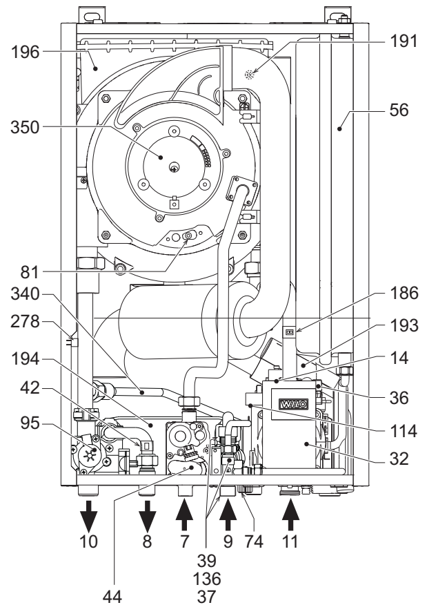
рис. 26 - Общий вид
