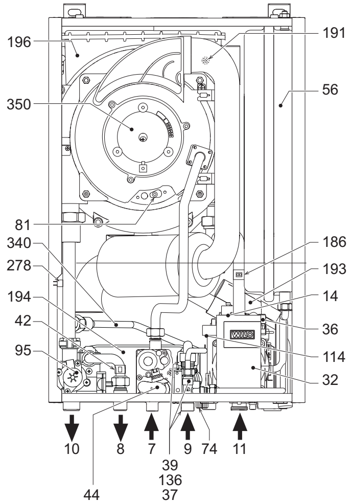
fig. 26 - Vista general
