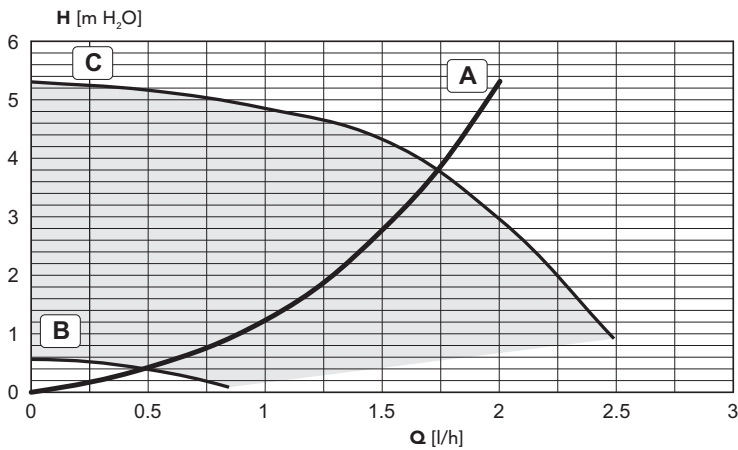
şek. 29 - Sirkülasyon yük / basınç kayıpları BLUEHELIX TECH 35 C
