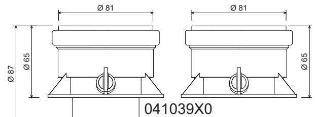
fig. 18 - Accessorio di partenza per condotti separati
