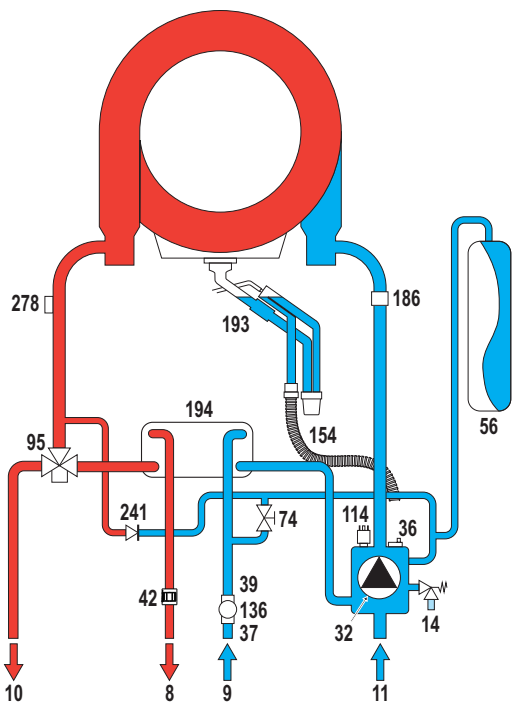
fig. 27 - Circuitul hidraulic
