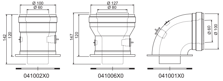
şek. 16 - Koaksiyal kanallar için çıkış aksesuarları
