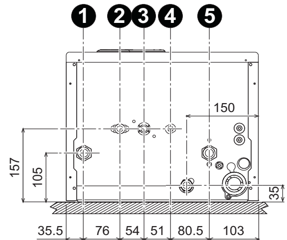
рис. 13 - Гидравлические штуцеры
