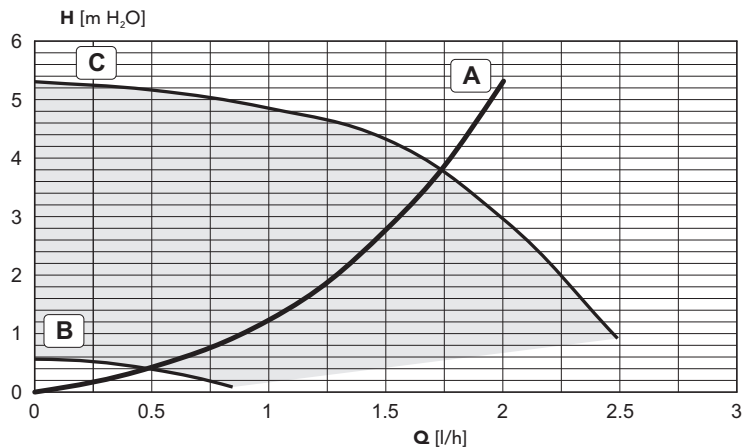
fig. 29 - Pierdere de sarcină / Înălțime de pompare pompă de circulație BLUEHELIX TECH 35 C
