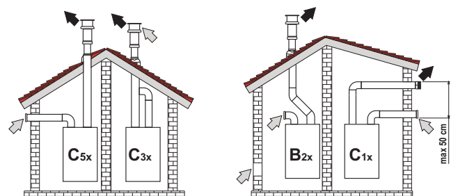
fig. 17 - Exemples de raccordements avec des conduits séparés (→ = Air / ← = Fumées)
