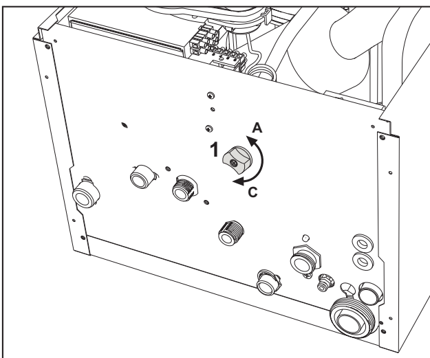
fig. 12 - Filling knob
