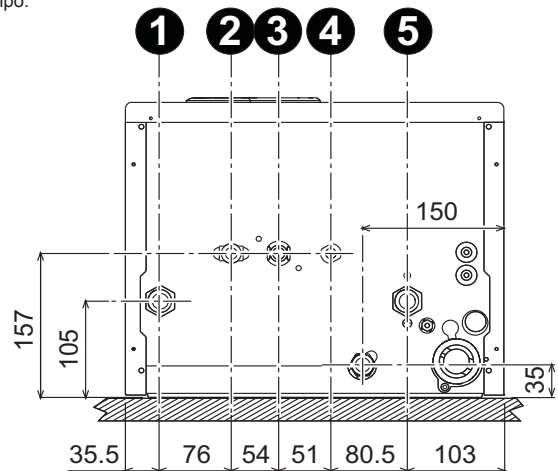
fig. 13 - Conexiones hidráulicas
