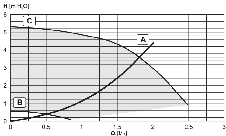
A = Pierderi de sarcină în centrală - B = Viteză minimă pompă de circulație - C = Viteză maximă pompă de circulație
