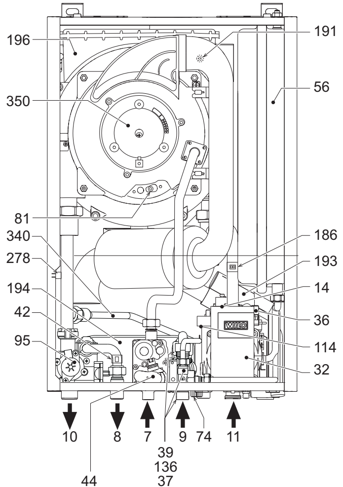
fig. 26 Vedere generală
