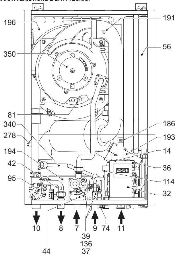
fig. 26 - Vista generale
