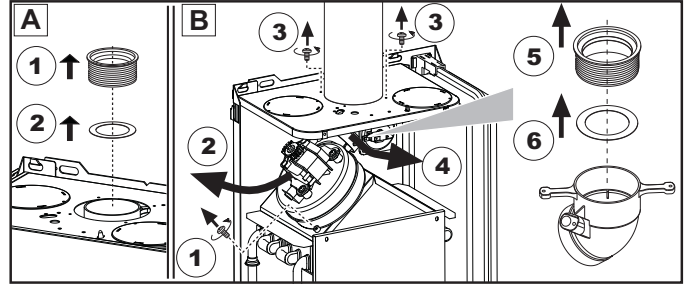
A Заміна діафрагми у ще не встановленому котлі
