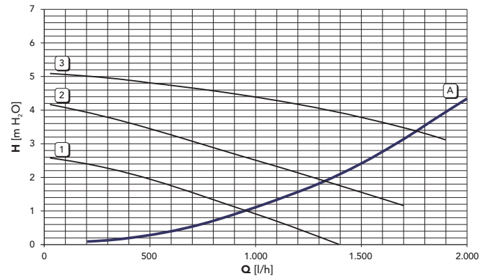
fig. 24 - Pertes de charge / pression circulatoires (DOMItech F 24 D)
