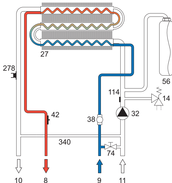
fig. 21 - Circuit hydraulique - sanitaire
