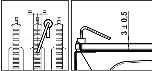
şek. 17 - Elektrot konumlandırma
