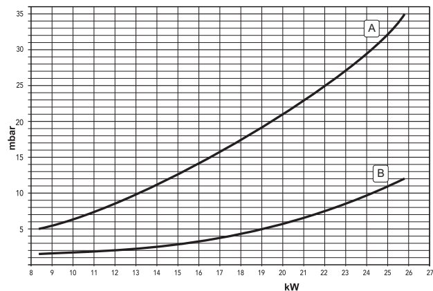
мал. 22 - Схема тиску - потужності (DOMItech F 24 D)
