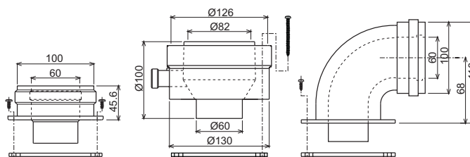
fig. 10 - Accesorios iniciales para conductos coaxiales
