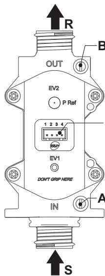
рис. 15 - Газовый клапан
