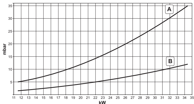
fig. 23 - Diagramă presiune - putere (DOMItech F 32 D)
