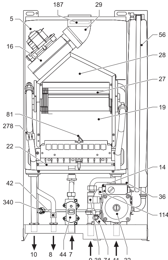
şek. 18 - Genel görünüm DOMItech F 24 D
