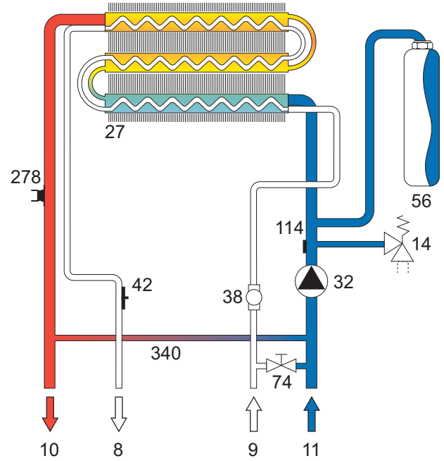
мал. 20 - Гідралічний контур системи опалення
