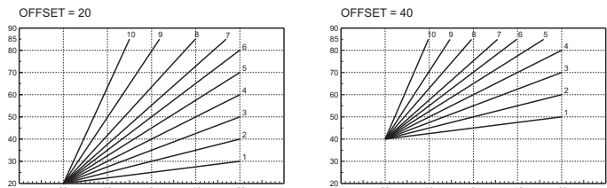
fig. 6 - Exemplu de deplasare paralelă a curbilor de compensare
