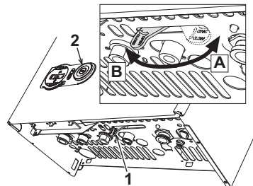
рис. 7 - Кран для подачи воды
