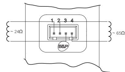
мал. 16 - Підключення газового клапану
