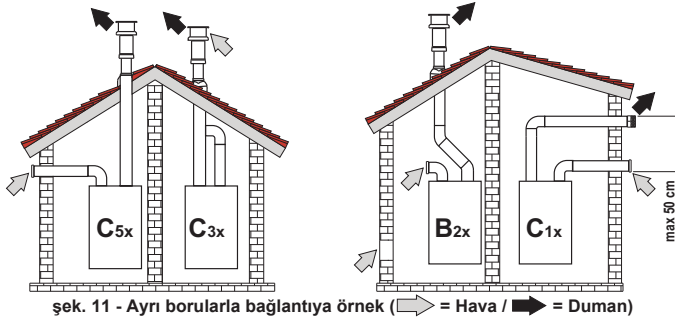
şek. 11 - Ayrı borularla bağlantıya örnek (⇐ = Hava / ⇨ = Duman)
