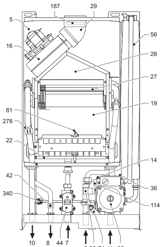
fig. 18 - Vue générale DOMItech F 24 D
