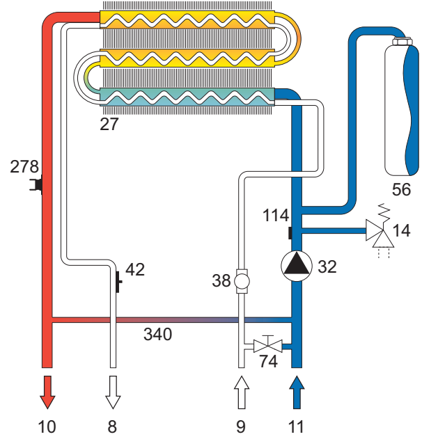
şek. 20 - Hidrolik devre Isıtma
