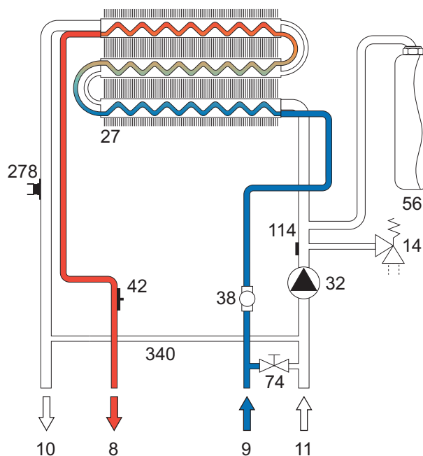
fig. 21 - Circuito idraulico Sanitario
