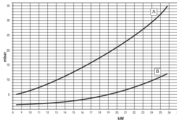
рис. 22 - Диаграммы давление - мощность (DOMItech F 24 D)
