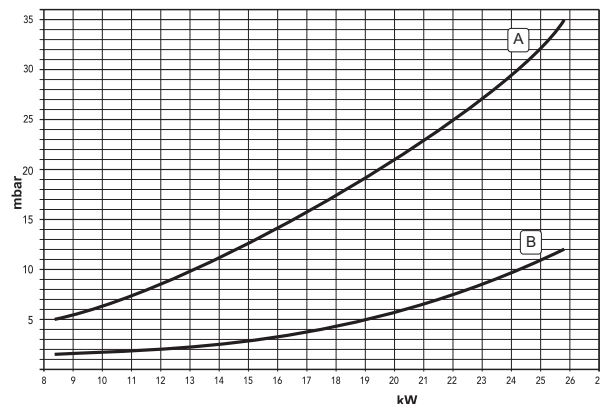
fig. 22 - Diagramă presiune - putere (DOMItech F 24 D)
