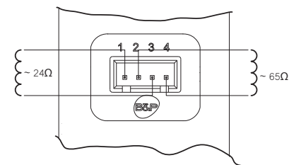
fig. 16 - Connexion soupape de gaz
