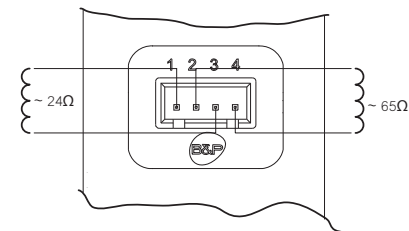
fig. 16 - Conexión de la válvula de gas
