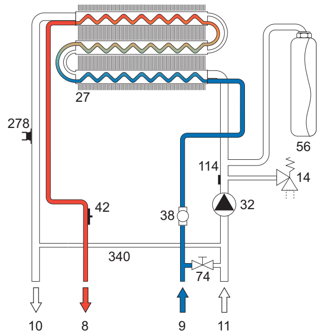
fig. 21 - Circuitul hidraulic Apă caldă menajeră
