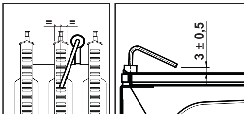
fig. 17 - Posizionamento elettrodo
