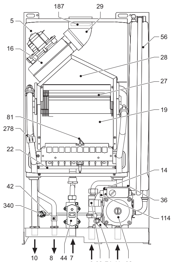
fig. 18 - Vista generale DOMItech F 24 D
