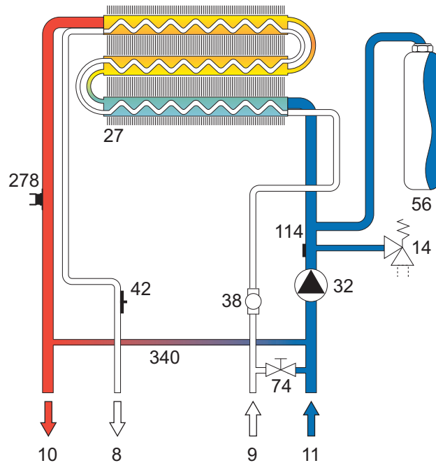
рис. 20 - Схема системы отопления
