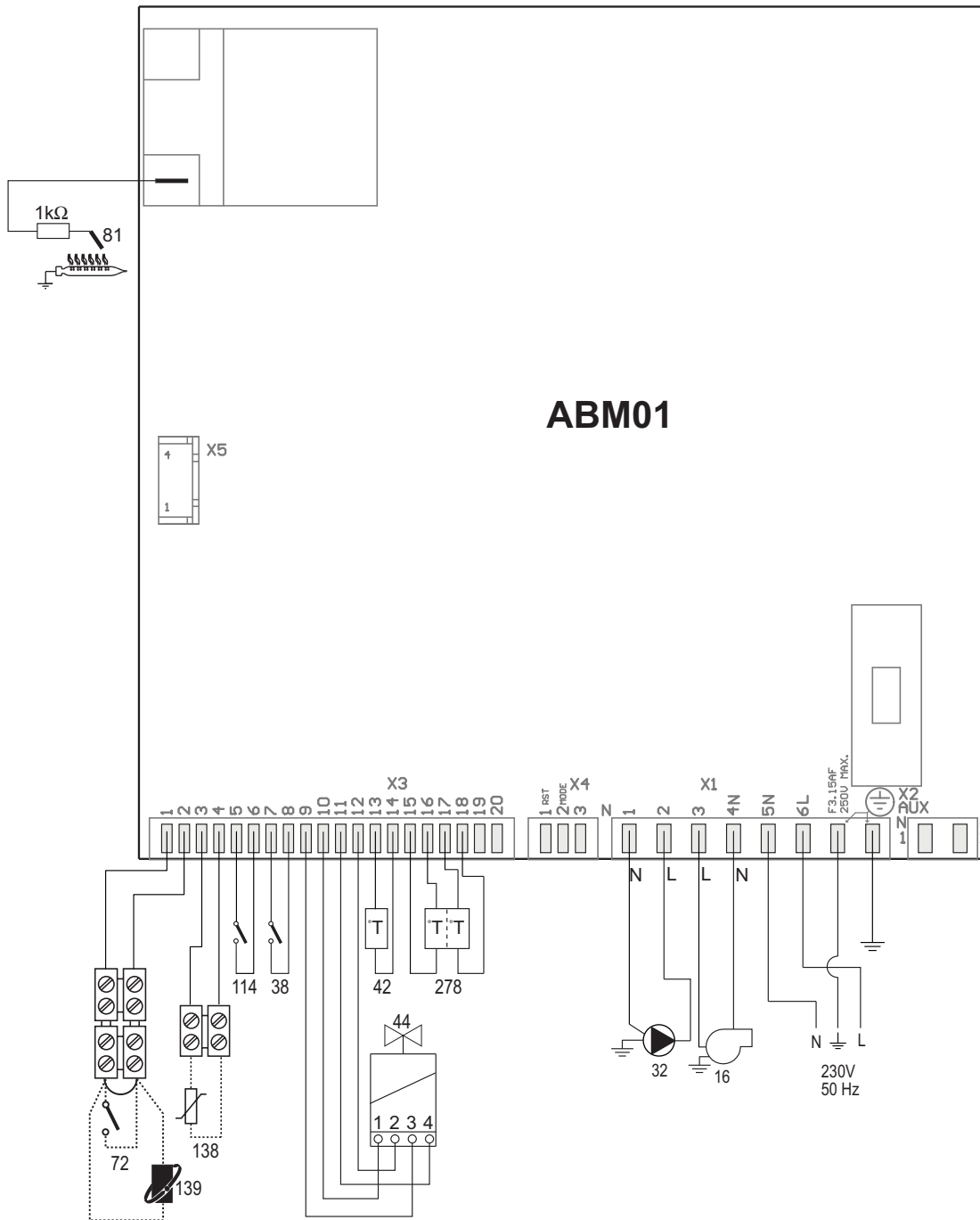
fig. 26 - Circuito elettrico
