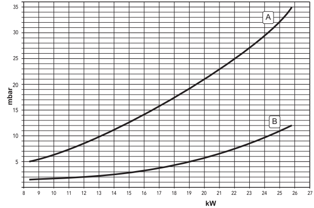
fig. 22 - Diagrama presión - potencia (DOMItech F 24 D)
