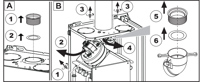
A Diyaframın kombi monte edilmemişken değiştirilmesi B Diyaframın kombi ve baca kanalları monte edildikten sonra değiştirilmesi
