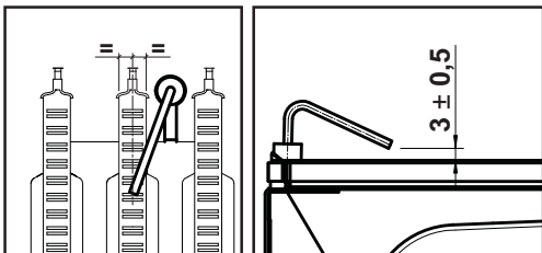
рис. 17 - Положение электрода
