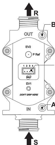
fig. 15 - Válvula del gas
