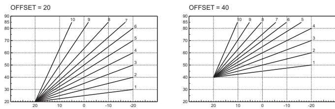
мал. 6 - Приклад паралельного пересування компенсаційних кривих
