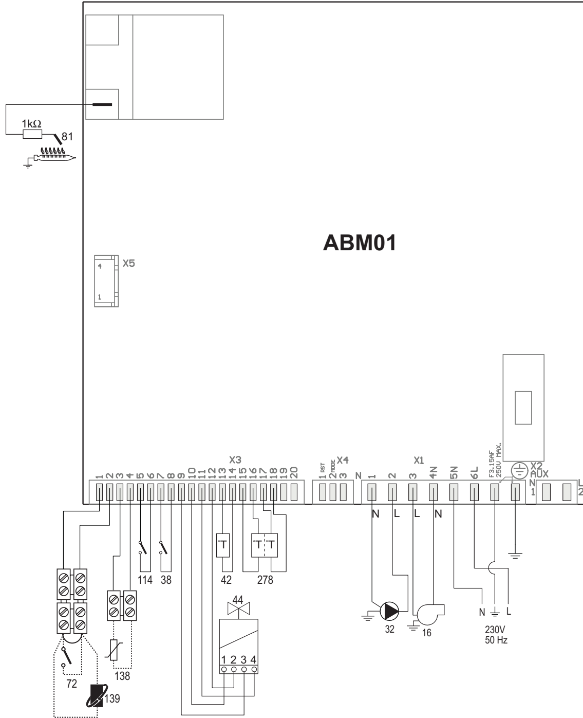
şek. 26 - Elektrik devresi
