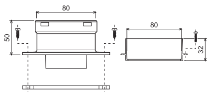
fig. 12 - Accesorio inicial para conductos separados
