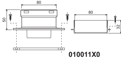
şek. 12 - Ayrı kanallar için çıkış aksesuarları
