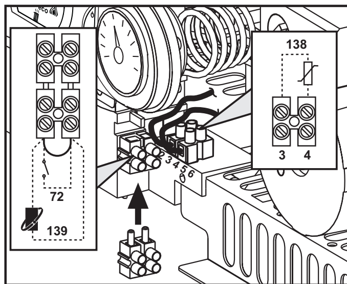
fig. 8 - Accès au bornier
