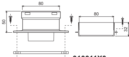
fig. 12 - Accessoire de départ pour conduits séparés
