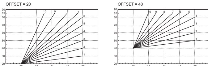
şek. 6 - Kompensasyon eğrilerinin paralel hareketi için örnek
