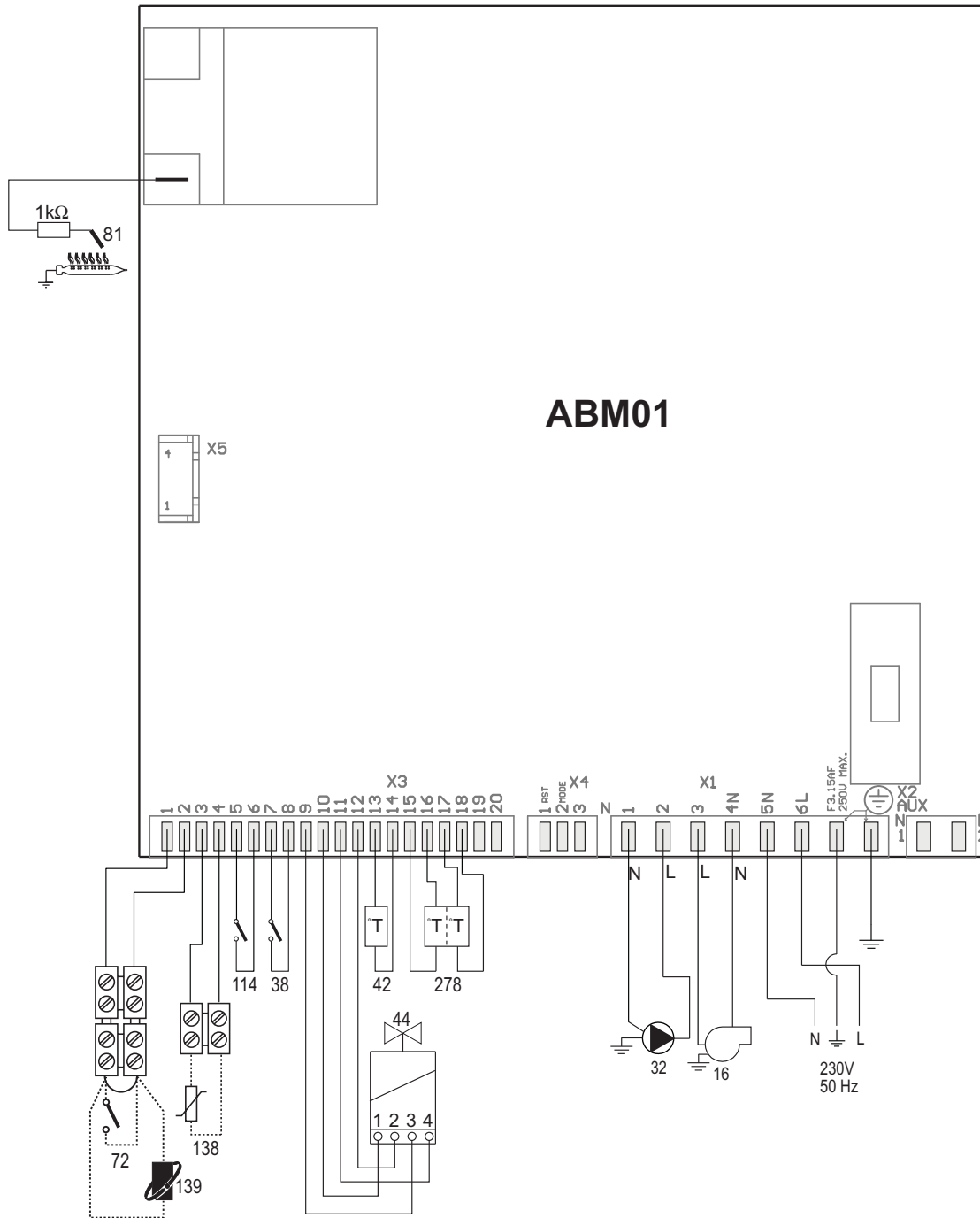
мал. 26 - Електричний контур
