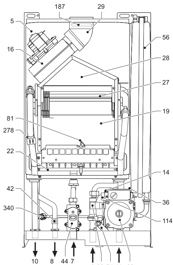
рис. 18 - Общий вид DOMItech F 24 D
