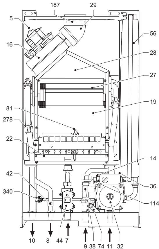
fig. 18 - Vedere generală DOMItech F 24 D
