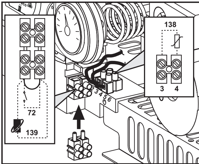
мал. 8 - Доступ до клемної коробки
