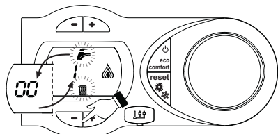
мал. 14 - Режим TEST (потужність опалення = 100%)
