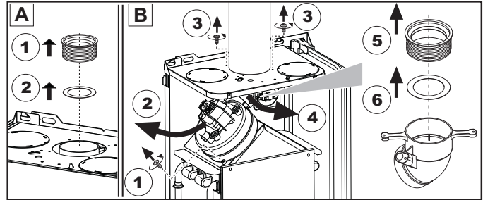
A Înlocuirea diafragmei cu centrala neinstalată
