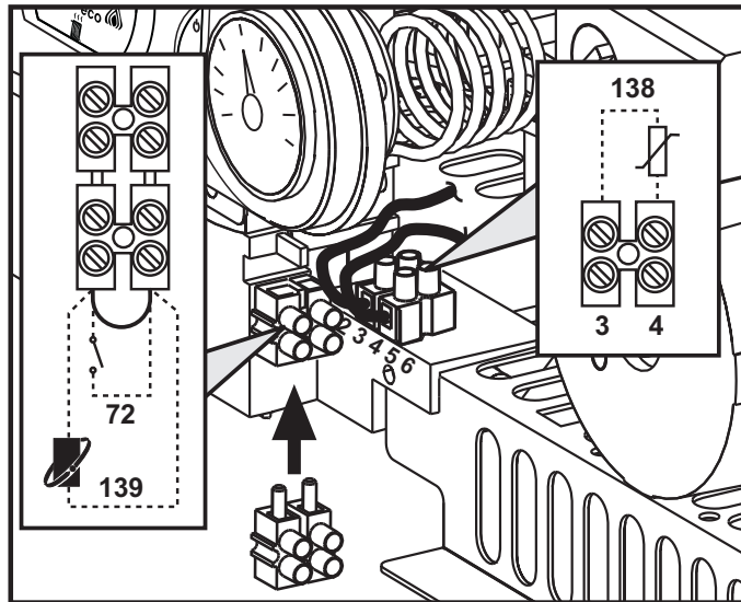
şek. 8 - Klemens kutusuna erişim
