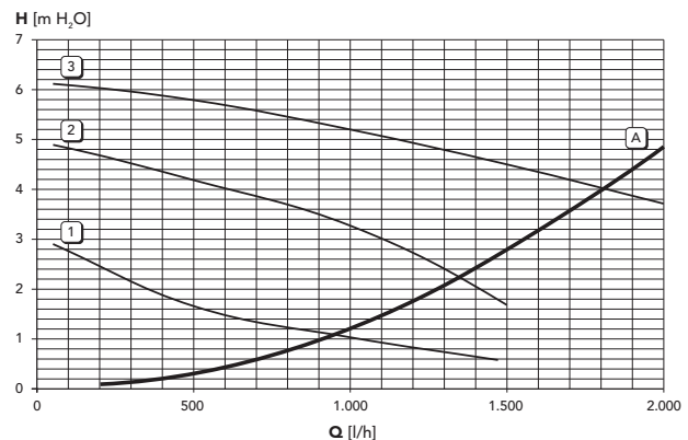
fig. 25 - Pertes de charge / pression circulatoires (DOMItech F 32 D)
