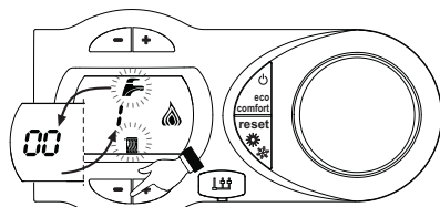
fig. 14 - Modul TEST (putere încălzire = 100%)
