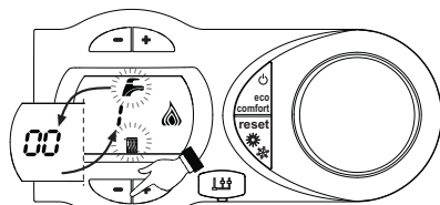
fig. 14 - Modalidad TEST (potencia de la calefacción = 100%)
