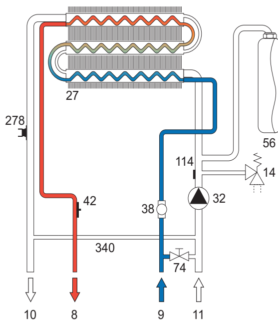
fig. 21 - Circuito hidráulico de AS
