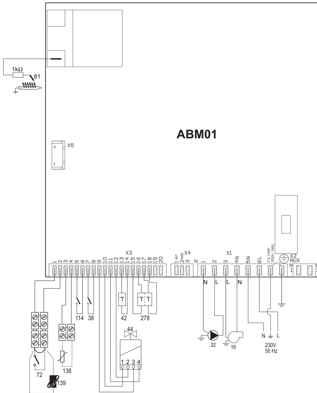
fig. 26 - Circuit électrique
