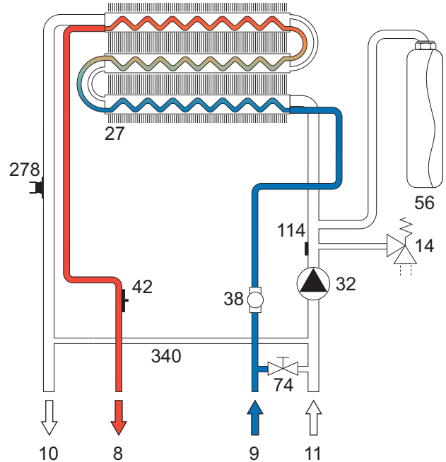
мал. 21 - Гідралічний контур ГВП
