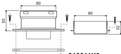
рис. 12 - Соединительный элемент для отдельных труб
