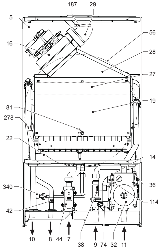
şek. 19 - DOMItech F 32 D
