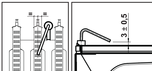
fig. 17 - Poziționarea electrodului
