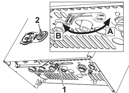
fig. 7 - Filling cock
