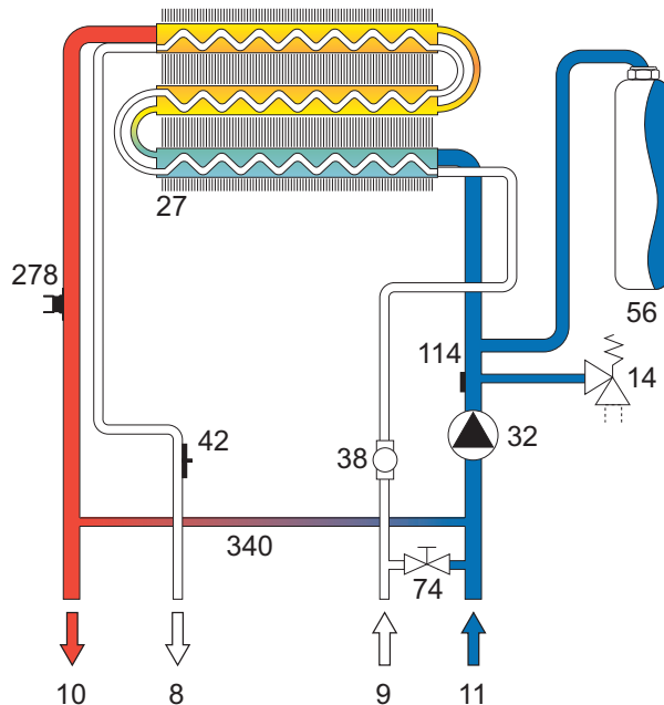
fig. 20 - Circuit hydraulique - chauffage
