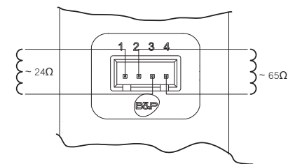
fig. 16 - Conexiune valvă gaz
