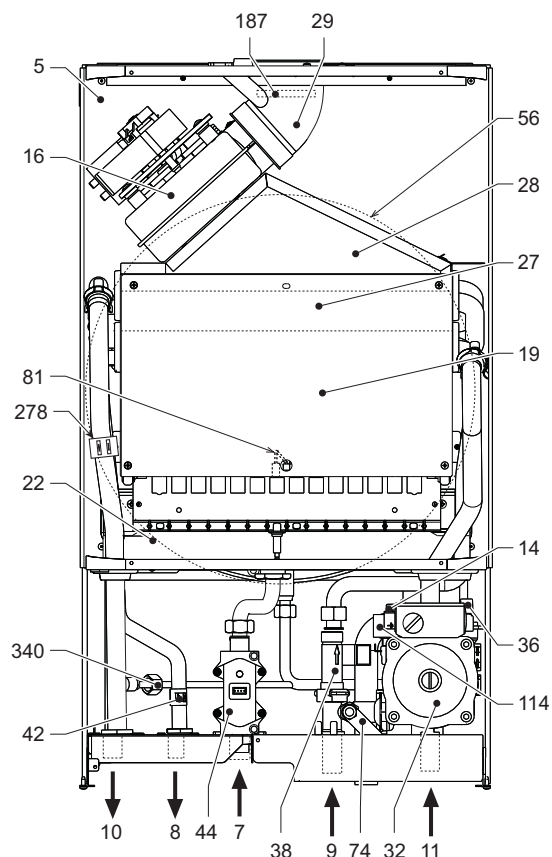
рис. 19 - DOMItech F 32 D
