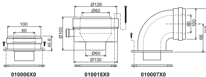
fig. 10 - Accessori di partenza per condotti coassiali
