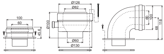
şek. 10 - Koaksiyal kanallar için çıkış aksesuarları
