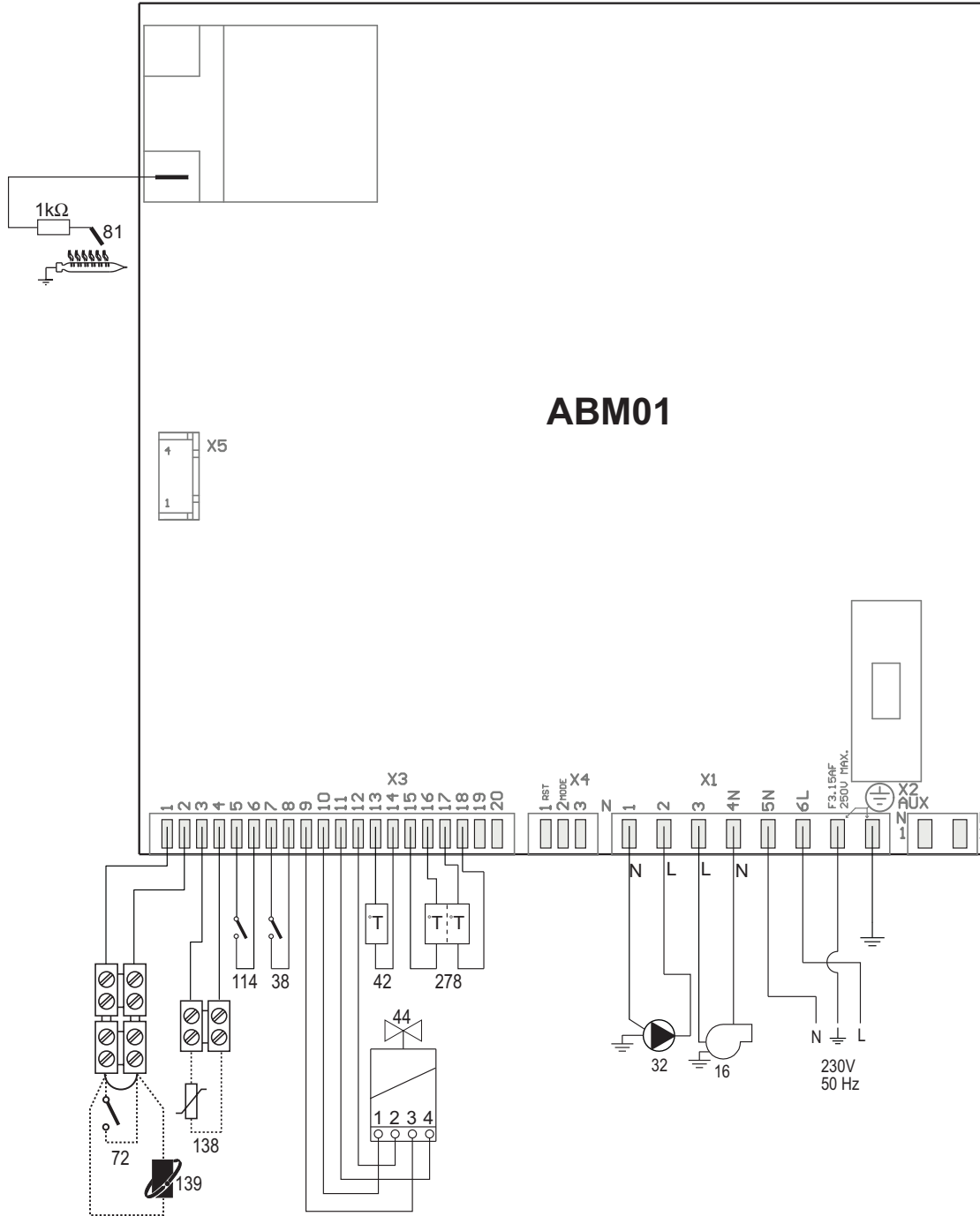
fig. 26 - Circuitul electric
