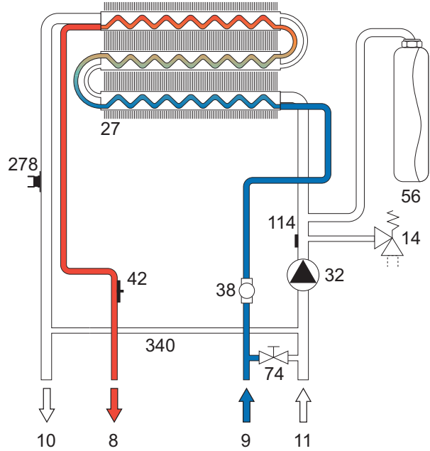
şek. 21 - Hidrolik devre Sıhhi Su
