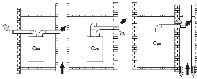
fig. 13 - Ejemplos de conexión a chimeneas (⇨ = aire / ⇨ = humos)
