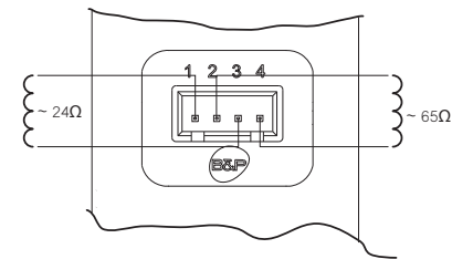
рис. 16 - Электрический разъем для подключения газового клапана
