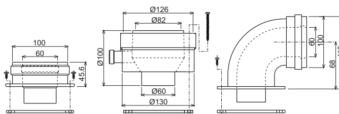
fig. 10 - Accessoires de départ pour conduits coaxiaux
