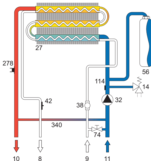
fig. 20 - Circuito hidráulico de calefacción
