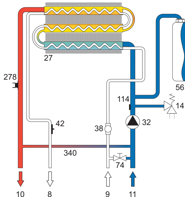
fig. 20 - Circuito idraulico Riscaldamento
