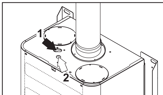
fig. 27 - Analisi fumi
