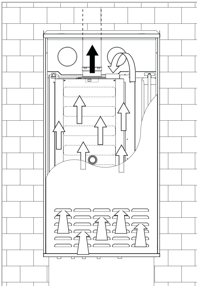
fig. 22 - Prelievo aria
