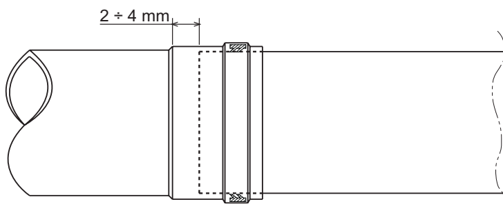
fig. 16 - Dilatazione
