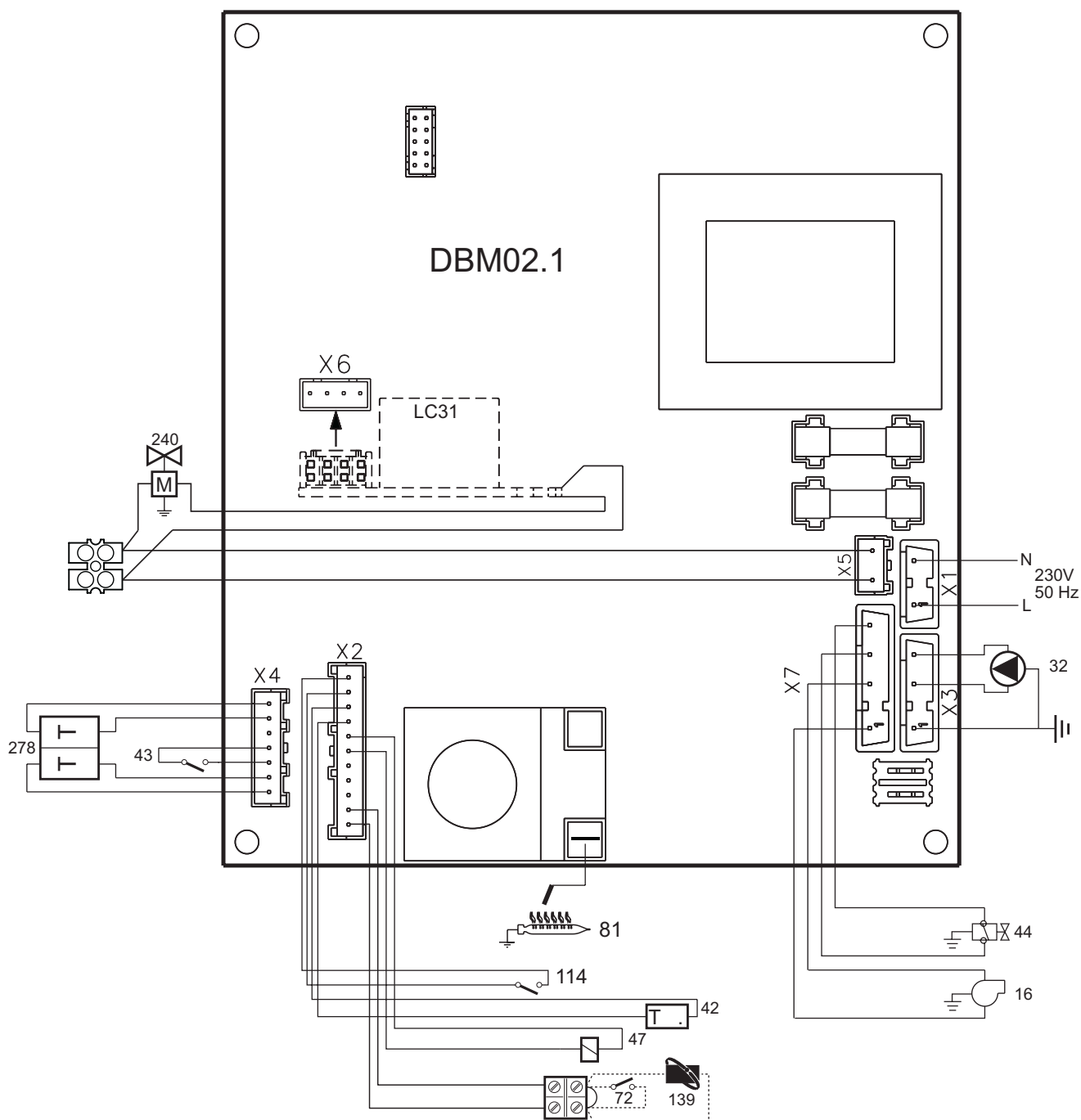
fig. 31 - Schema elettrico
