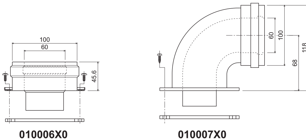
fig. 19 - Accessori di partenza per condotti coassiali
