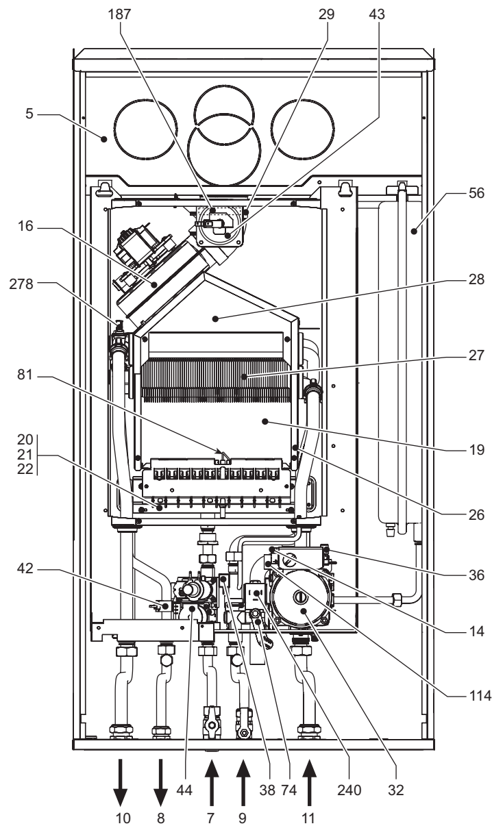
fig. 29 - Vista generale
