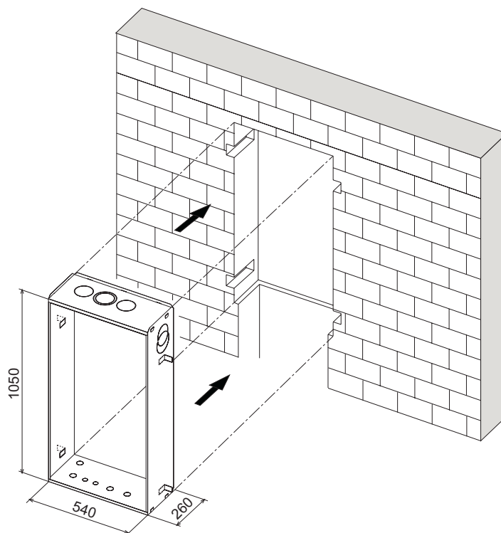
fig. 12 - Fissaggio dell'involucro alla parete
