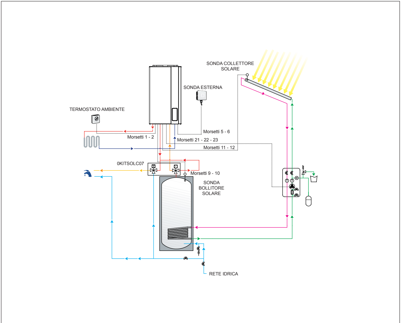
Fig. 13 Schema di collegamento impianto solare a circolazione forzata con caldaia combinata
