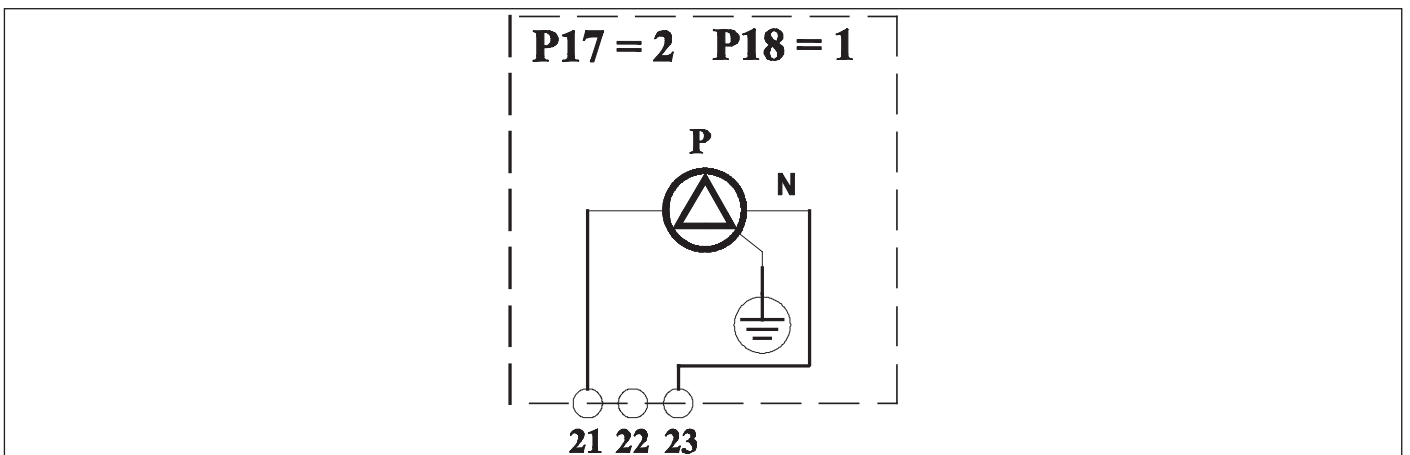
Fig. 14 Schema di collegamento relè multifunzione
