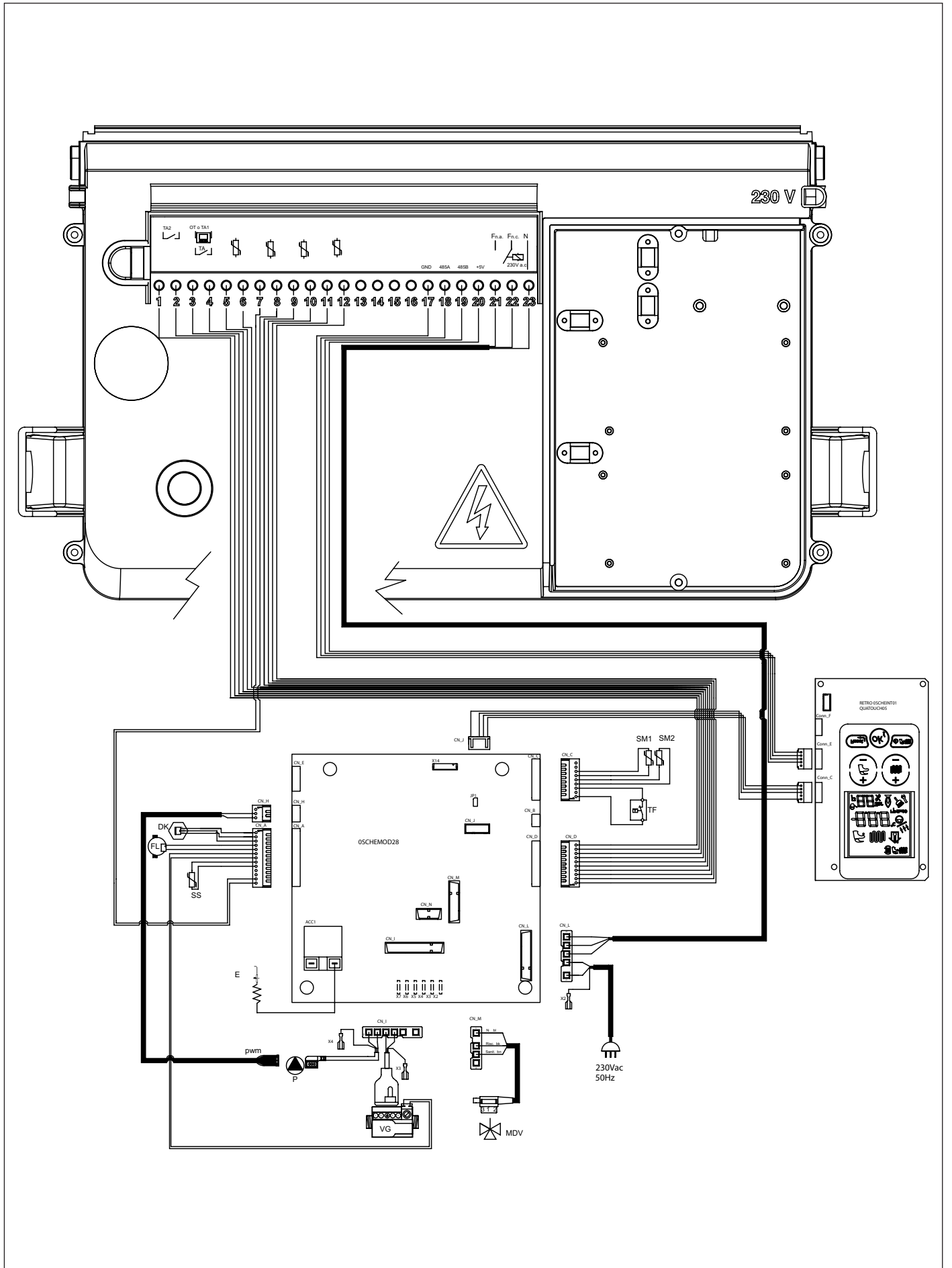
Fig. 12 Schema elettrico
