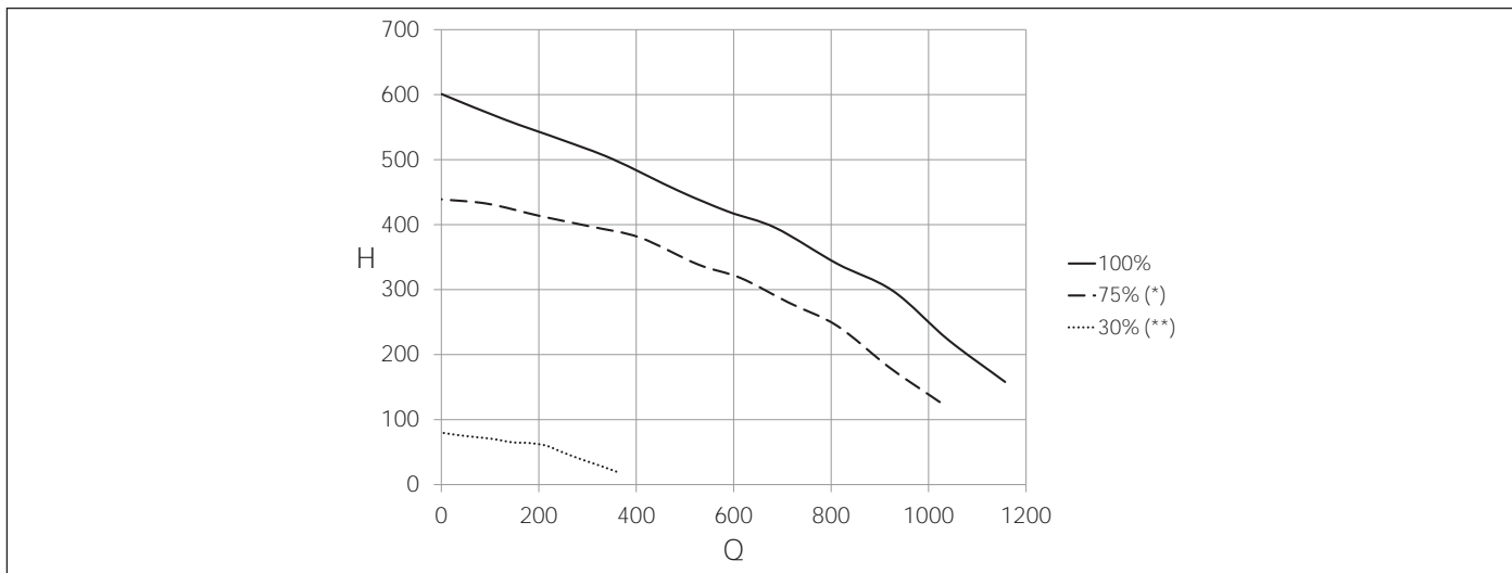
Fig. 20 Prevalenza disponibile KBS 24
