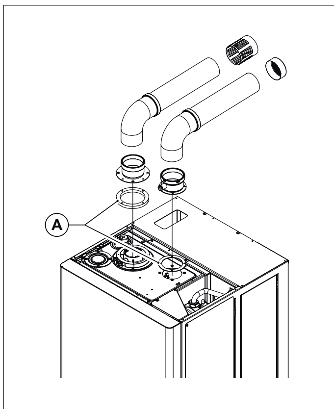
Fig. 12 Condotti coassiali tipo C43 - C53 - C83
