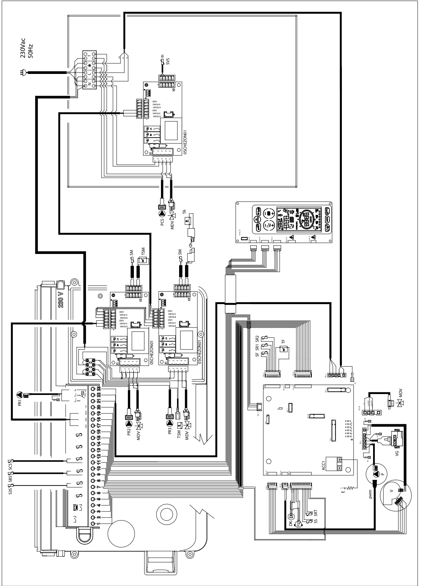
Fig. 28 Schema elettrico KRBS-Z
