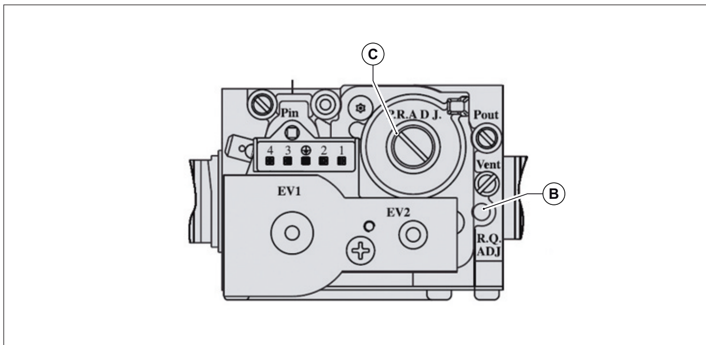
Fig. 33 Regolazione valore anidride carbonica
