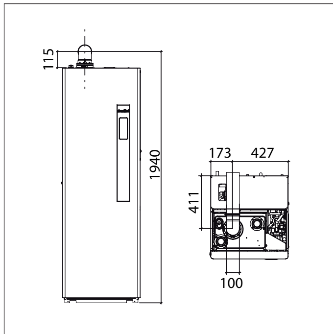
Fig. 11 Distanze condotti coassiali tipo C33
