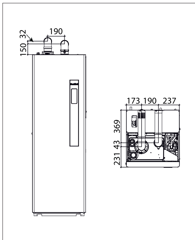
Fig. 13 Distanze condotti coassiali tipo C43 - C53 - C83
