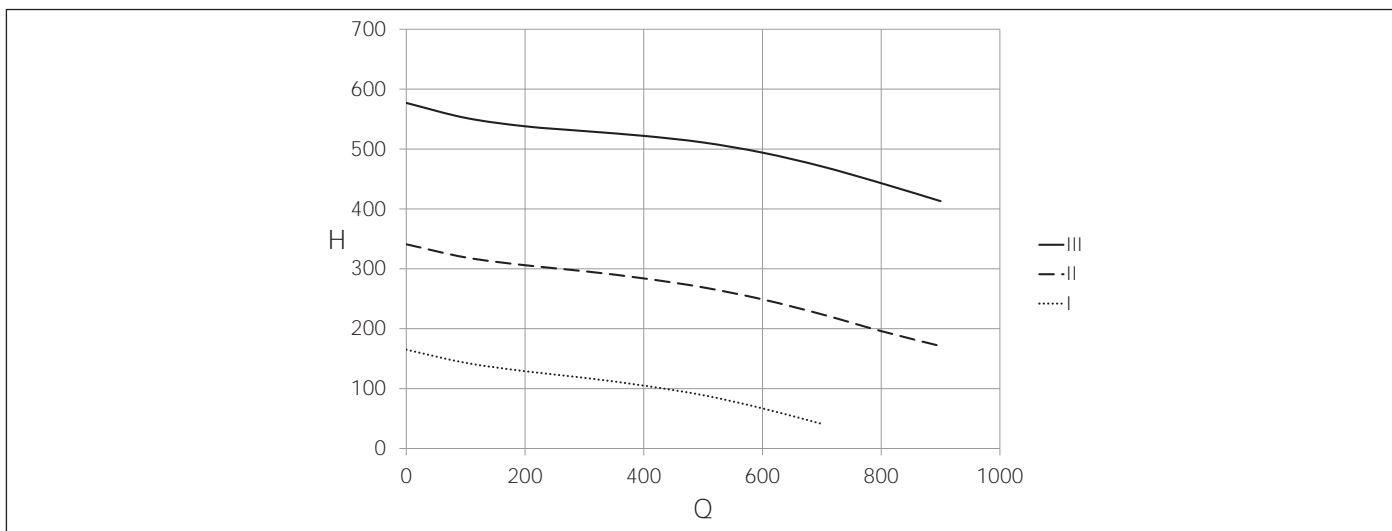
Fig. 22 Prevalenza disponibile circolatore solare
