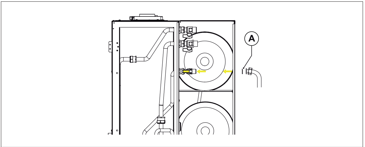
Fig. 16 Allacciamento alla rete del gas
