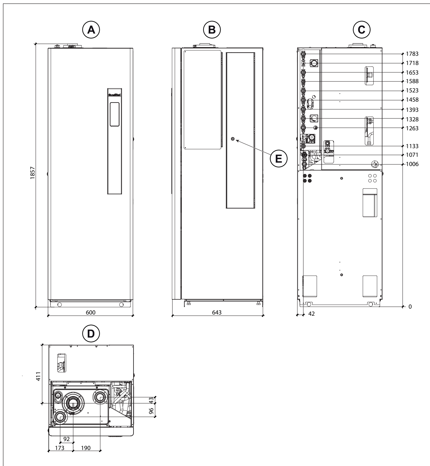
Fig. 4 Dimensioni
