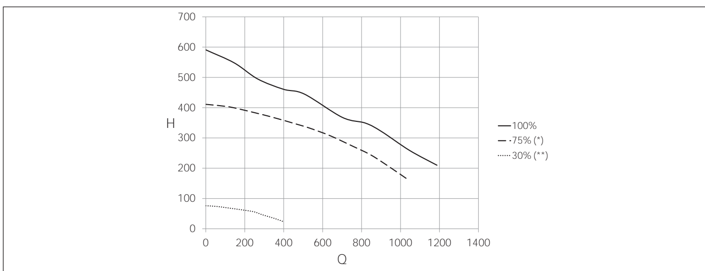
Fig. 21 Prevalenza disponibile KBS 32
