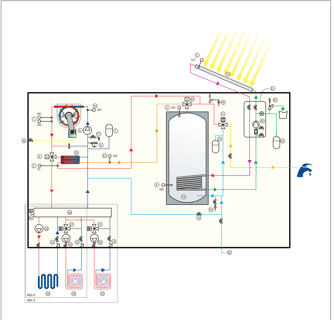
Fig. 9 Schema di funzionamento caldaia
