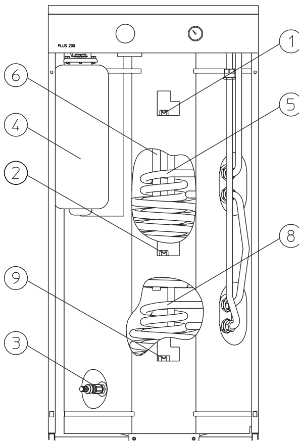
Unità bollitore 200 litri
