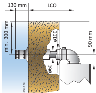
Esempio di sistema coassiale orizzontale (C 12 )
