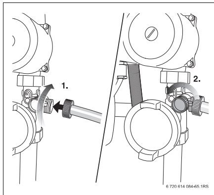
Fig. 4 Collegamento del tubo flessibile
