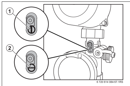
Fig. 10 Valvola di non ritorno
