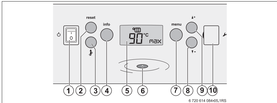
Fig. 1 Elementi di comando
