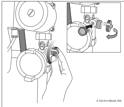
Fig. 3 Tappo di chiusura rubinetto di riempimento/scarico caldaia
