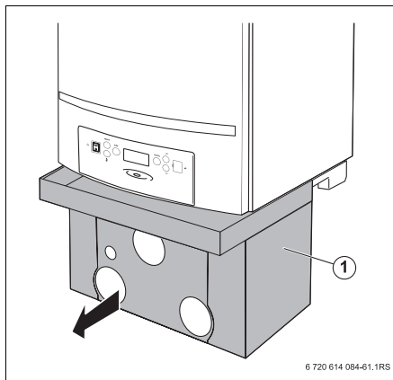
Fig. 2 Copertura del kit di collegamento idraulico (accessorio)
