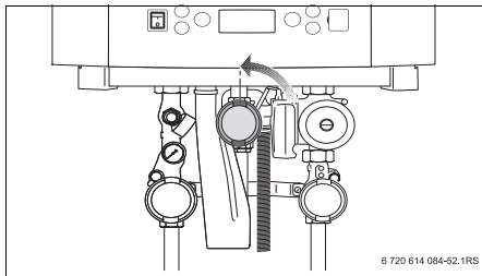
Fig. 9 Chiusura del rubinetto del gas
