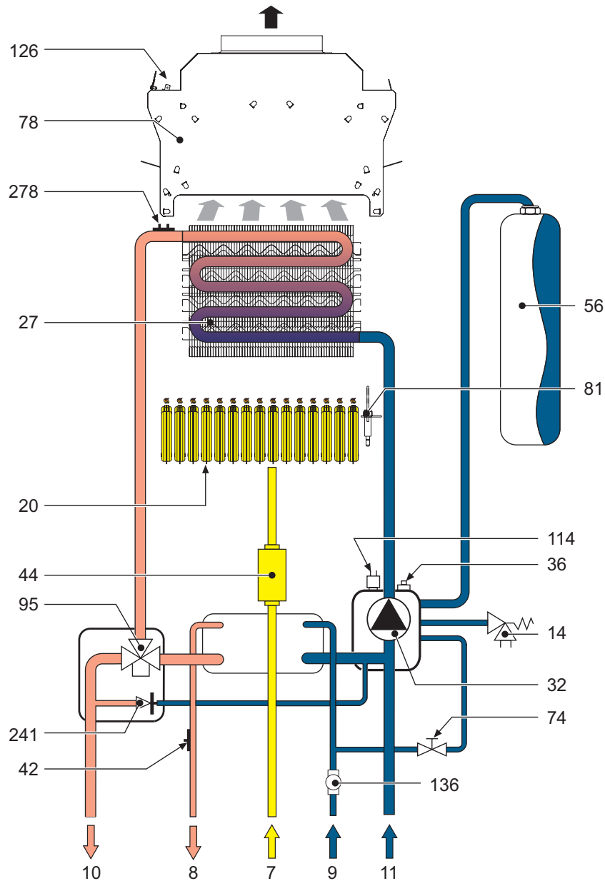
fig. 26 - Circuito hidráulico
