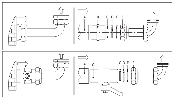
fig. 18 - Kit de ligação
