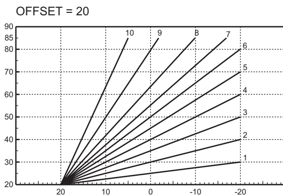
fig. 15 - Exemplo de deslocação paralela das curvas de compensação
