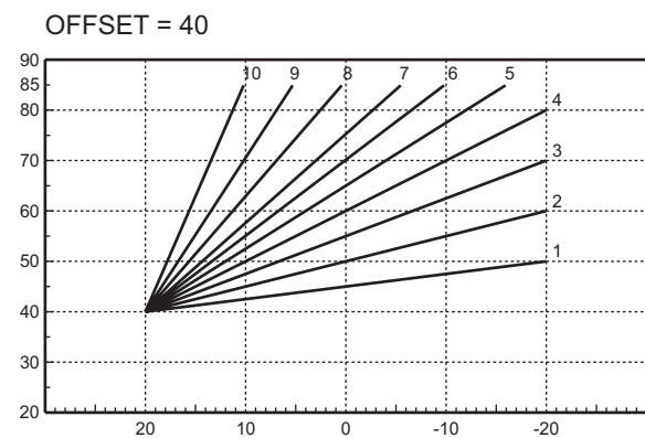
fig. 15 - Exemple de déplacement parallèle des courbes de compensation
