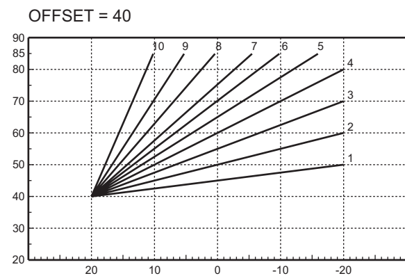
fig. 15 - Exemplo de deslocação paralela das curvas de compensação
