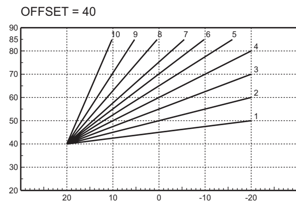
εικ. 15 - Παράδειγμα παράλληλης μετακίνησης των καμπυλών αντιστάθμισης
