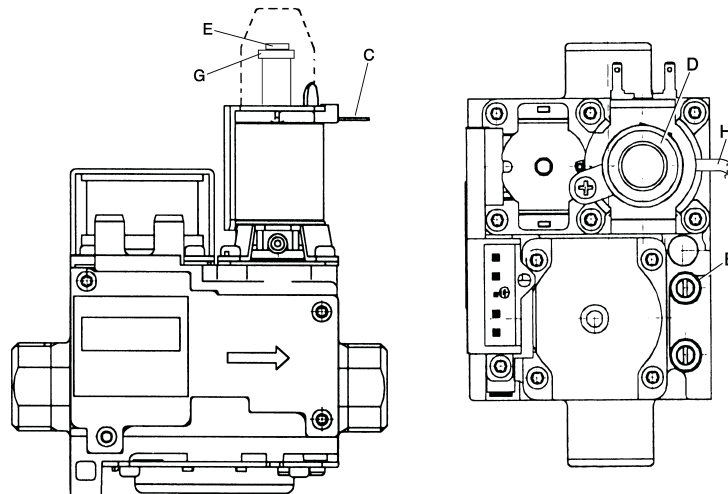
fig. 22 - Válvula de gas
