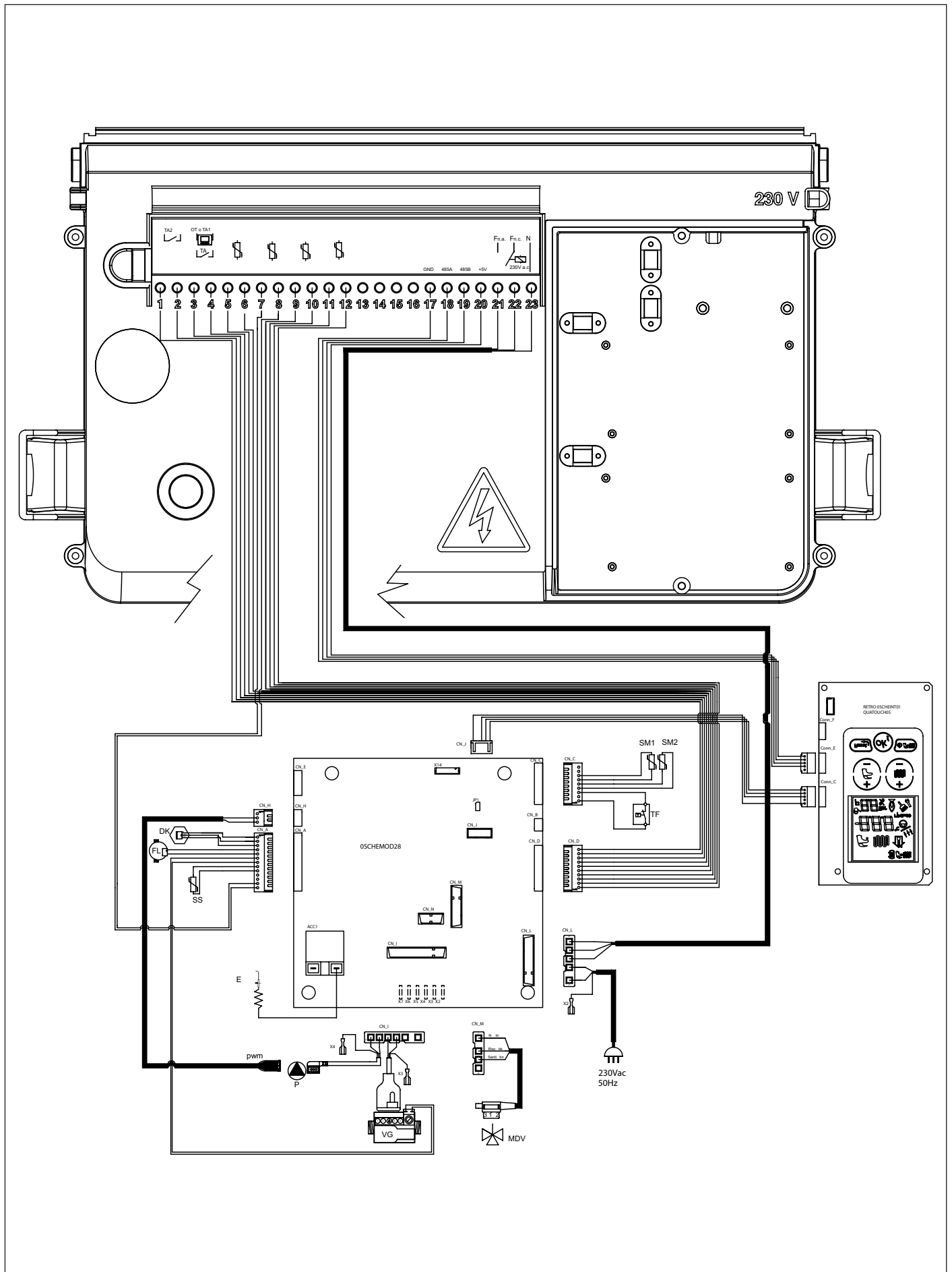
Fig. 12 Schema elettrico
