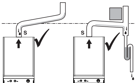
Scarico condensa Scarico valvola sicurezza
