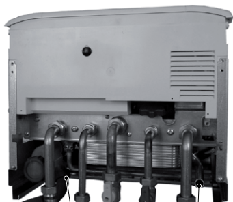
Scarico condensa Scarico valvola sicurezza
