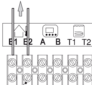
Morsetteria collegamento sonda esterna Fig. 5.45
