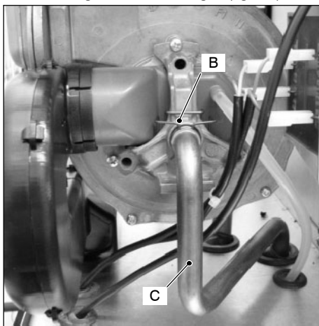
fig. 8.2 (vista dalla parte destra del ventilatore)
