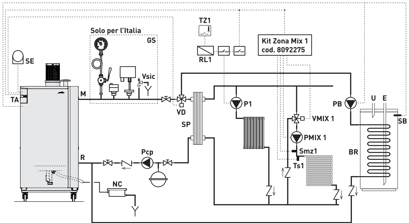
Schema idraulico con bollitore prima dello scambiatore a piastre
