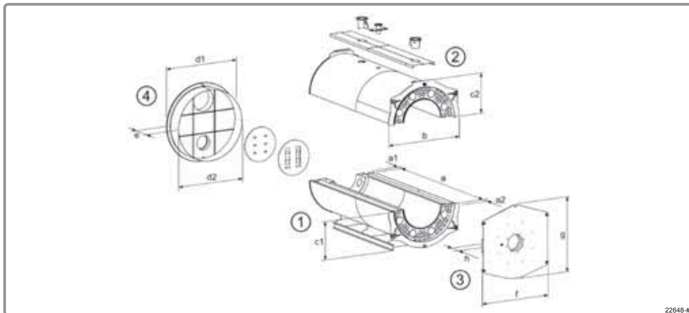
figura 19 - Dimensioni versione sezionata
