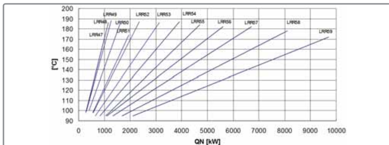
figura 12 - Temperatura dei fumi LRR, low-NOx, metano e ARF con caldaia pulita
