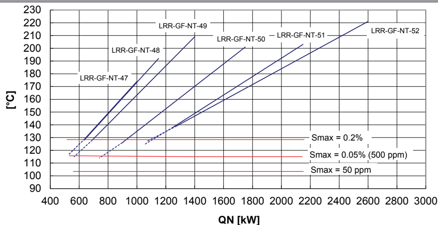
figura 22 - Temperatura dei fumi LRR-GF-NT, low-NOx, gasolio con caldaia pulita
