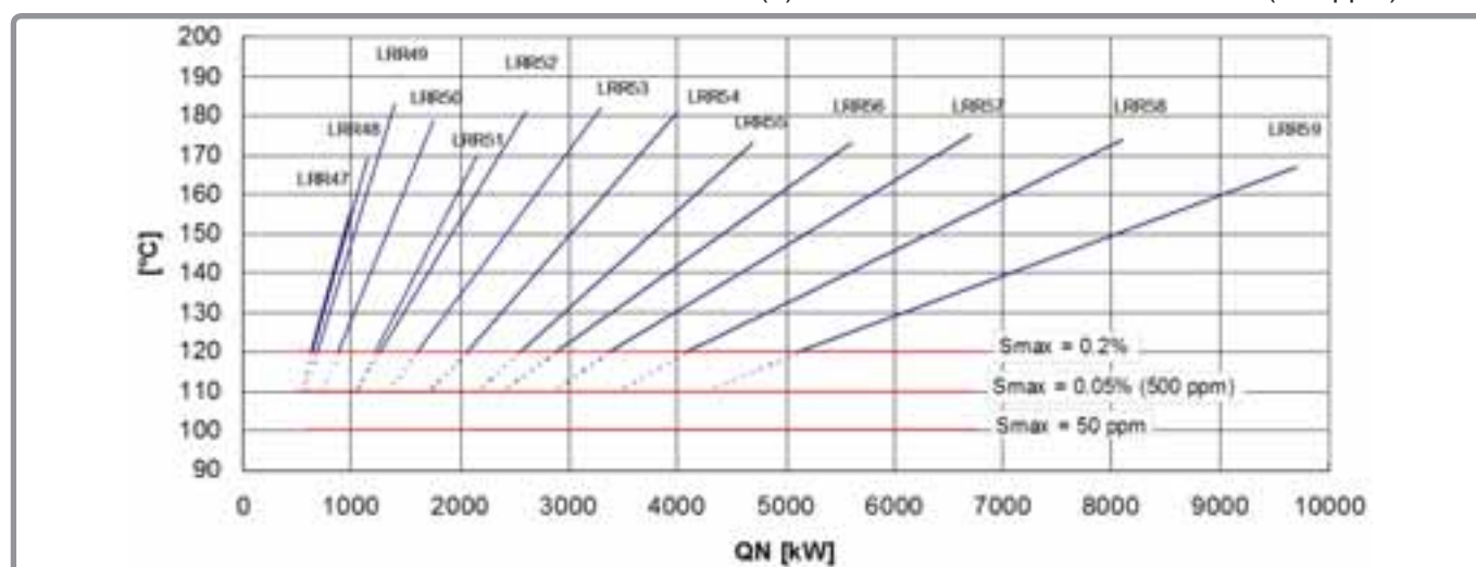
figura 9 - Temperatura dei fumi LRR, low-NOx, gasolio con caldaia pulita
