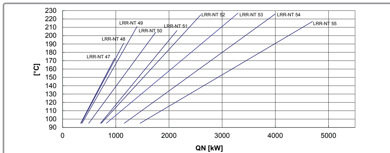
figura 16 - Temperatura dei fumi LRR-NT, low-NOx, metano con caldaia pulita
