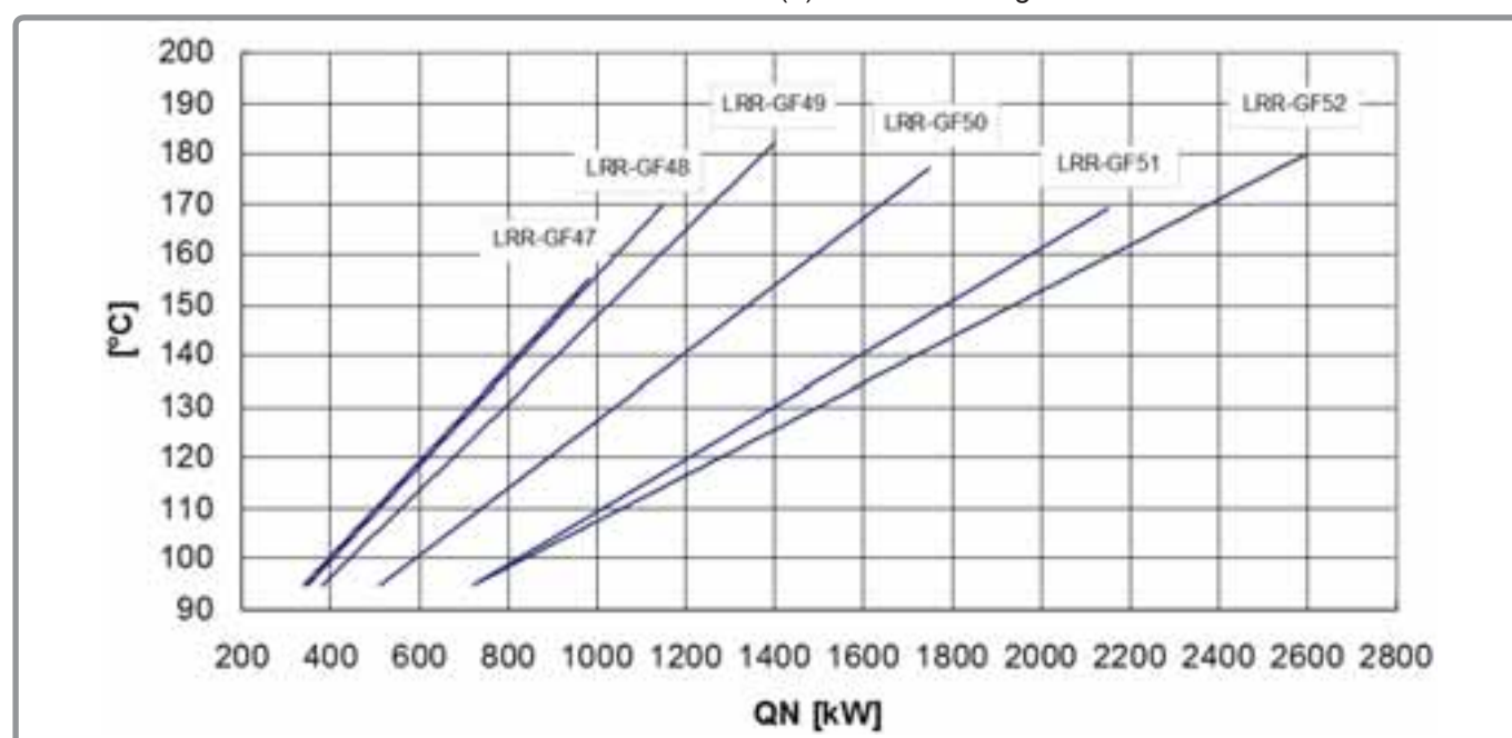
figura 21 - Temperatura dei fumi LRR-GF, low-NOx, metano con caldaia pulita
