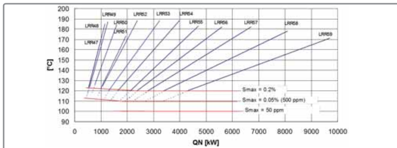
figura 11 - Temperatura dei fumi LRR, low-NOx, gasolio e ARF con caldaia pulita
