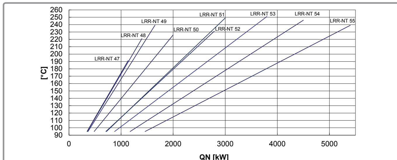
figura 14 - Temperatura dei fumi LRR-NT, metano con caldaia pulita
