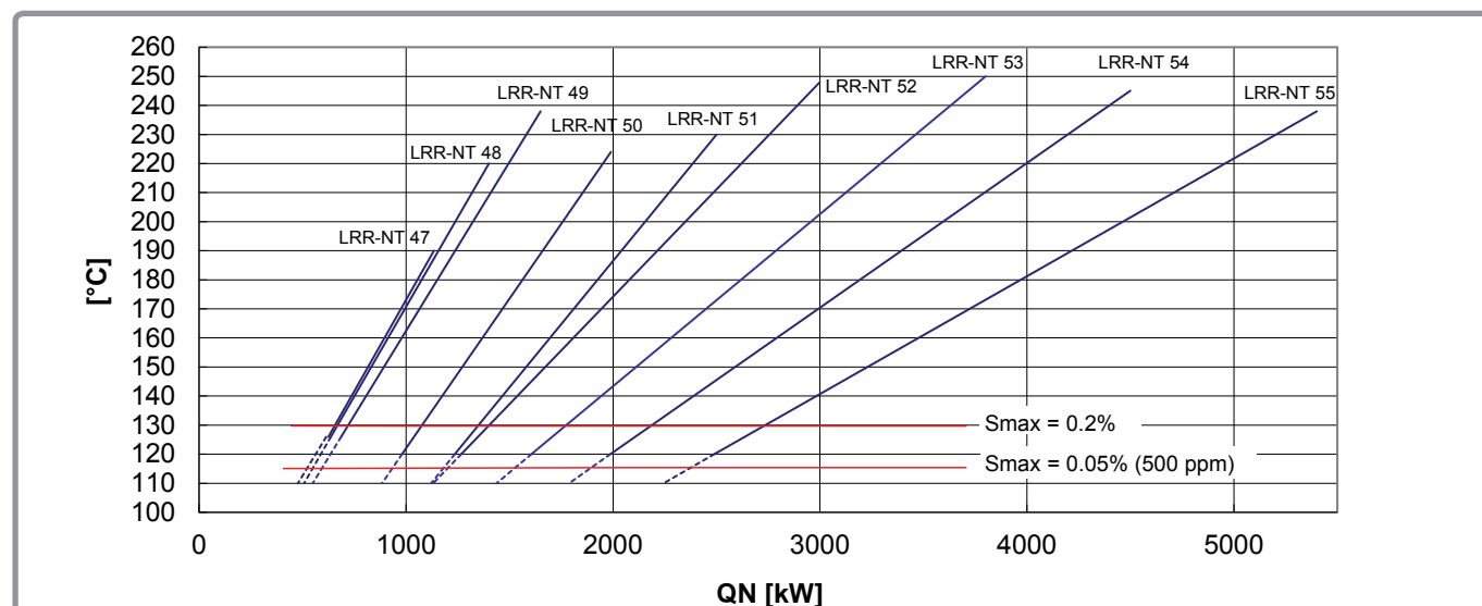
figura 13 - Temperatura dei fumi LRR-NT, gasolio con caldaia pulita
