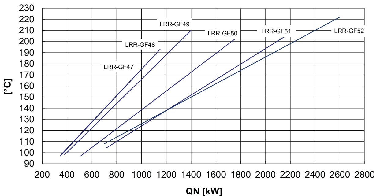
figura 23 - Temperatura dei fumi LRR-GF-NT, low-NOx, metano con caldaia pulita
