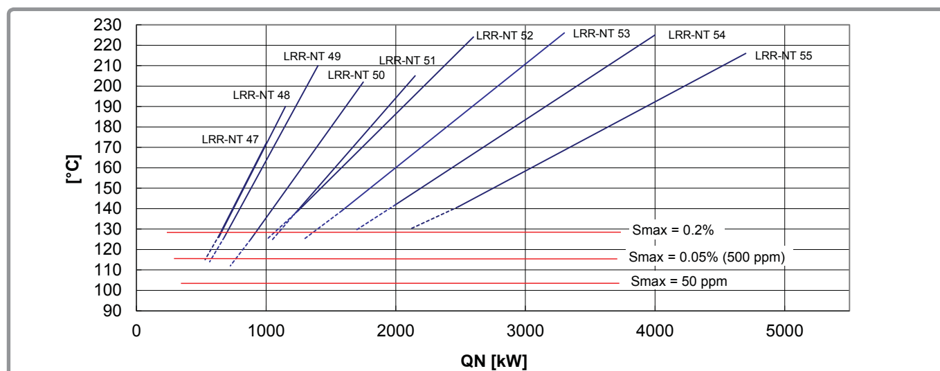
figura 15 - Temperatura dei fumi LRR-NT, low-NOx, gasolio con caldaia pulita
