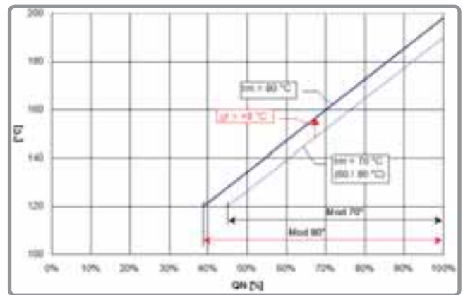
figura 24 - Temperatura Fumi – Potenza (esempio per due temperature medie dell'acqua caldaia)
