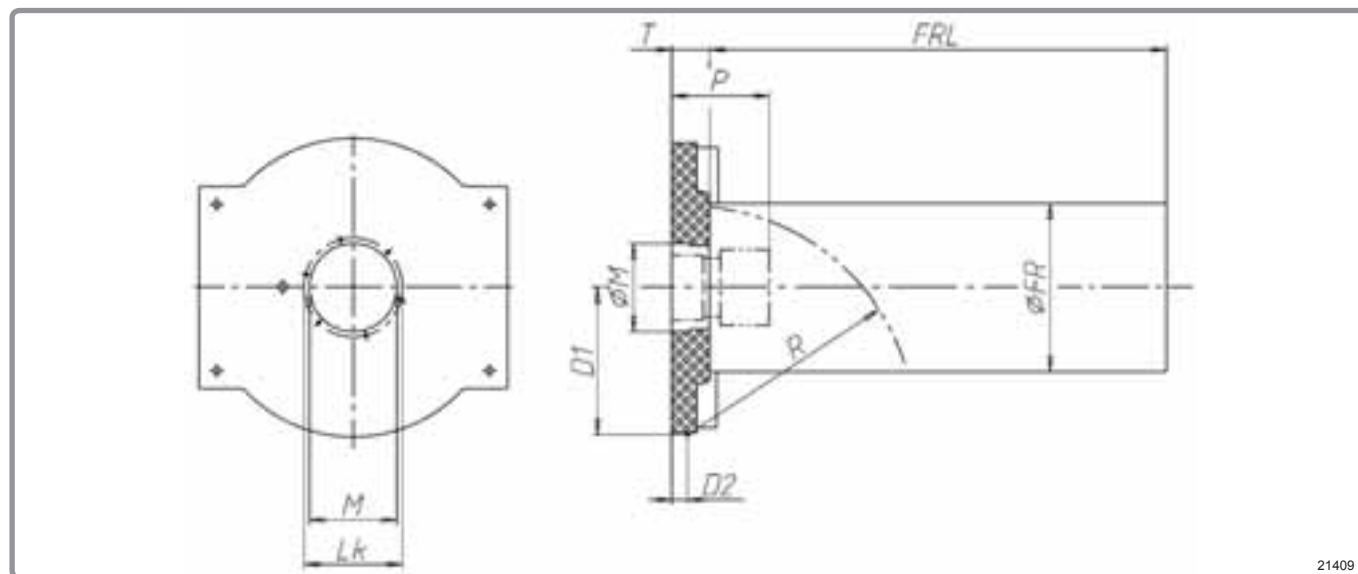
figura 30 - Quote di accoppiamento LRR-GF / LRR-GF-NT
