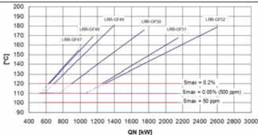
figura 20 - Temperatura dei fumi LRR-GF, low-NOx, gasolio con caldaia pulita
