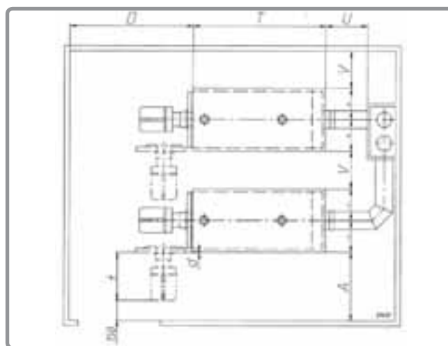
figura 25 - Distanze di installazione
