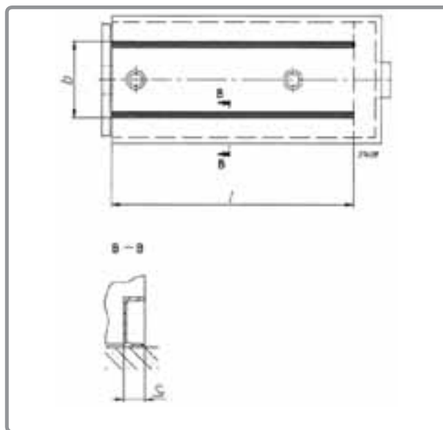
figura 27 - Senza antivibranti
