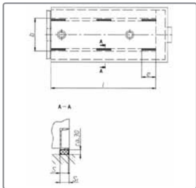
figura 26 - Con antivibranti
