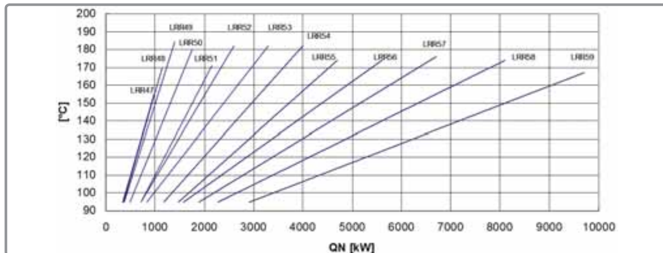
figura 10 - Temperatura dei fumi LRR, low-NOx, metano con caldaia pulita
