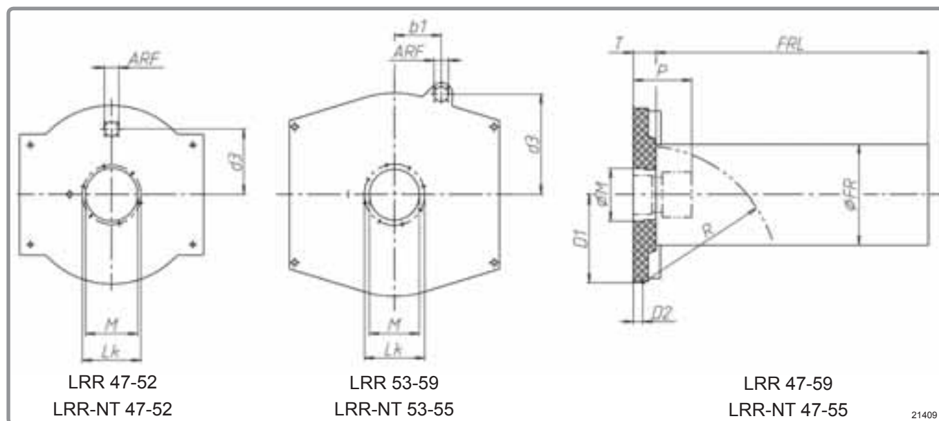
figura 29 - Quote di accoppiamento LRR / LRR-NT
