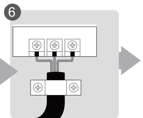
6 Conecte el cableado (no aplicable a algunos lugares en Norteamérica)
