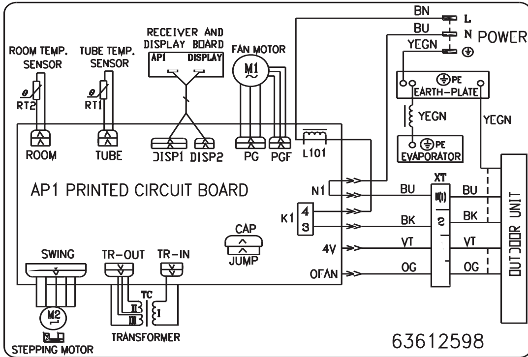
Cablaggi unità interna ON/OFF 5300 W / 5300 W ON/OFF Indoor unit wiring diagram
