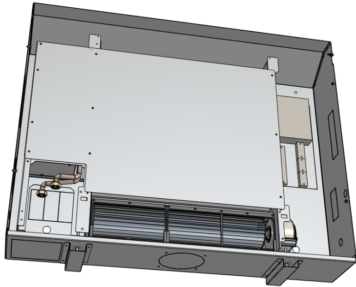
Montaggio a parete unità con mobiletto
