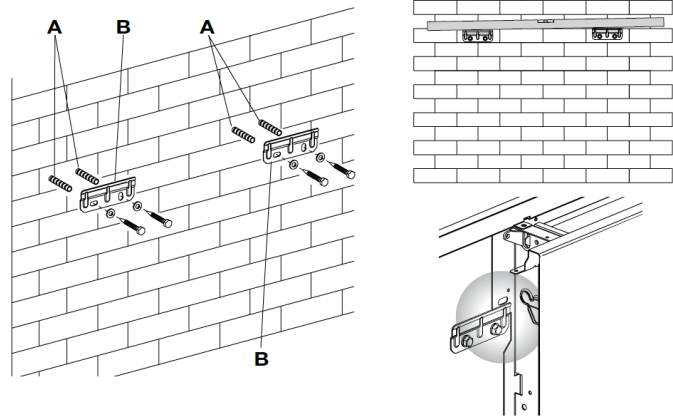
Montaggio a parete unità con mobiletto
