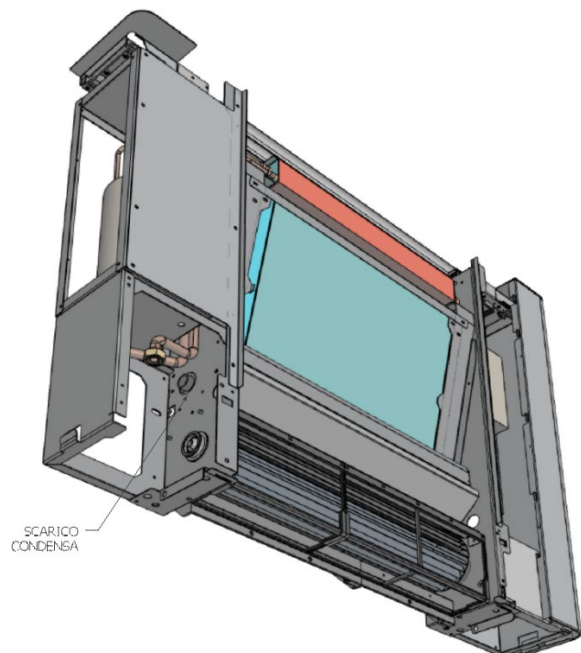
Scarico condensa laterale
