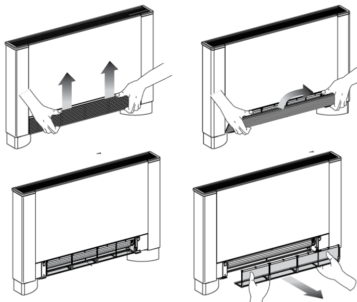
Vista per estrazione filtri
